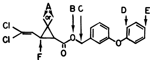
(+) trans -permethrin
