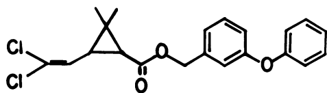
(+) cis -permethrin
