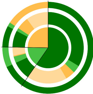
Mycoplasma pneumoniae
