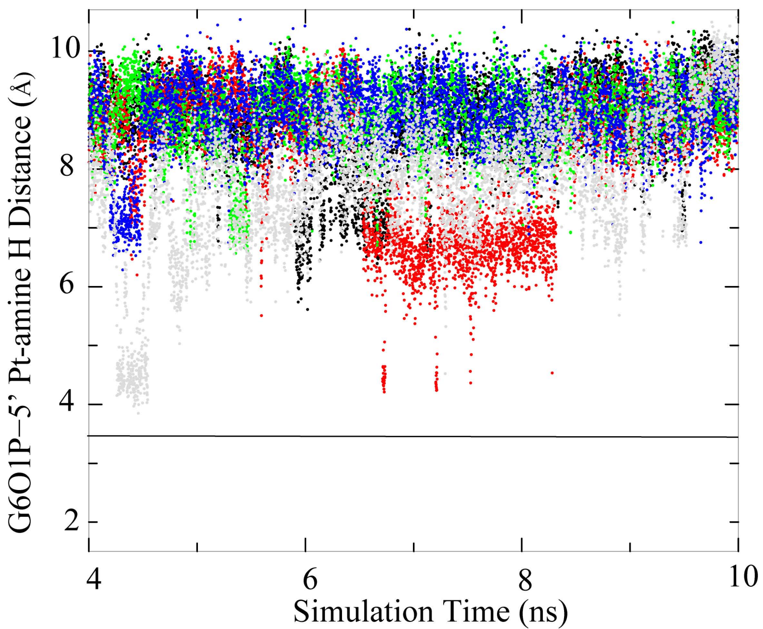
CP-SRY
