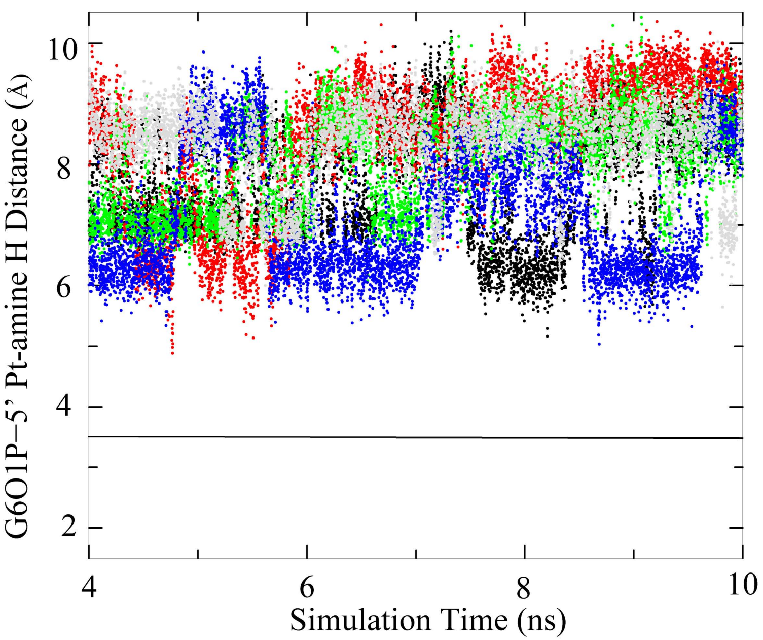
OX-SRY
