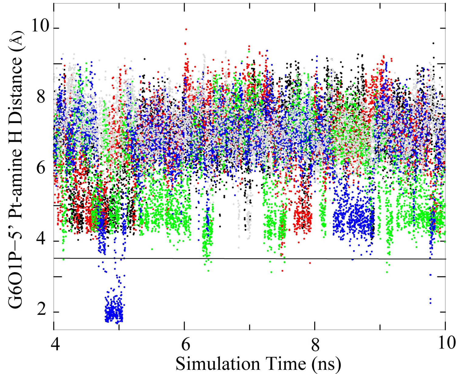
CP-NMR
