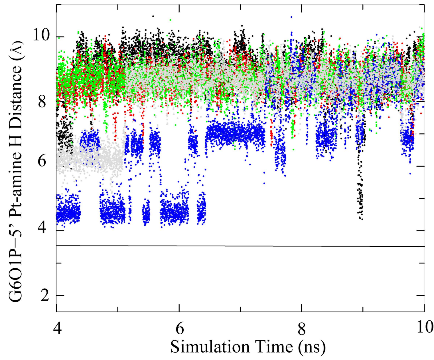
OX-NMR
