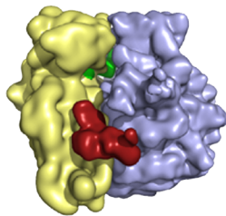
70S·RF3
