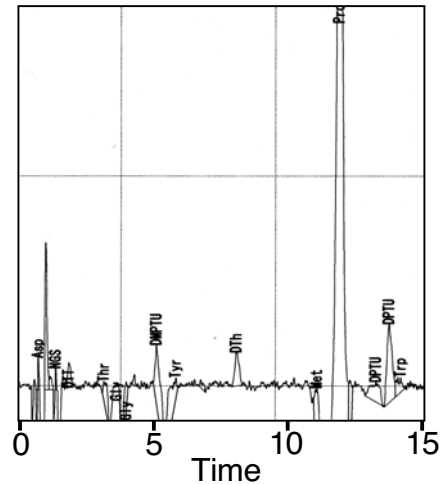
c: Pro32
