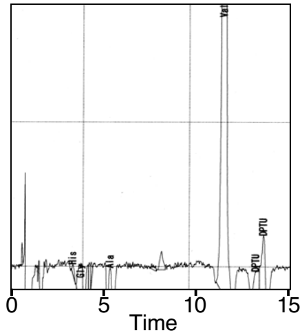
a: Val30
