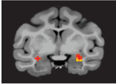
Monkey E
