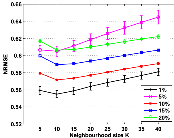
Calcineurin
