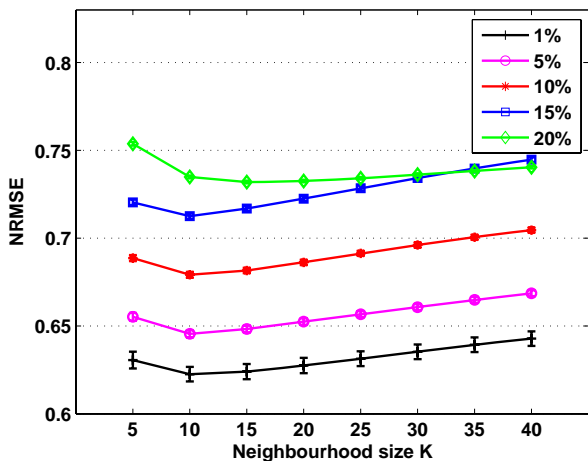
Diauxic
