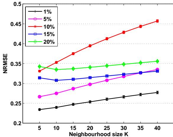
Calcineurin
