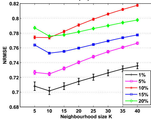
Gasch
