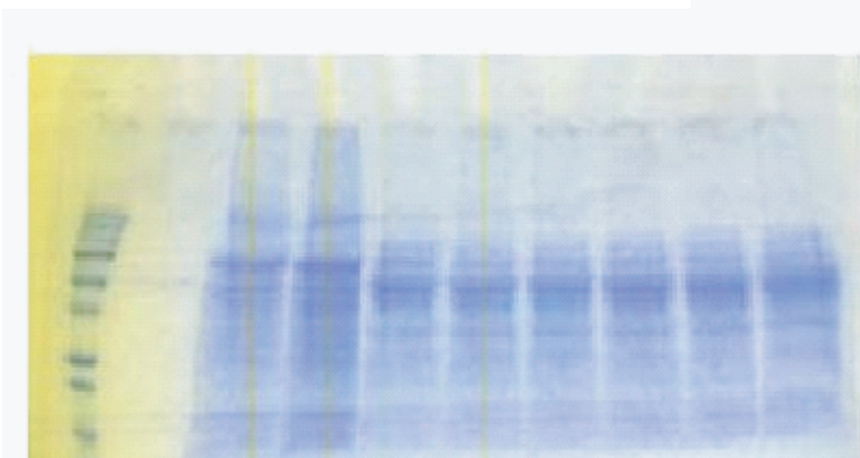
SDS-PAGE gel/dried
