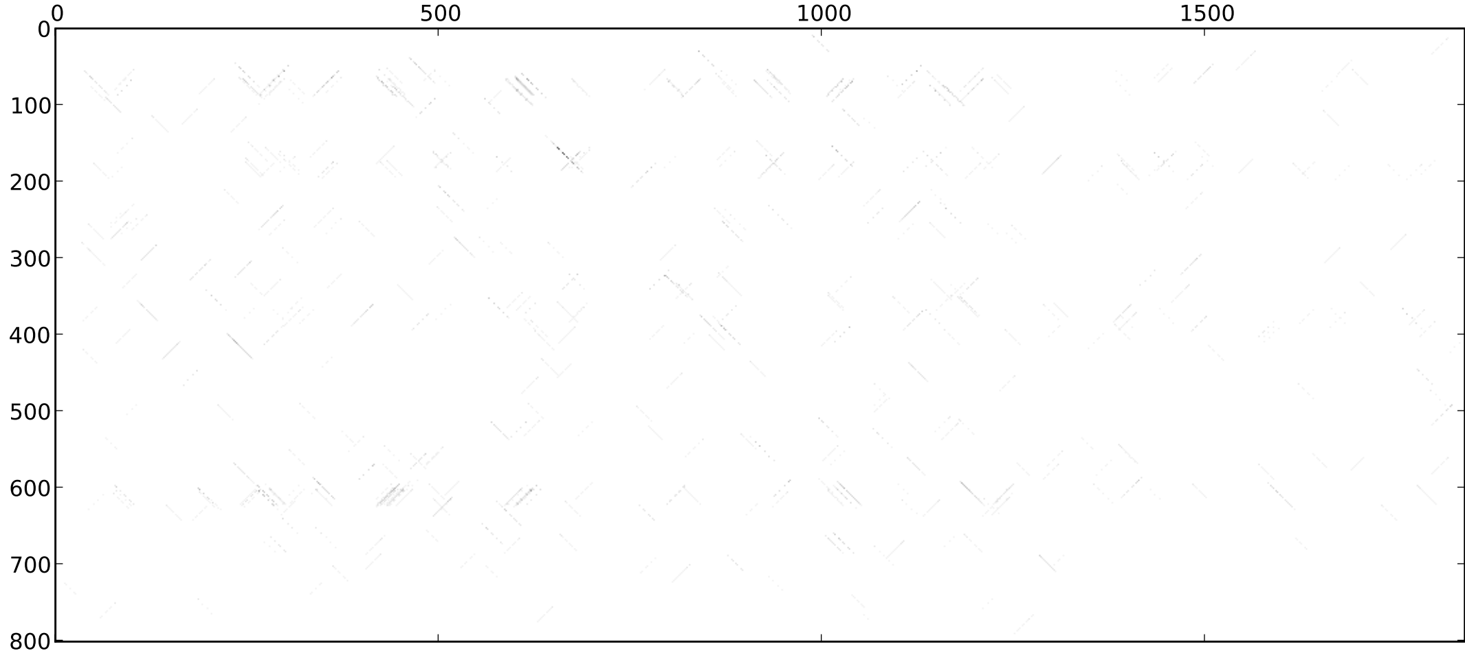
st46_dmel_themira_putris_dotplot_20-0.60_rev_normed_extend
