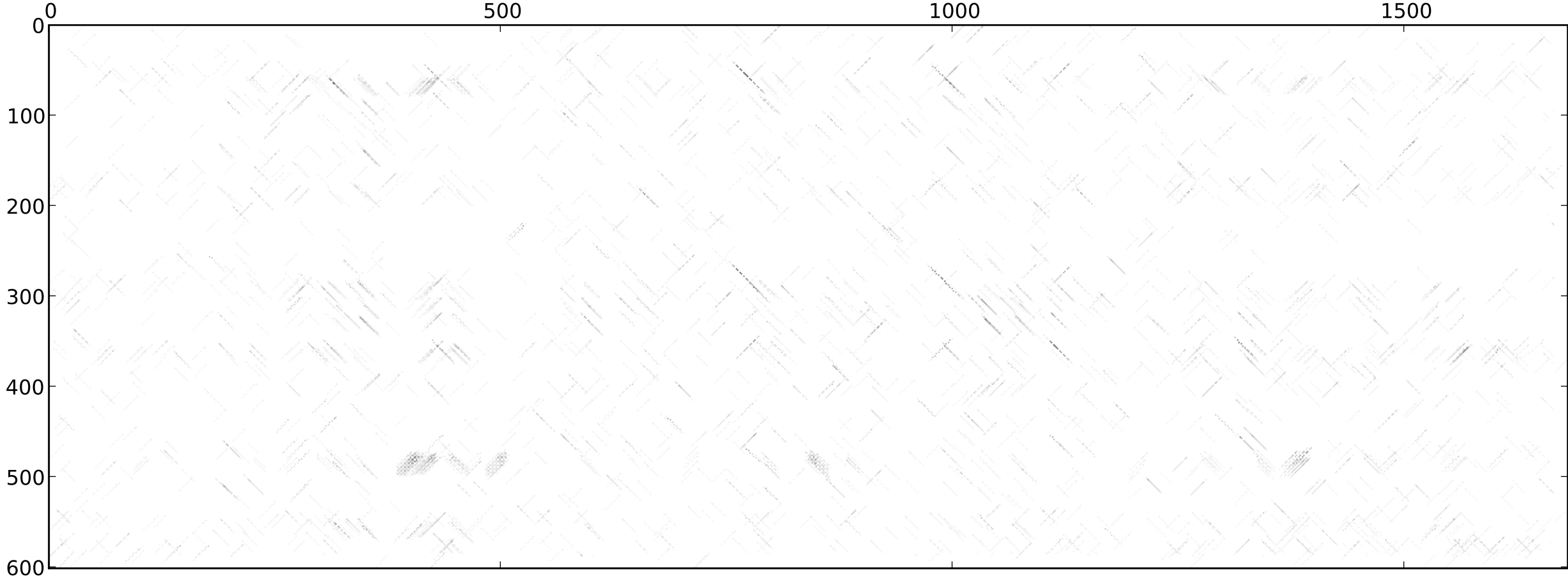
st37_dmel_themira_putris_dotplot_14-0.60_rev_normed_extend
