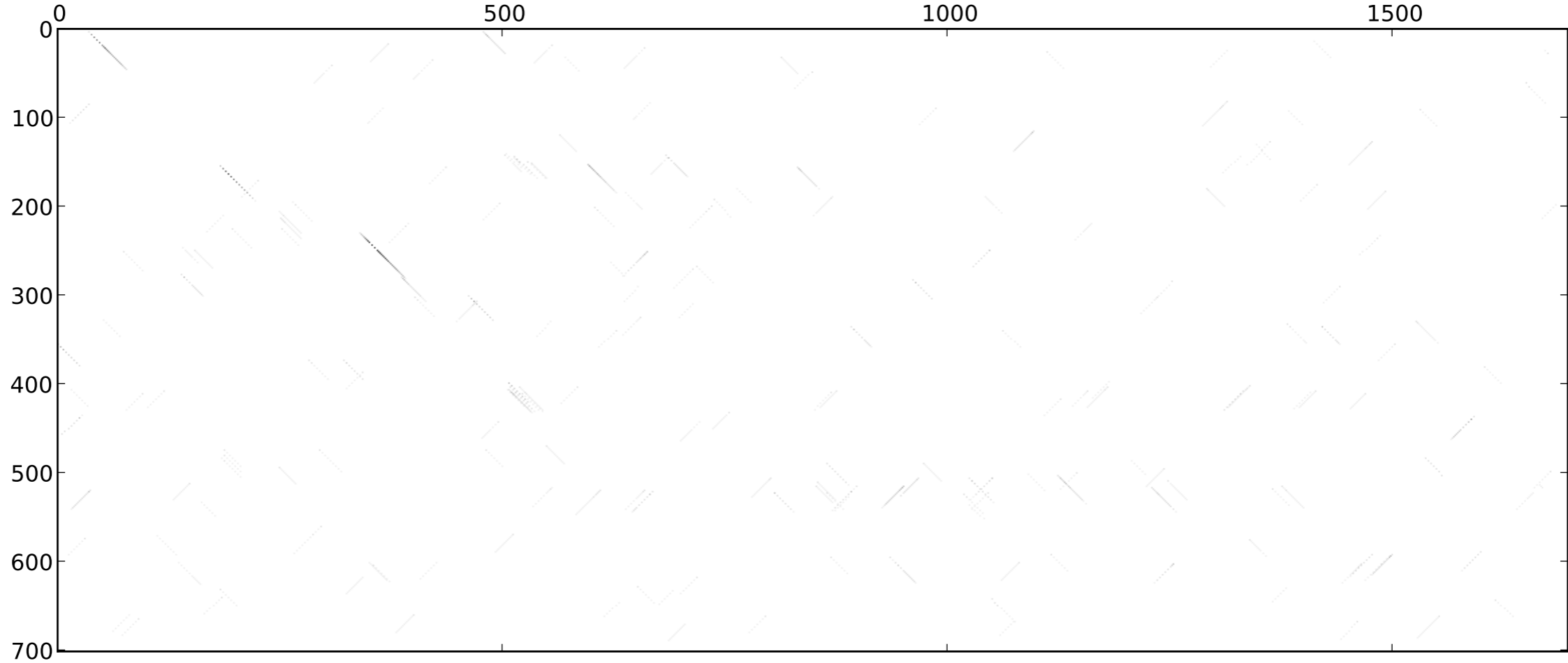
st2_dmel_themira_putris_dotplot_20-0.60_rev_normed_extend
