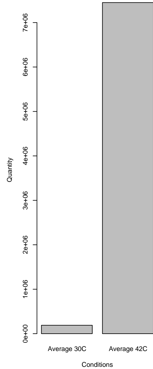
SCO3671 (dnaK)
