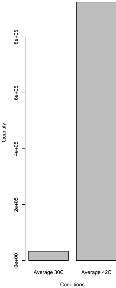
SCO4157
