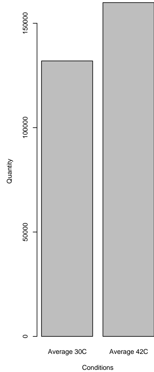
SCO5639
