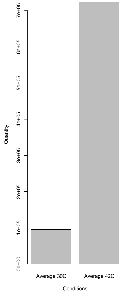
SCO3202
