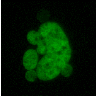
H3K27me3
