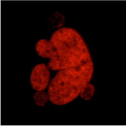
H3K27me2
