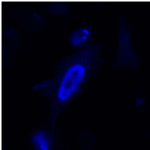
ATF6 \alpha (1-373)
