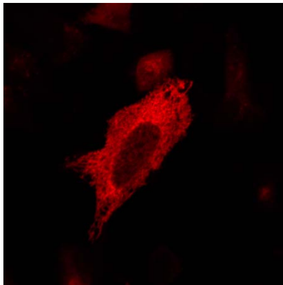
DsRed-ER
