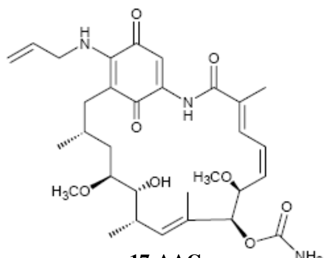
17-AAG
