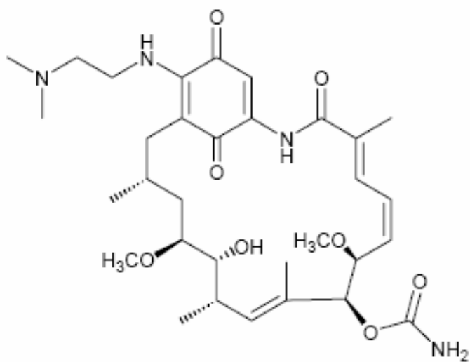
17-DMAG
