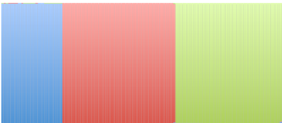
M msp3 , K=3
