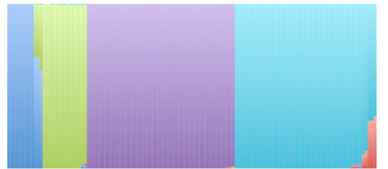
N msp3 , K=5
