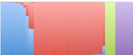
Q glurp , K=4
