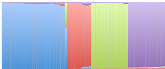
G ama1 , K=5
