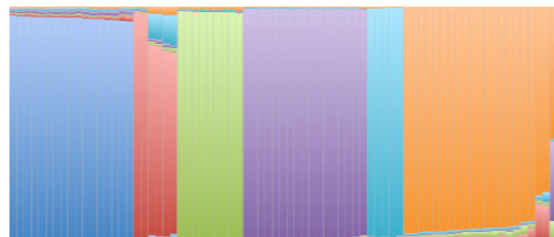
H ama1 , K=7
