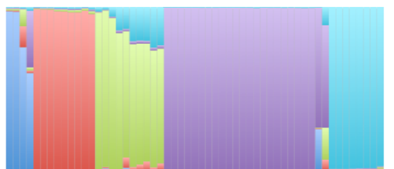
T pfs48/45 , K=5
