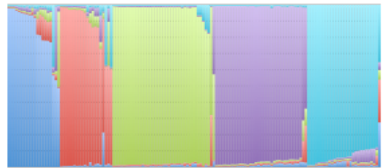
R glurp , K=6
