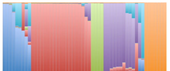
R glurp , K=6
