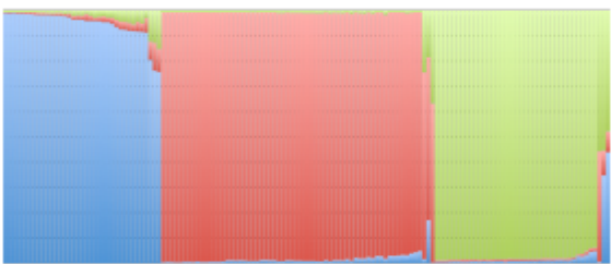
Q glurp , K=4
