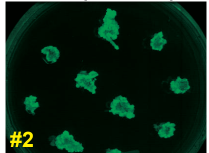
35S( GtCHS )
