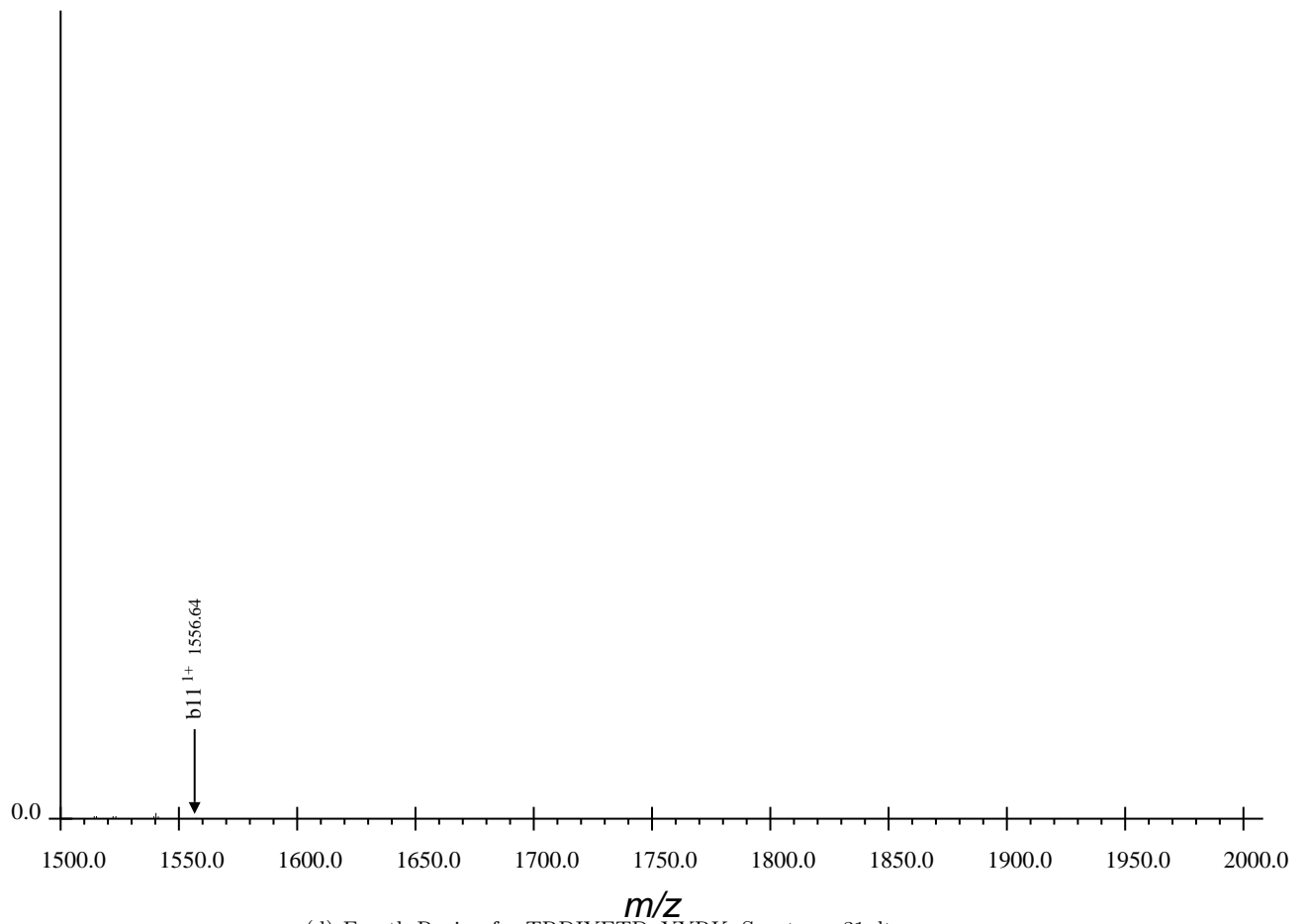
(d) Fourth Region for TRDIYETDpYYRK, Spectrum 31.dta
