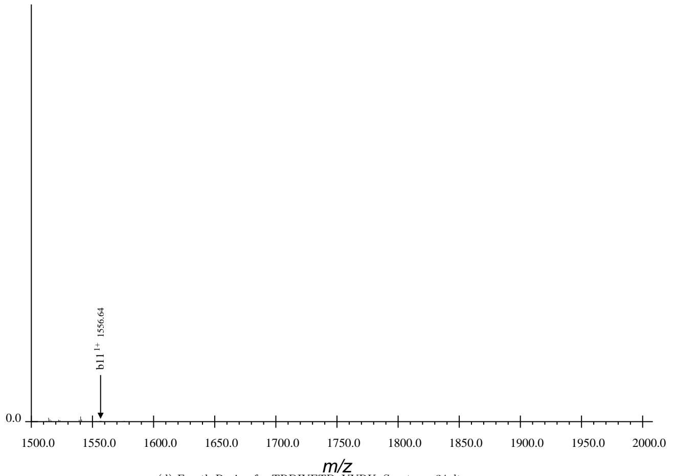
(d) Fourth Region for TRDIYETDpYYRK, Spectrum 34.dta
