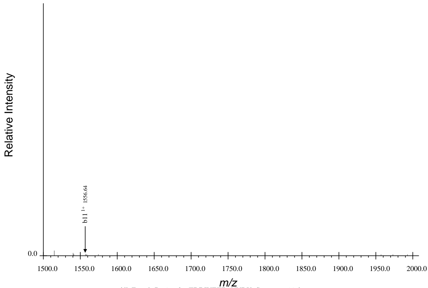
(d) Fourth Region for TRDIYETDpYYRK, Spectrum 36.dta
