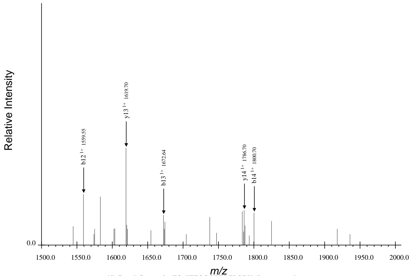
(d) Fourth Region for FQpSEEQQQTEDELQDK, Spectrum 7.dta
