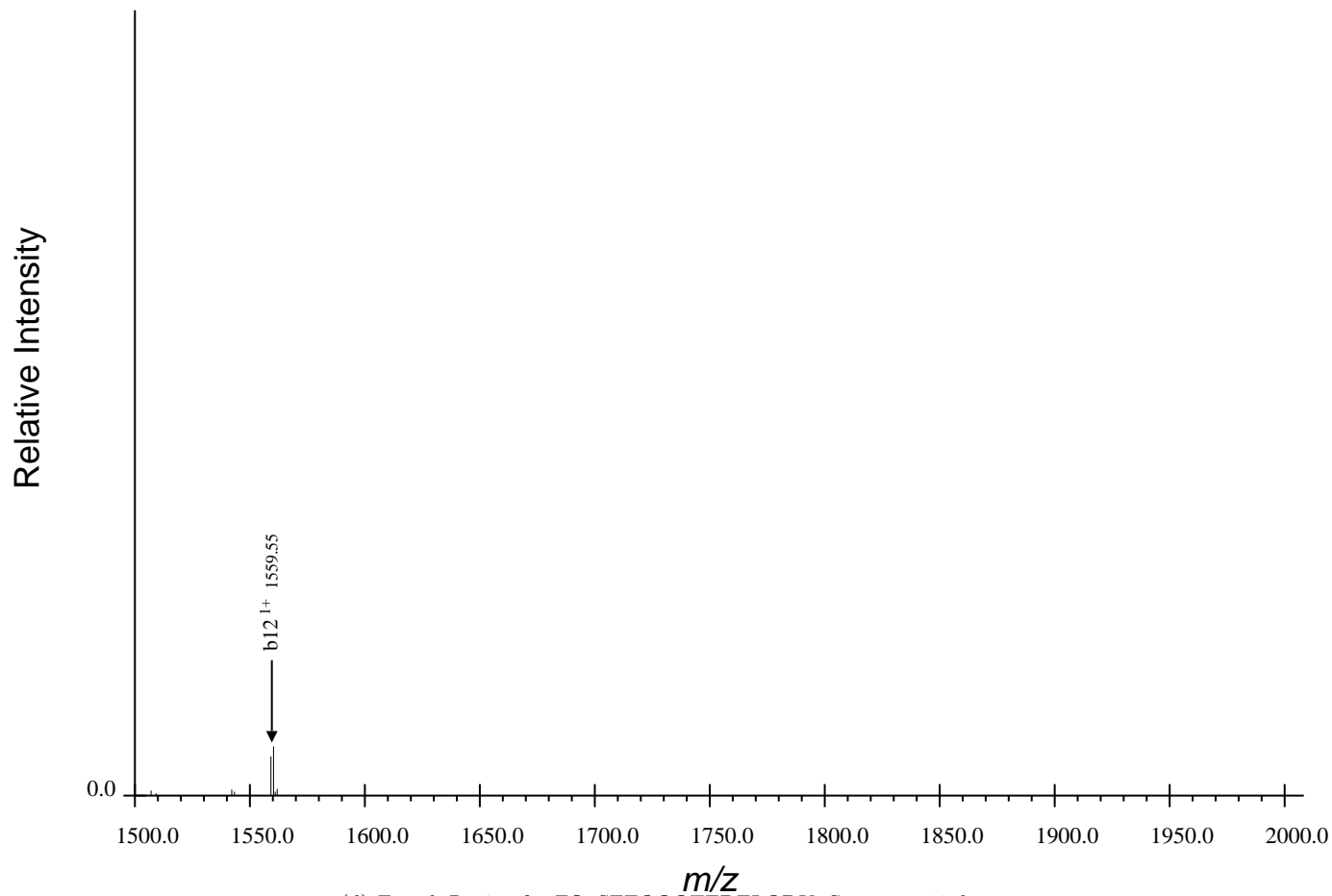
(d) Fourth Region for FQpSEEQQQTEDELQDK, Spectrum 13.dta
