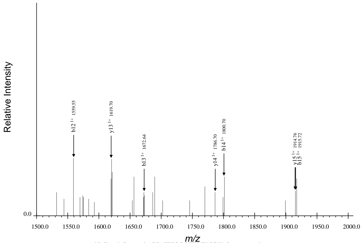
(d) Fourth Region for FQpSEEQQQTEDELQDK, Spectrum 6.dta
