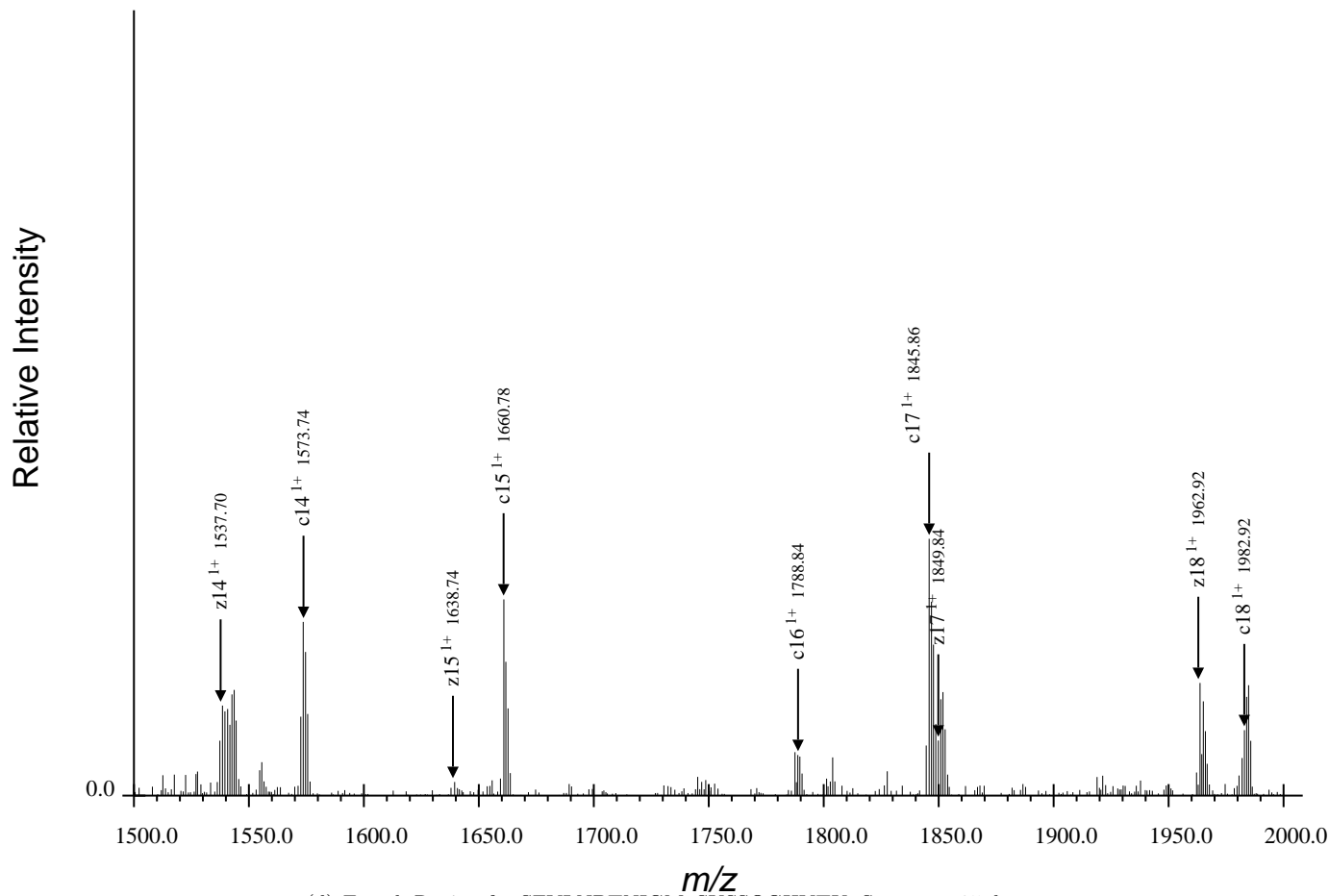
(d) Fourth Region for SFVLNPTNIGMpSKSSQGHVTK, Spectrum 25.dta
