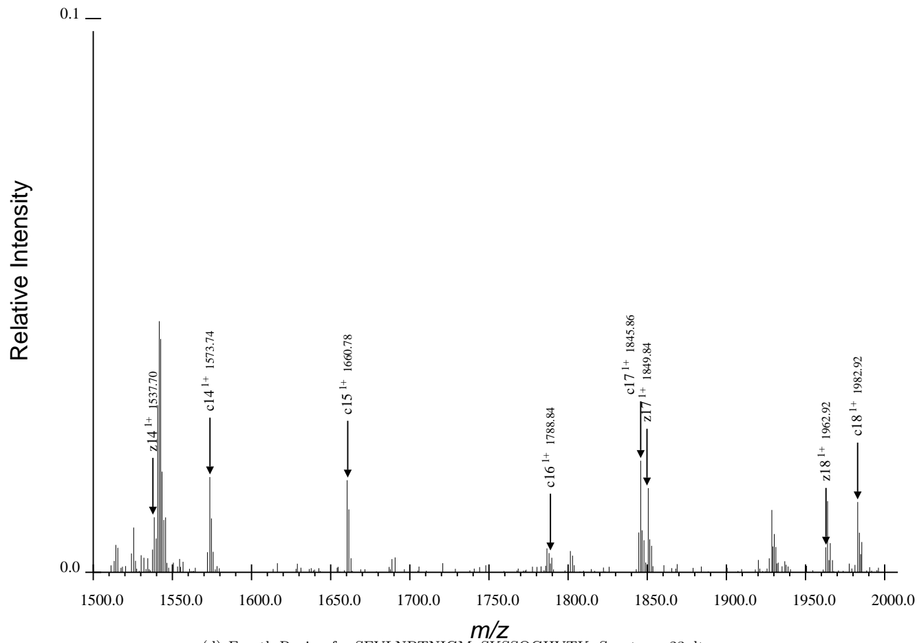
(d) Fourth Region for SFVLNPTNIGMpSKSSQGHVTK, Spectrum 23.dta
