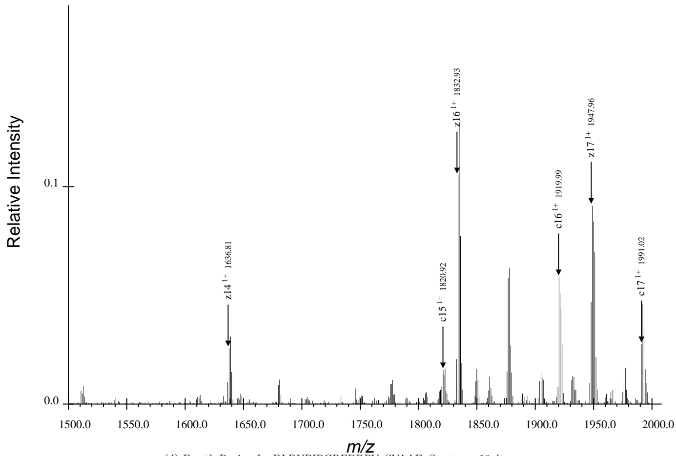
(d) Fourth Region for DLDVPIPGRFDRRVpSVA AE, Spectrum 18.dta
