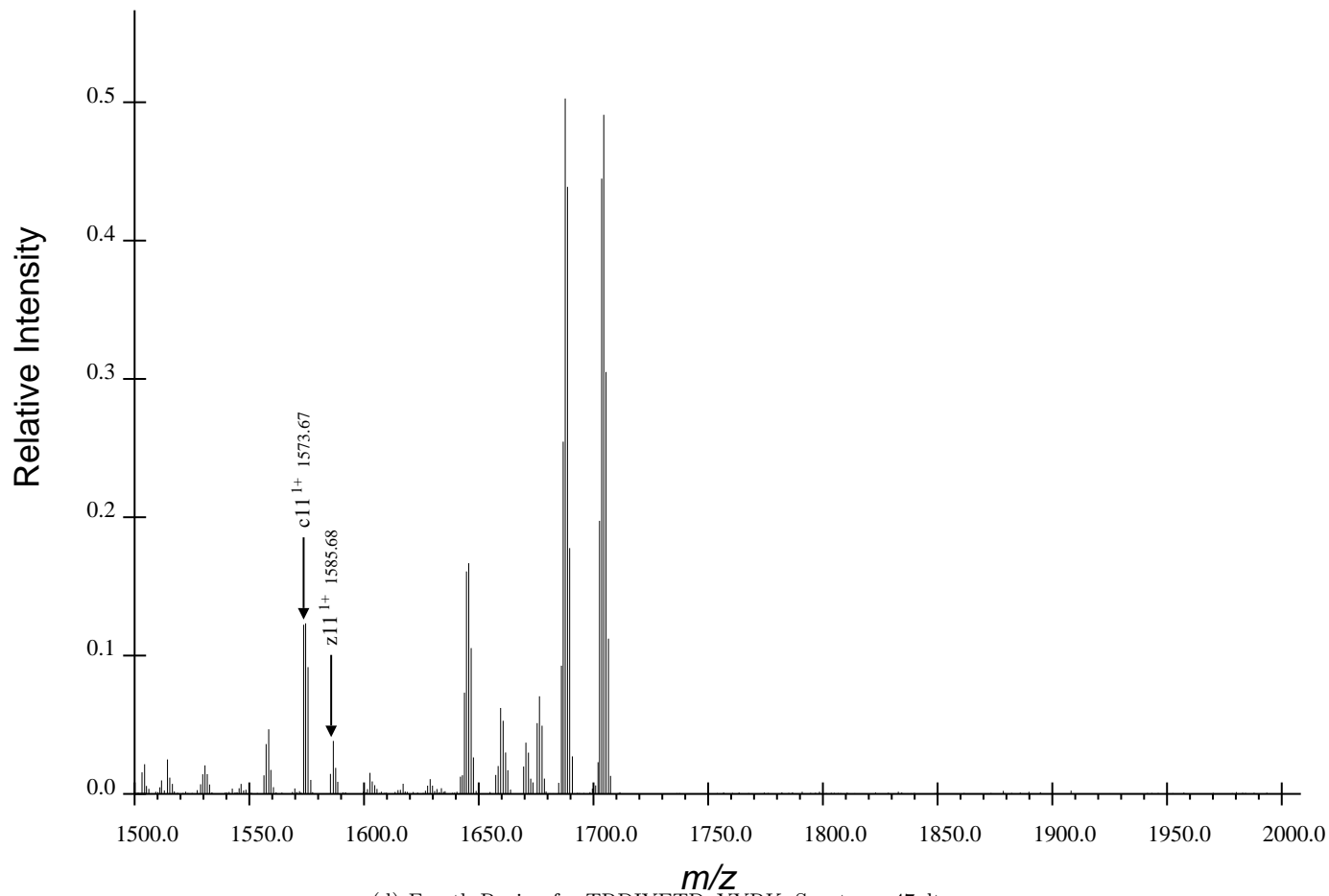
(d) Fourth Region for TRDIYETDpYYRK, Spectrum 47.dta
