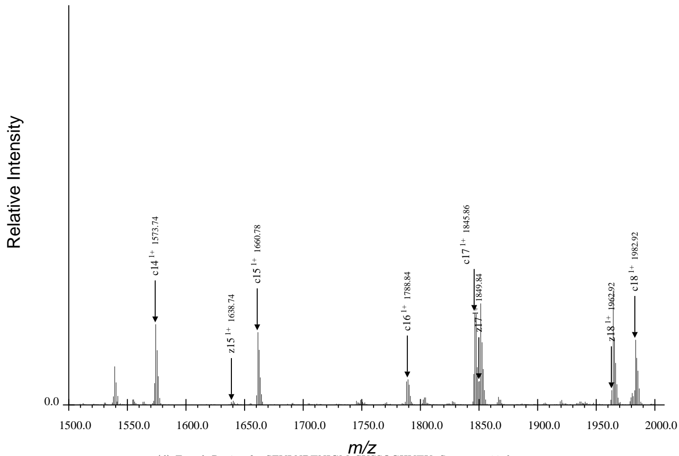
(d) Fourth Region for SFVLNPTNIGMpSKSSQGHVTK, Spectrum 22.dta
