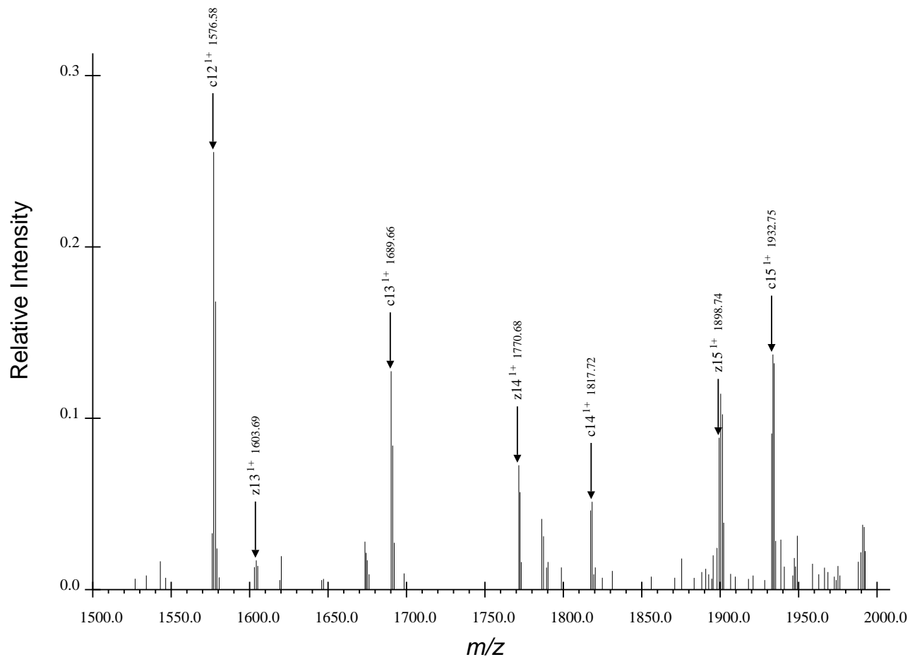
(d) Fourth Region for FQpSEEQQQTEDELQDK, Spectrum 16.dta
