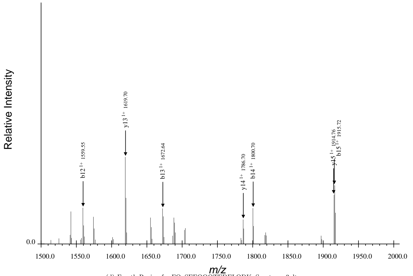
(d) Fourth Region for FQpSEEQQQTEDELQDK, Spectrum 3.dta
