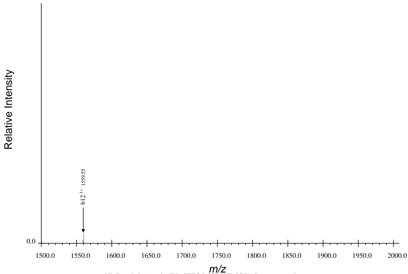
(d) Fourth Region for FQpSEEQQQTEDELQDK, Spectrum 14.dta
