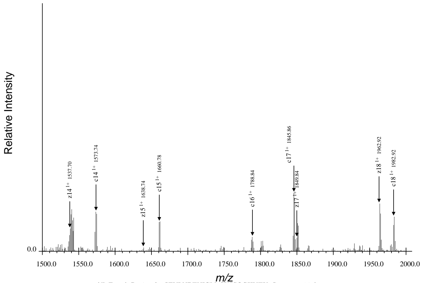
(d) Fourth Region for SFVLNPTNIGMpSKSSQGHVTK, Spectrum 26.dta
