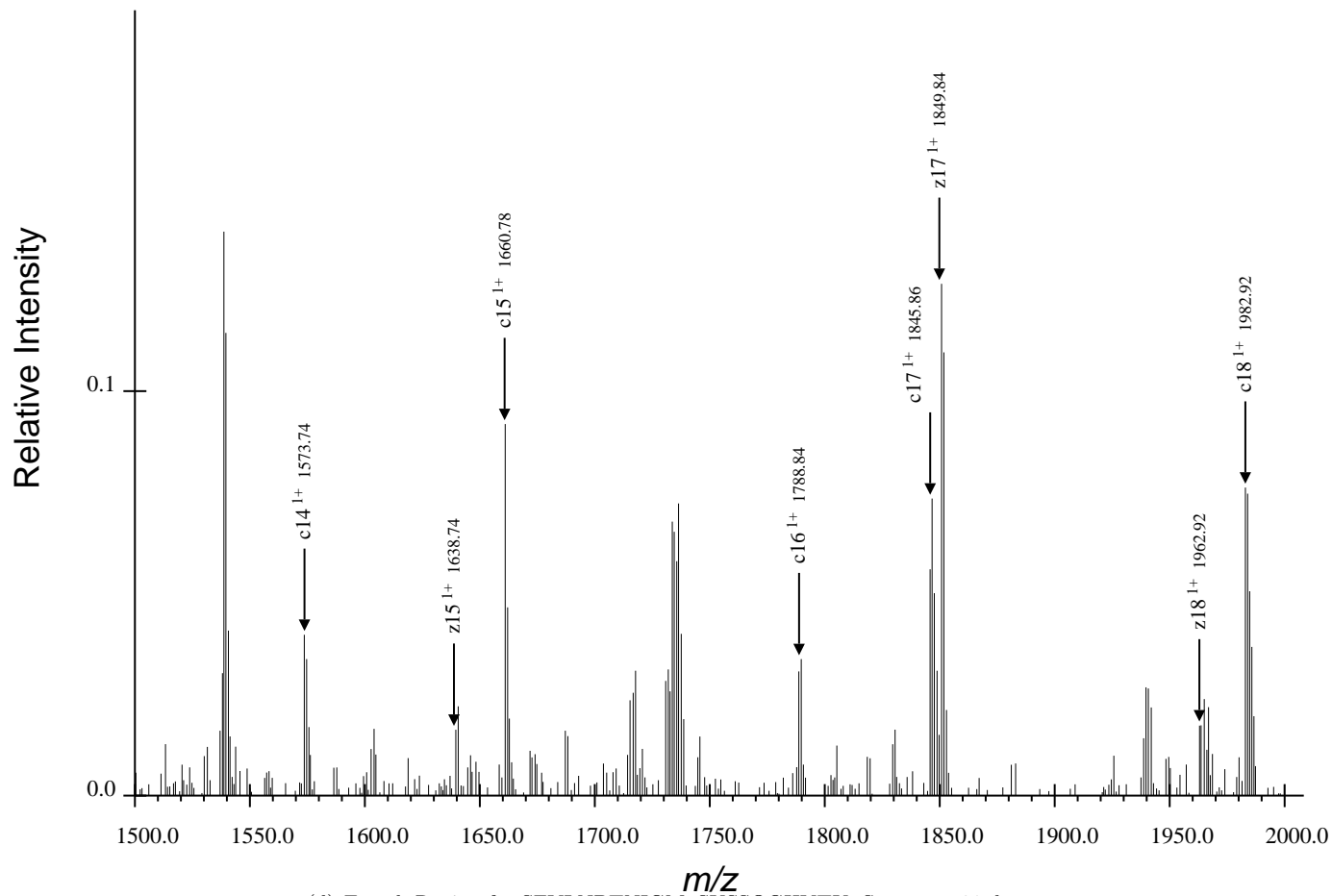
(d) Fourth Region for SFVLNPTNIGMpSKSSQGHVTK, Spectrum 28.dta
