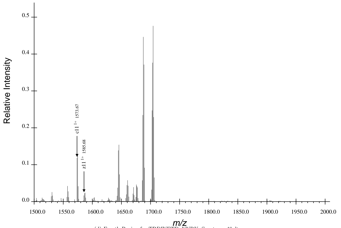
(d) Fourth Region for TRDIYETDpYYRK, Spectrum 46.dta
