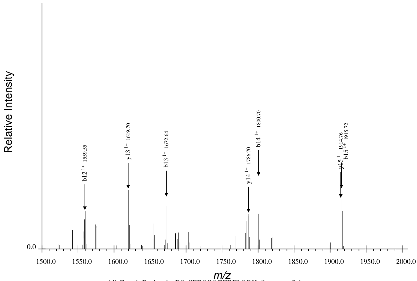
(d) Fourth Region for FQpSEEQQQTEDELQDK, Spectrum 5.dta
