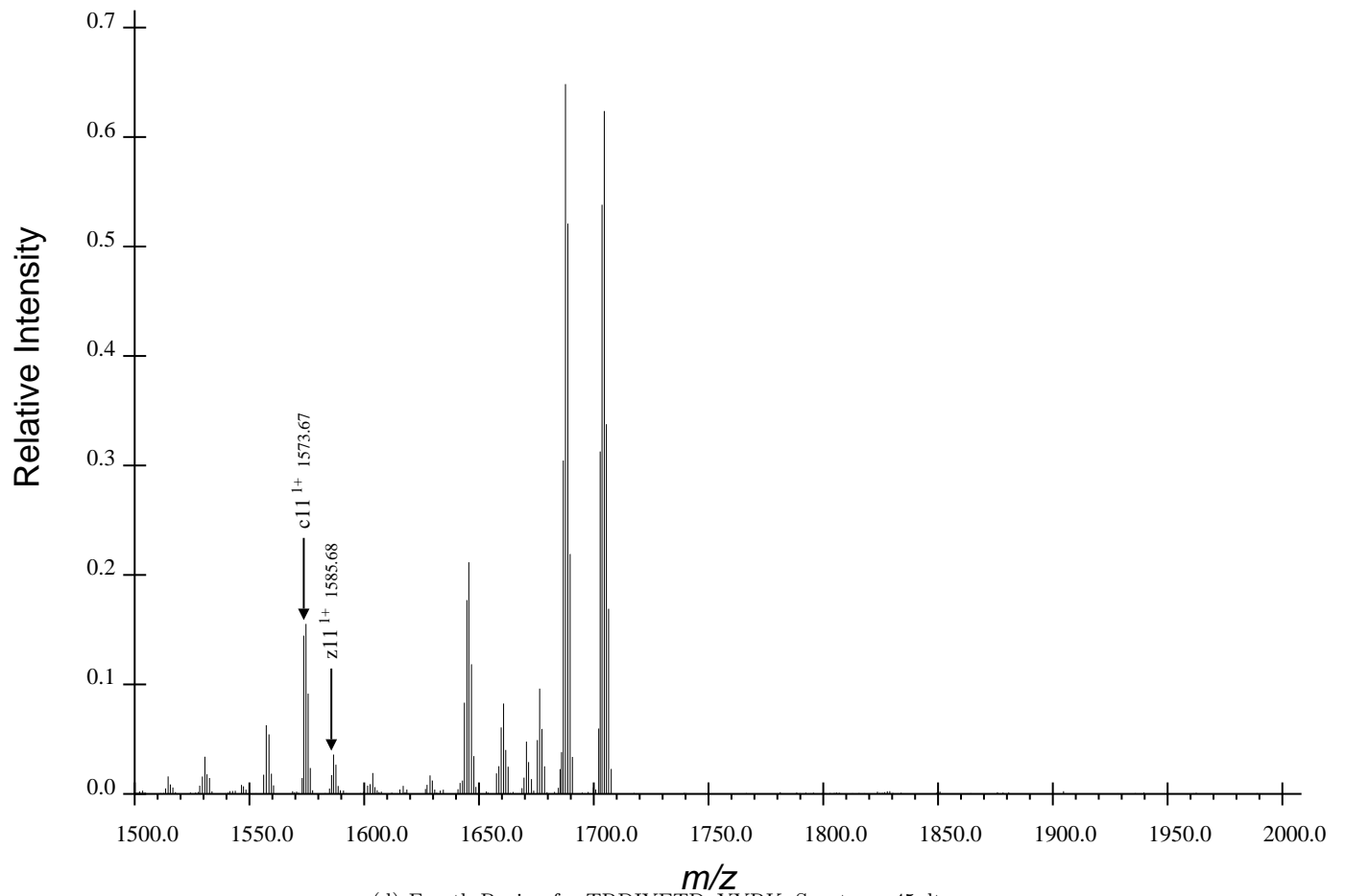
(d) Fourth Region for TRDIYETDpYYRK, Spectrum 45.dta
