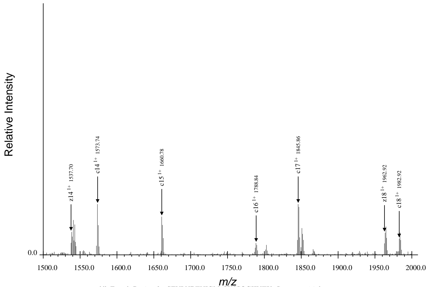
(d) Fourth Region for SFVLNPTNIGMpSKSSQGHVTK, Spectrum 24.dta
