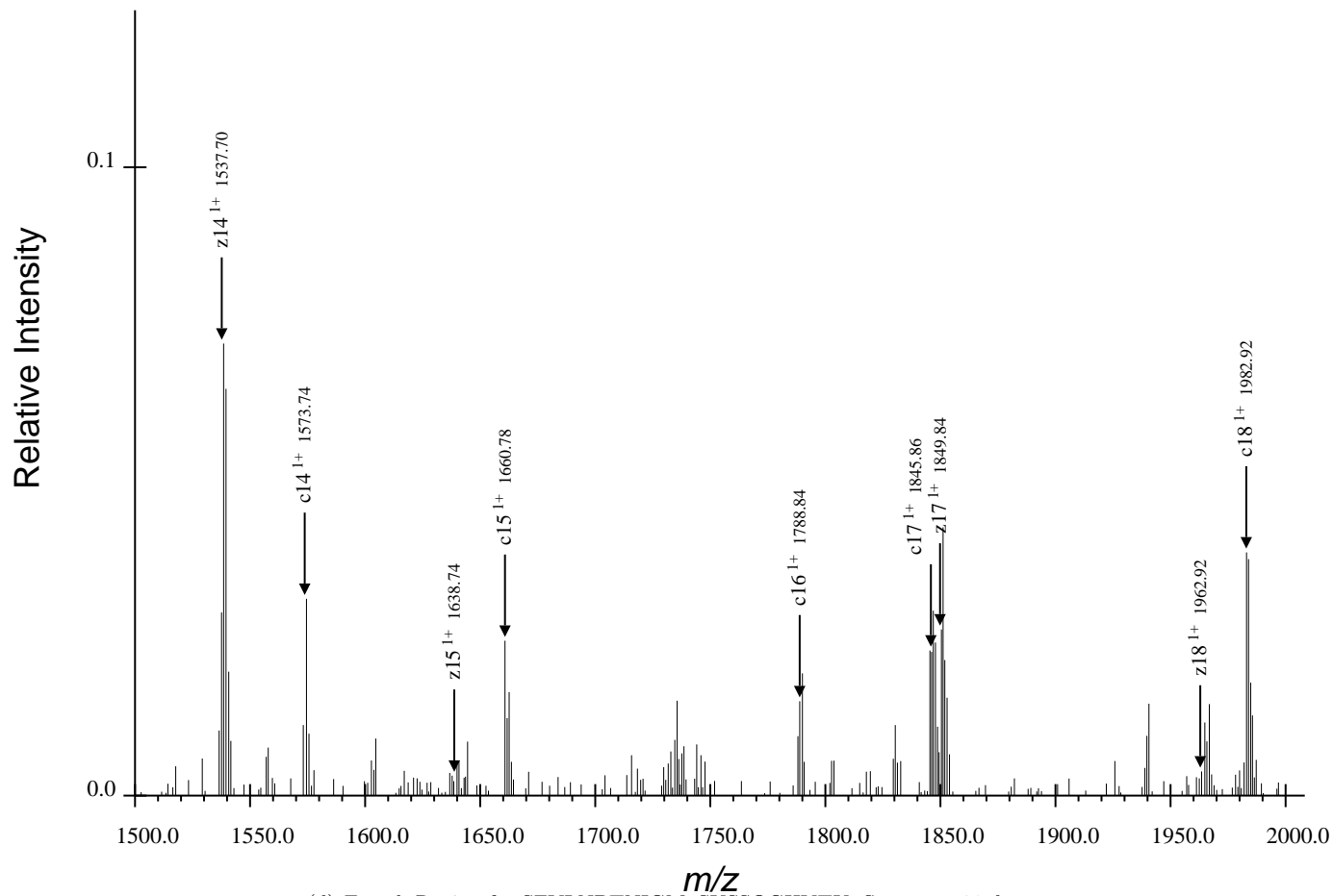
(d) Fourth Region for SFVLNPTNIGMpSKSSQGHVTK, Spectrum 29.dta
