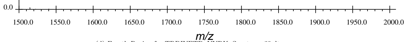
(d) Fourth Region for TRDIYETDpYYRK, Spectrum 30.dta
