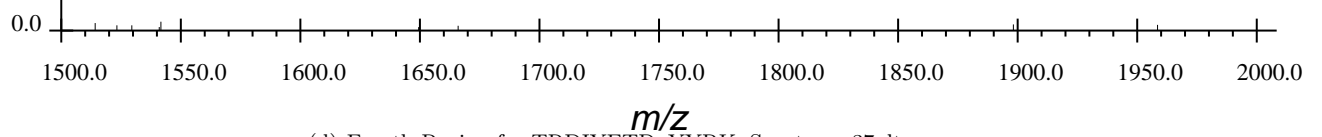
(d) Fourth Region for TRDIYETDpYYRK, Spectrum 37.dta
