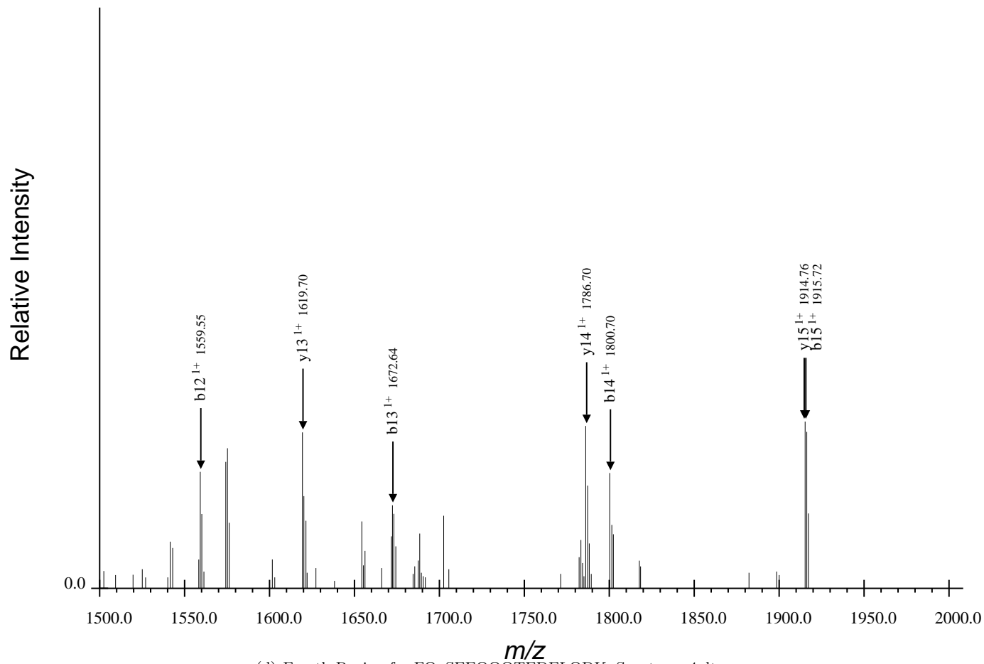
(d) Fourth Region for FQpSEEQQQTEDELQDK, Spectrum 4.dta
