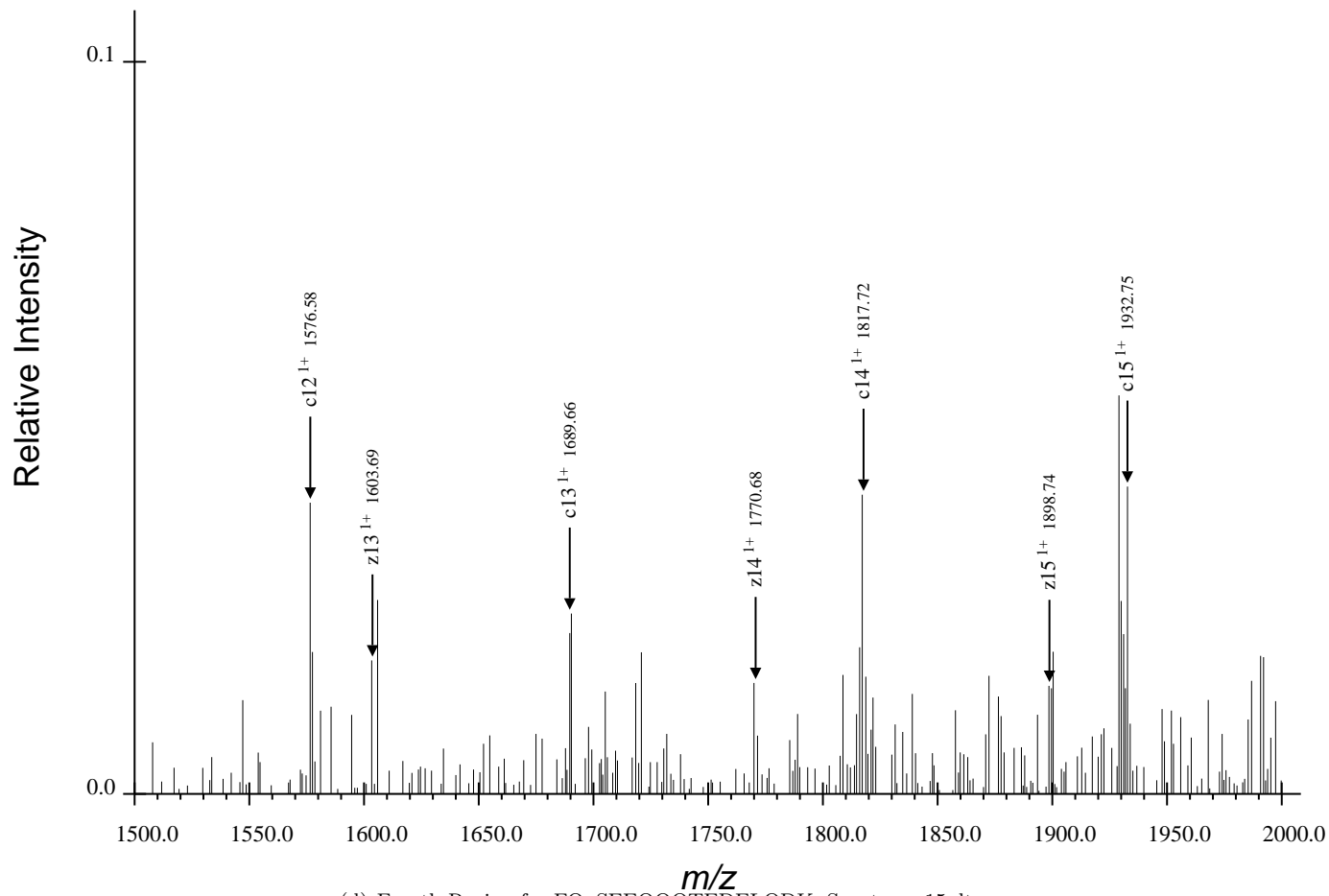
(d) Fourth Region for FQpSEEQQQTEDELQDK, Spectrum 15.dta
