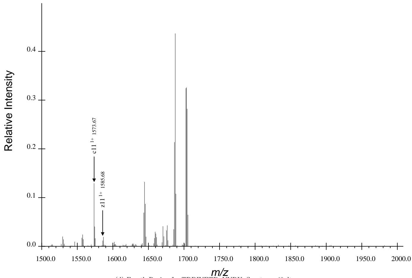
(d) Fourth Region for TRDIYETDpYYRK, Spectrum 48.dta
