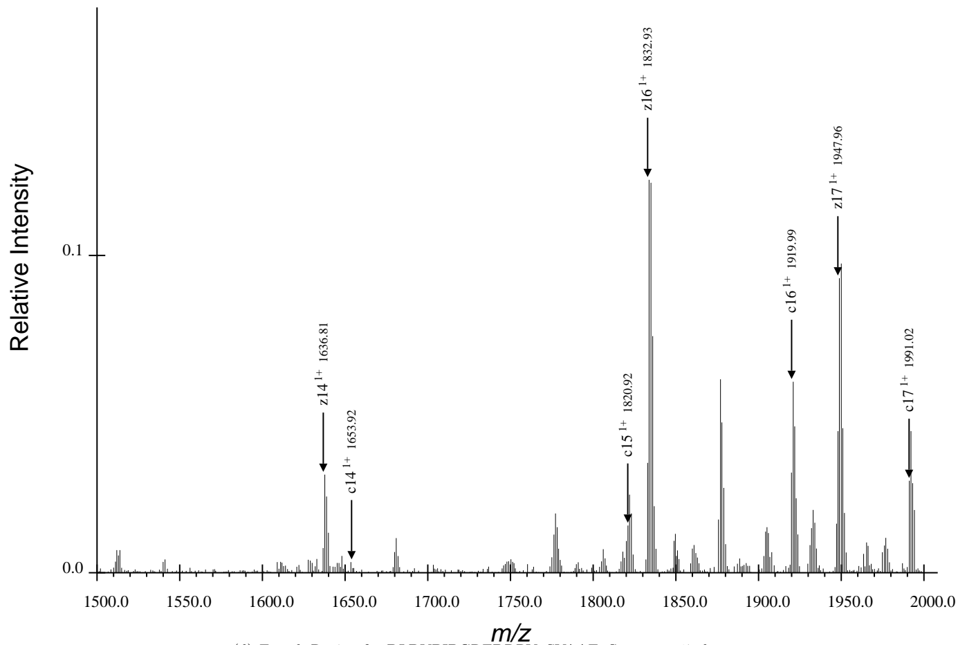
(d) Fourth Region for DLDVPIPGRFDRRVpSVAEE, Spectrum 17.dta
