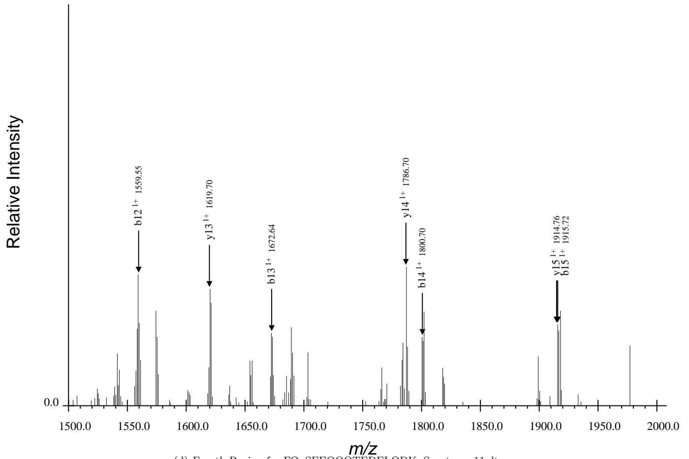
(d) Fourth Region for FQpSEEQQQTEDELQDK, Spectrum 11.dta
