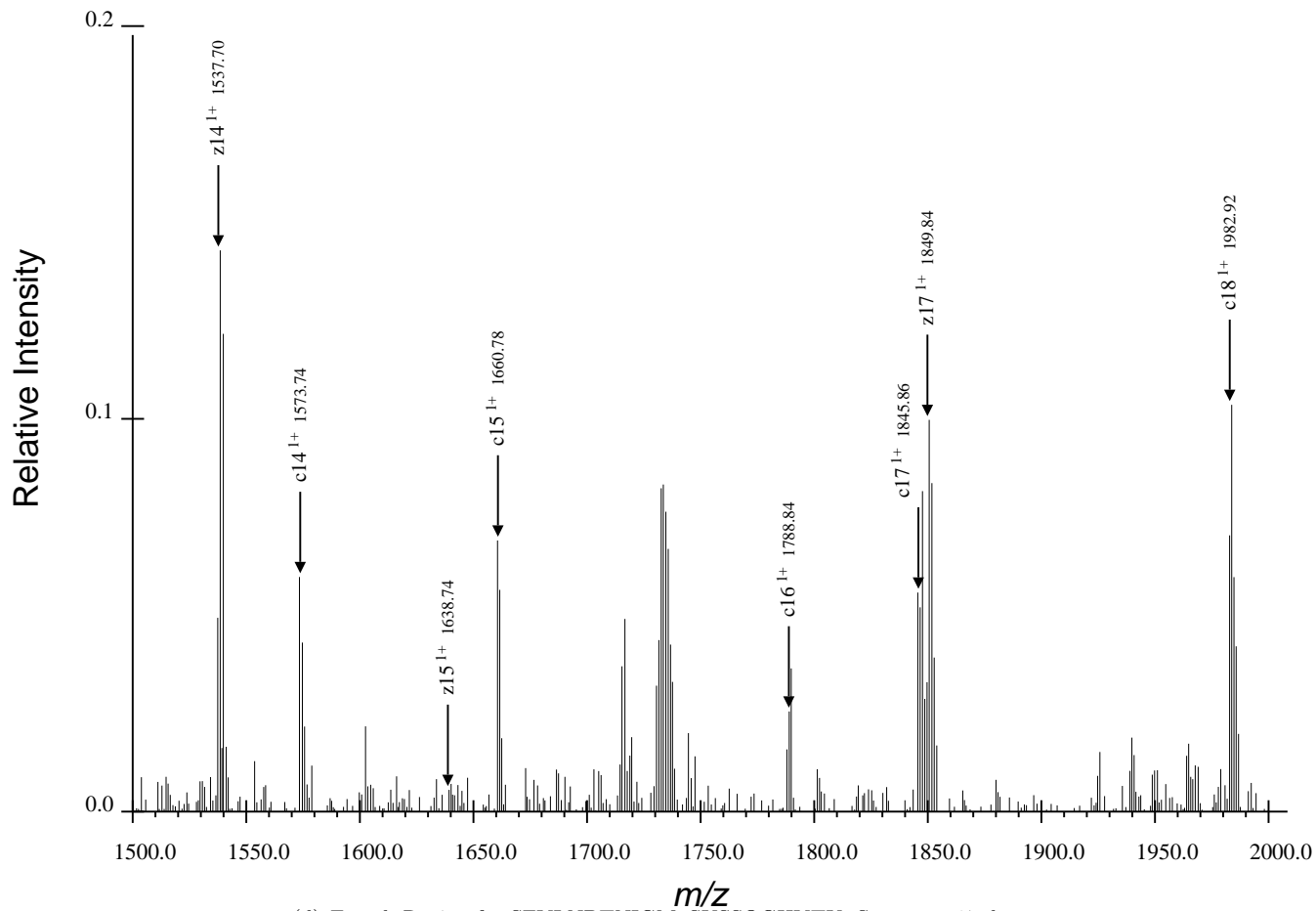
(d) Fourth Region for SFVLNPTNIGMpSKSSQGHVTK, Spectrum 27.dta
