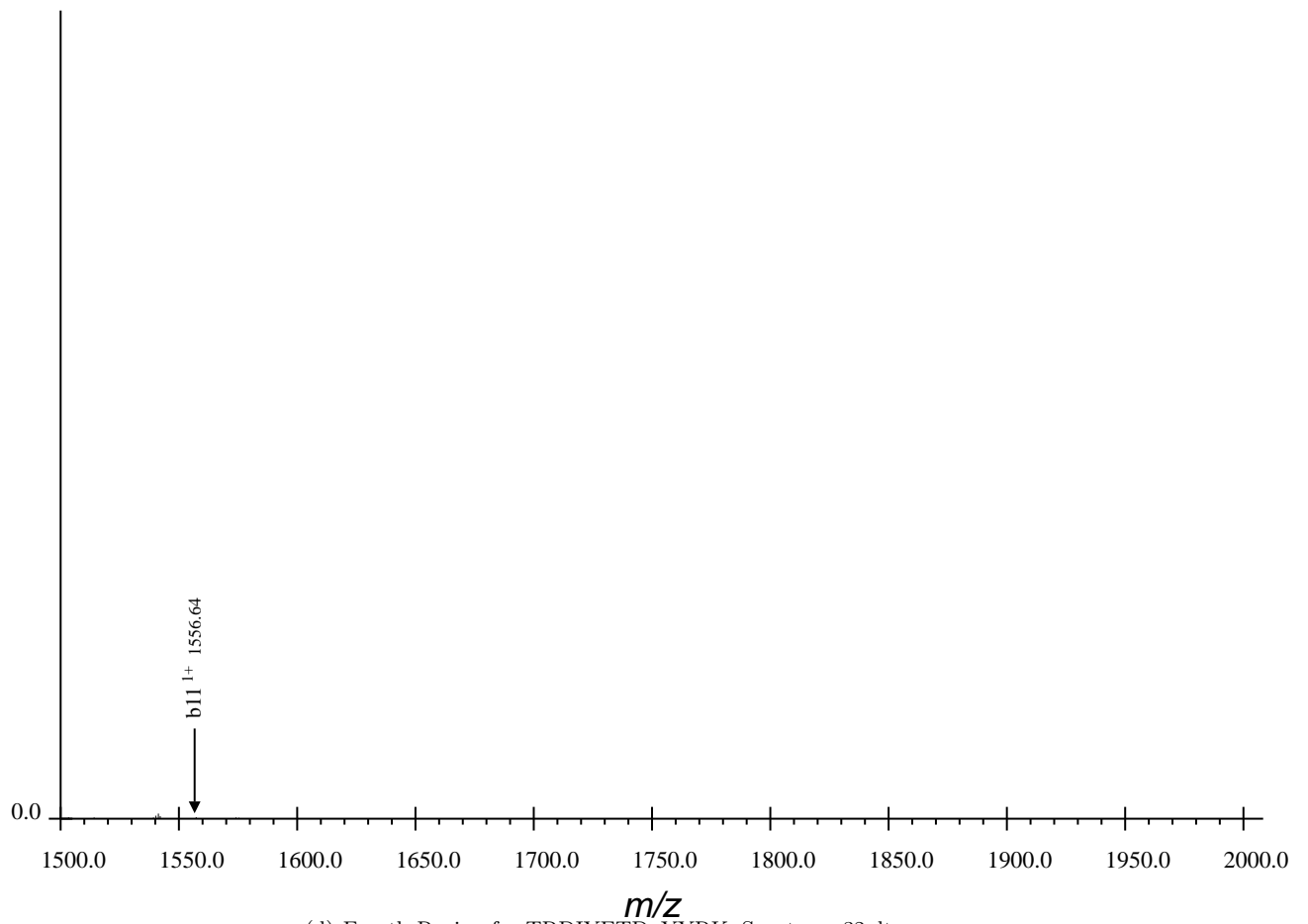
(d) Fourth Region for TRDIYETDpYYRK, Spectrum 32.dta
