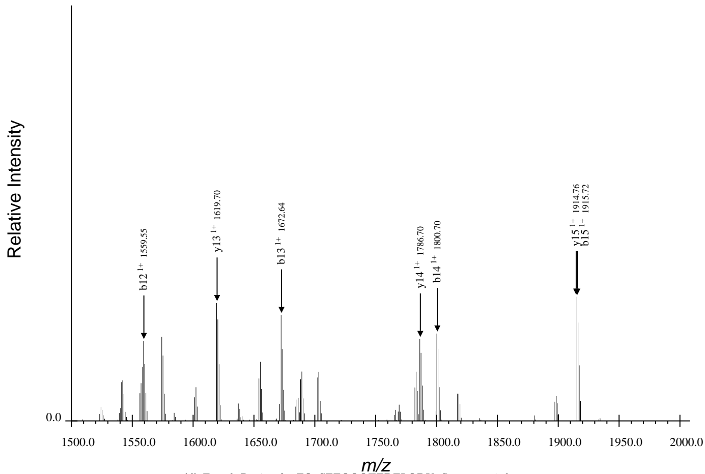
(d) Fourth Region for FQpSEEQQQTEDELQDK, Spectrum 2.dta
