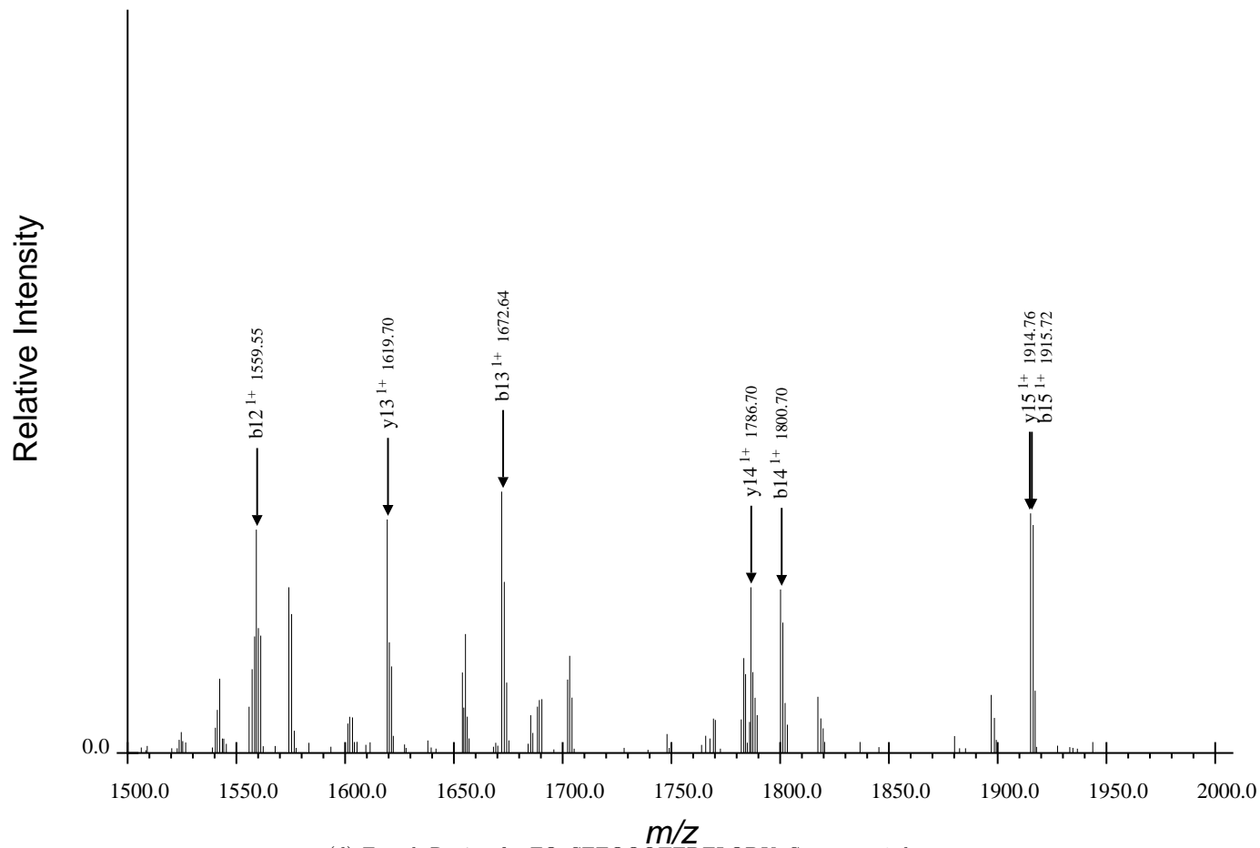
(d) Fourth Region for FQpSEEQQQTEDELQDK, Spectrum 9.dta
