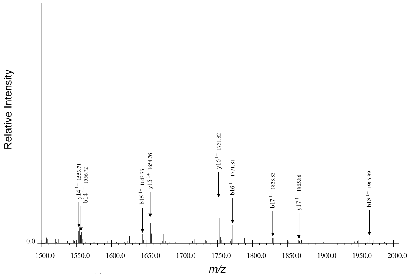
(d) Fourth Region for SFVLNPTNIGMpSKSSQGHVTK, Spectrum 20.dta
