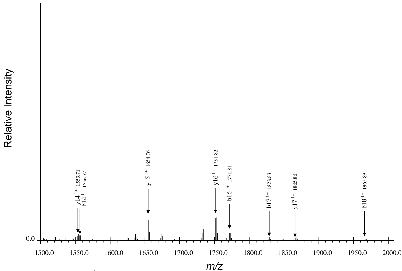
(d) Fourth Region for SFVLNPTNIGMpSKSSQGHVTK, Spectrum 19.dta
