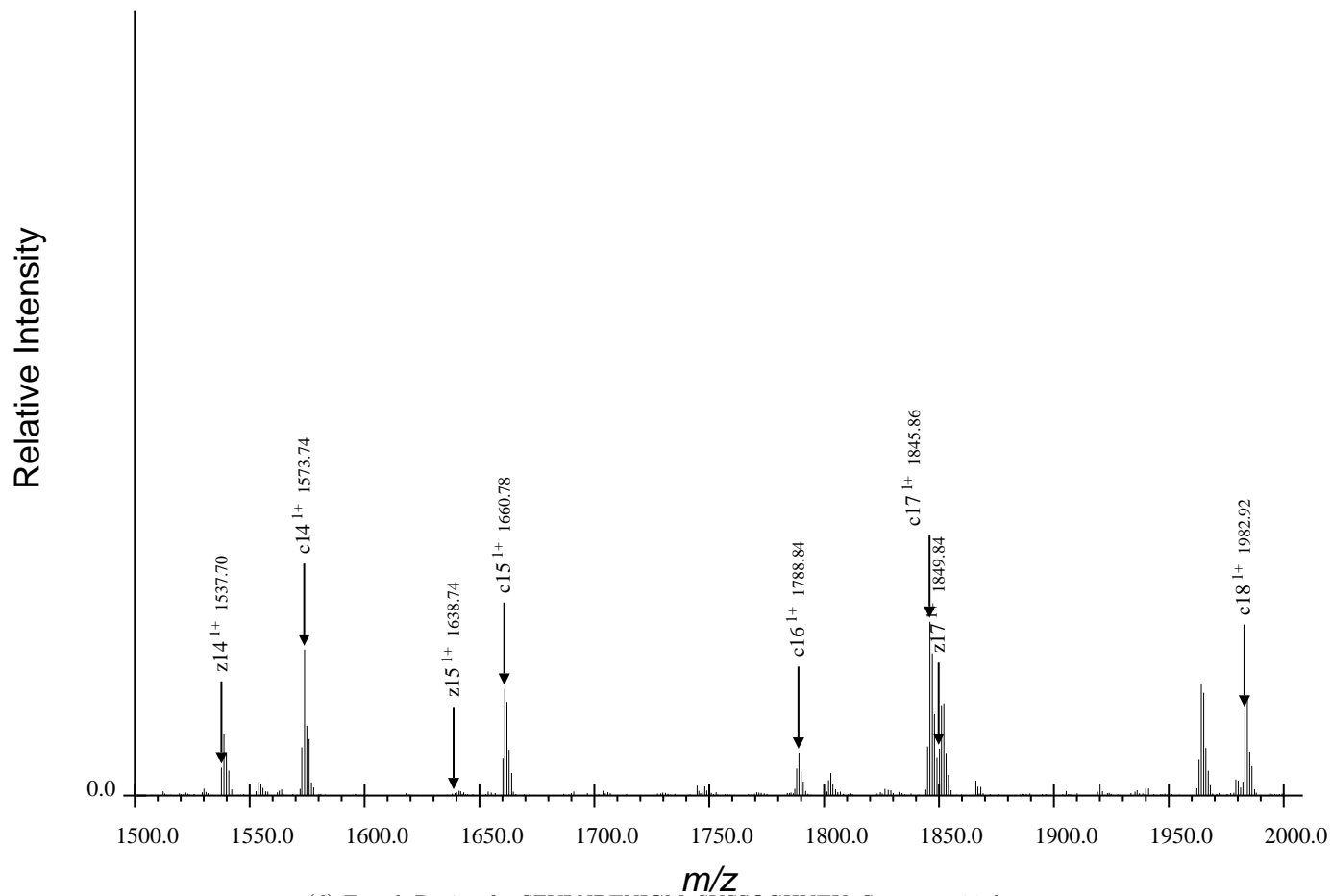
(d) Fourth Region for SFVLNPTNIGMpSKSSQGHVTK, Spectrum 21.dta
