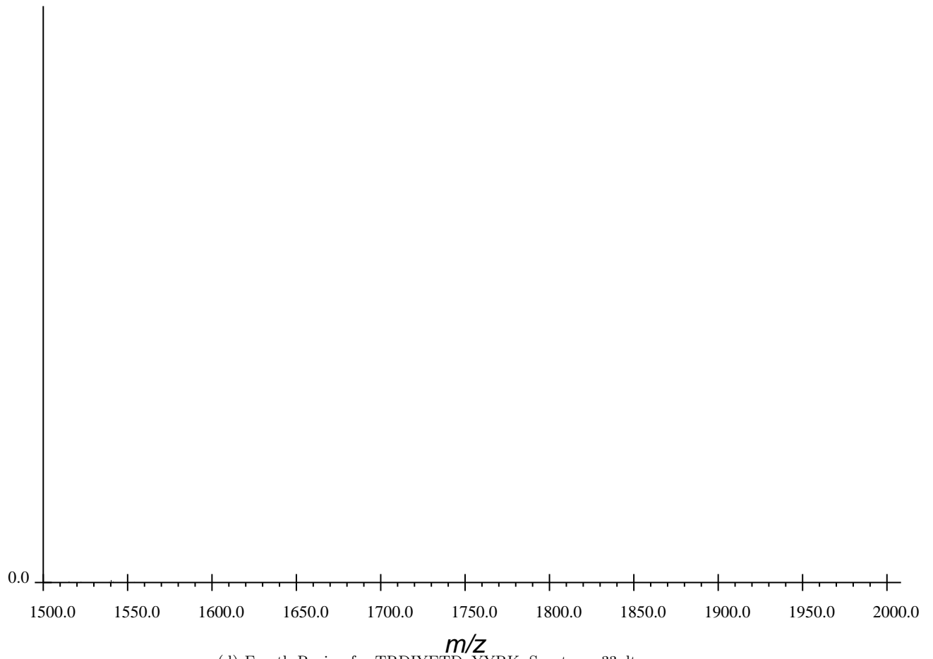
(d) Fourth Region for TRDIYETDpYYRK, Spectrum 33.dta
