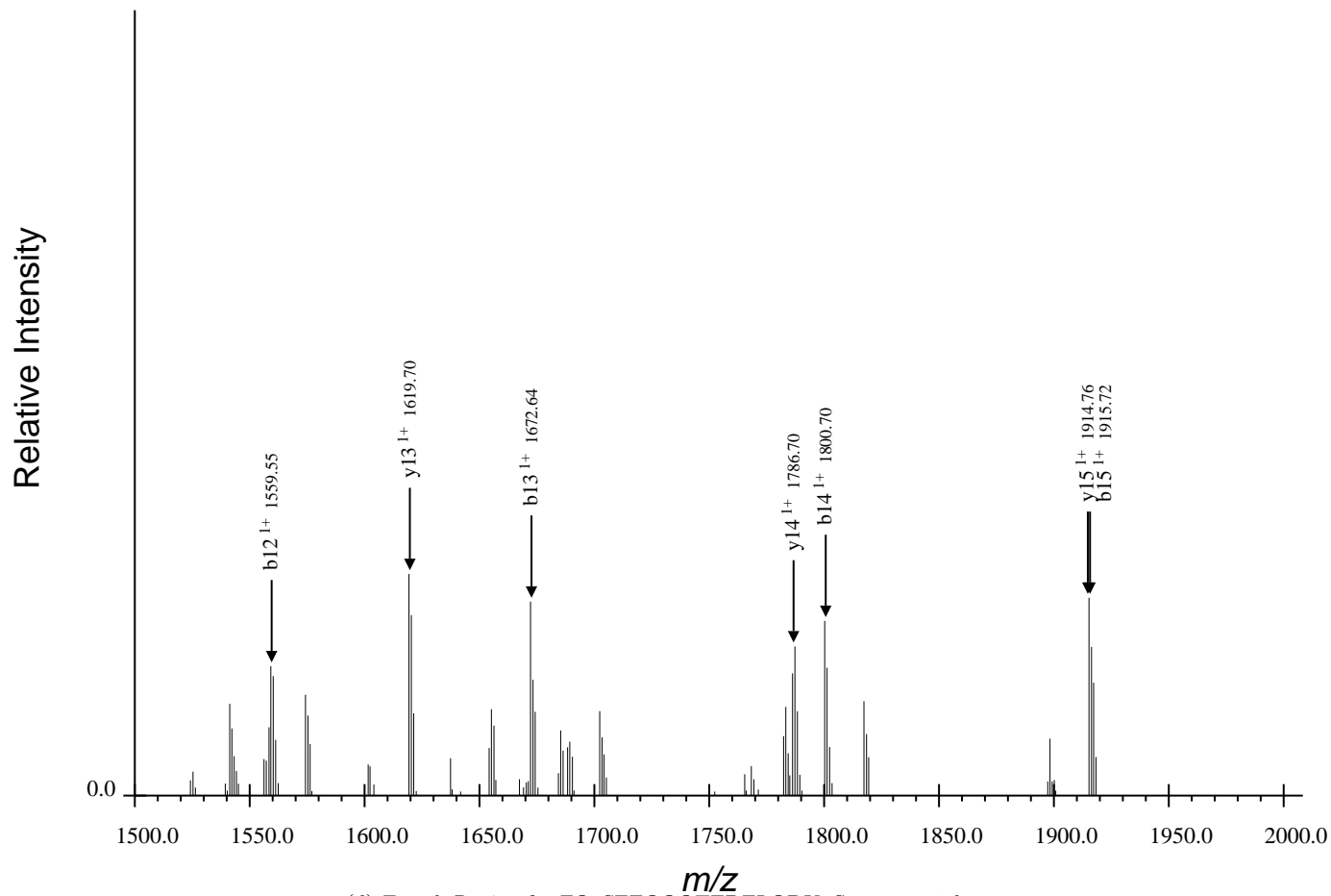
(d) Fourth Region for FQpSEEQQQTEDELQDK, Spectrum 1.dta
