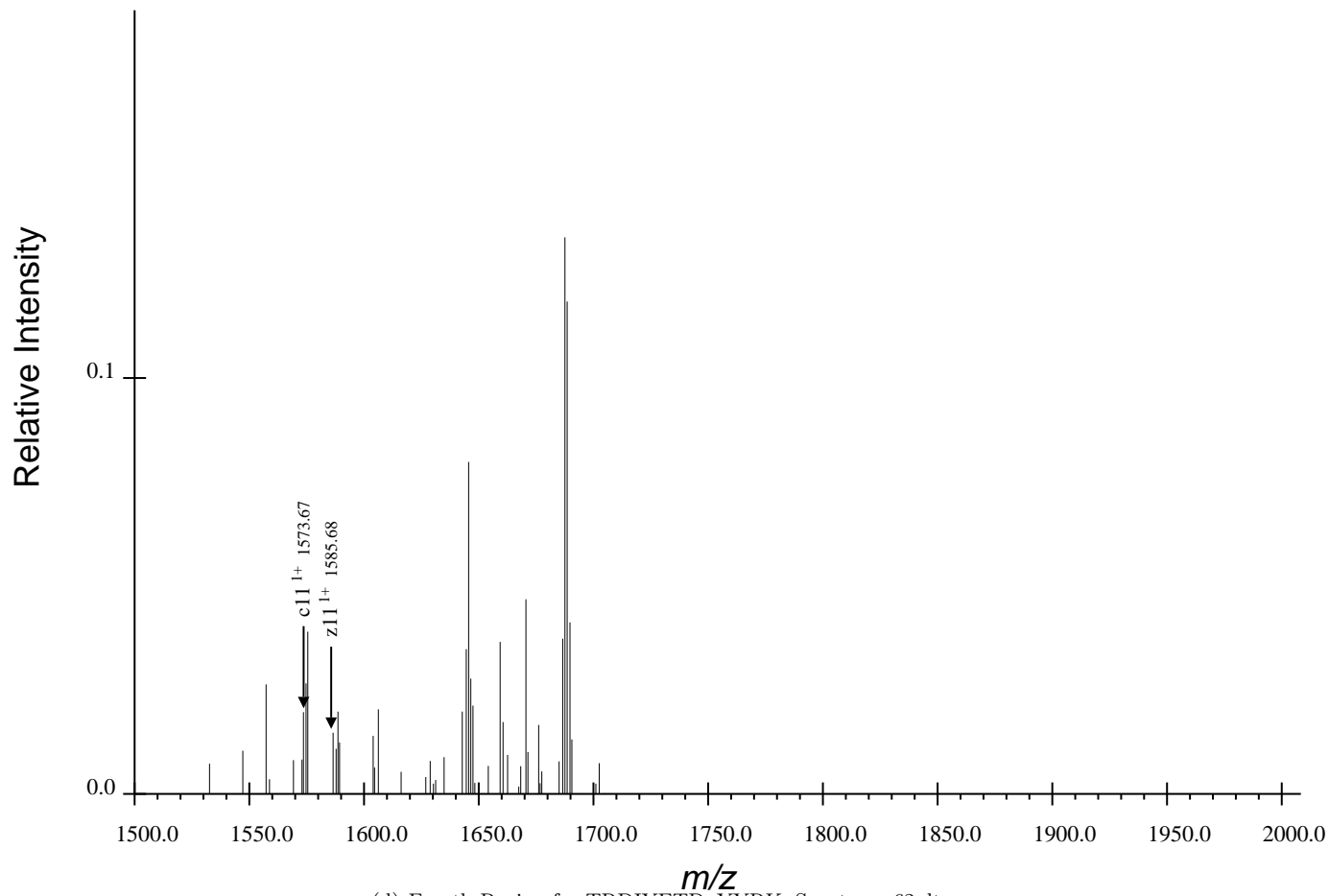
(d) Fourth Region for TRDIYETDpYYRK, Spectrum 62.dta
