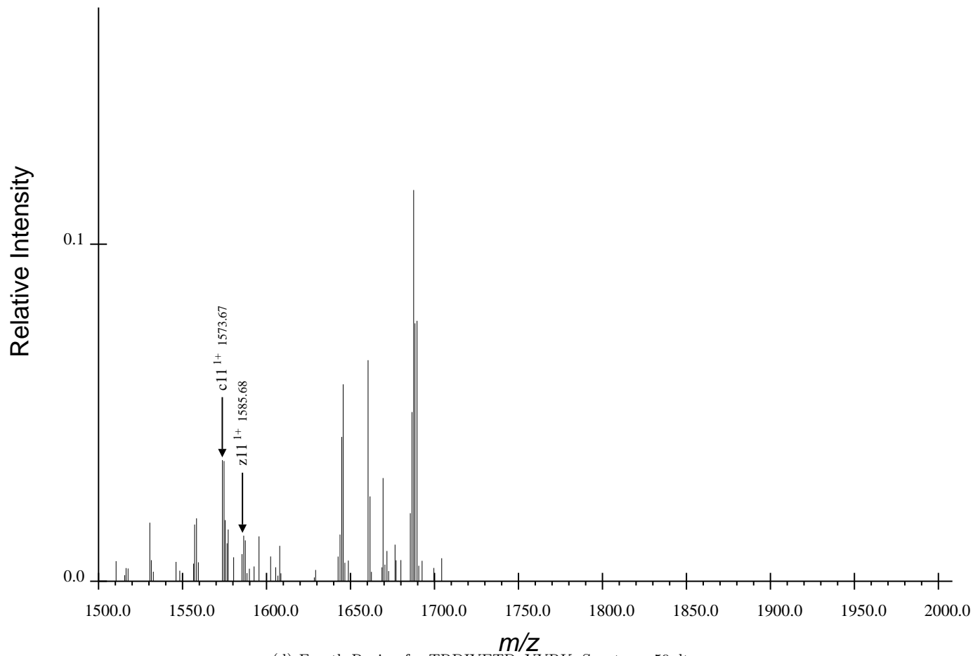
(d) Fourth Region for TRDIYETDpYYRK, Spectrum 59.dta
