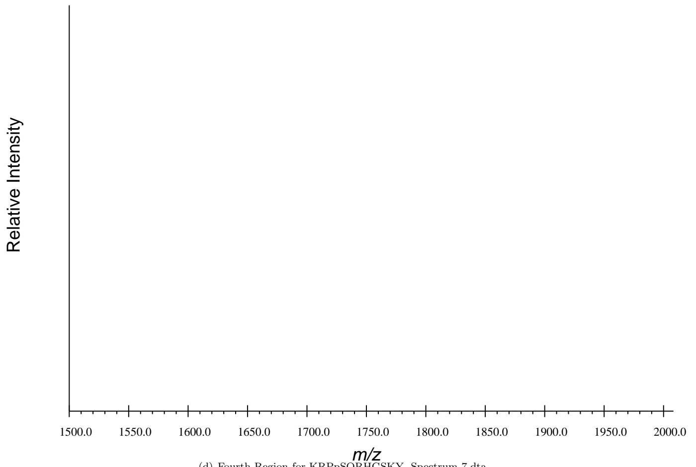
(d) Fourth Region for KRPPSQRHGSKY, Spectrum 7.dta
