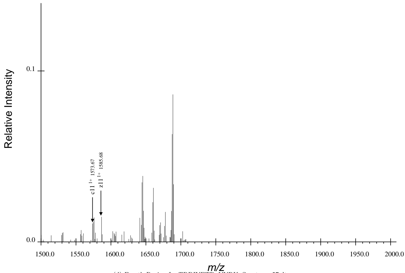
(d) Fourth Region for TRDIYETDpYYRK, Spectrum 57.dta
