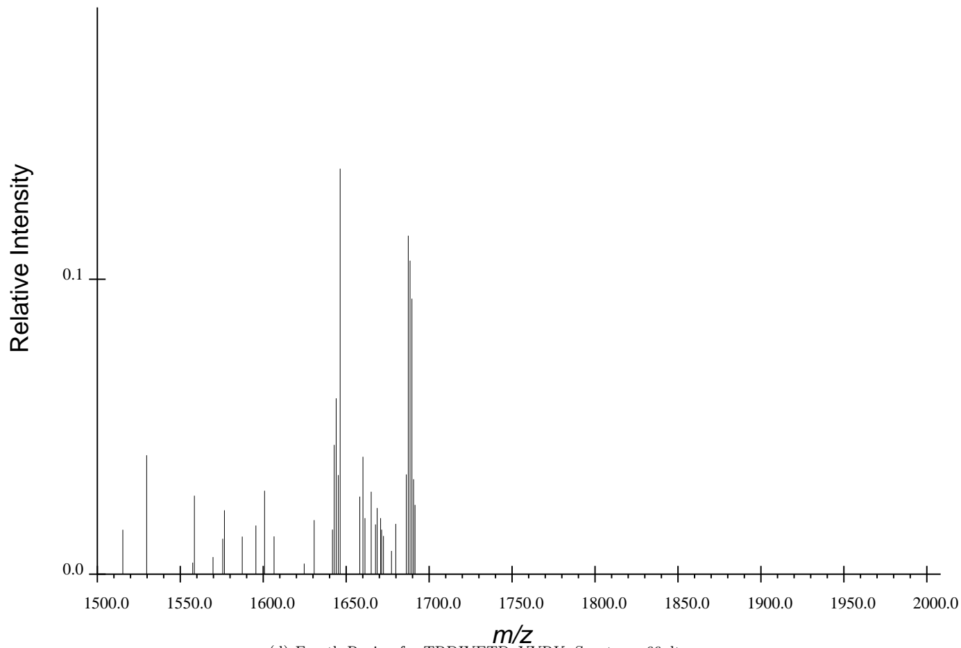
(d) Fourth Region for TRDIYETDpYYRK, Spectrum 66.dta
