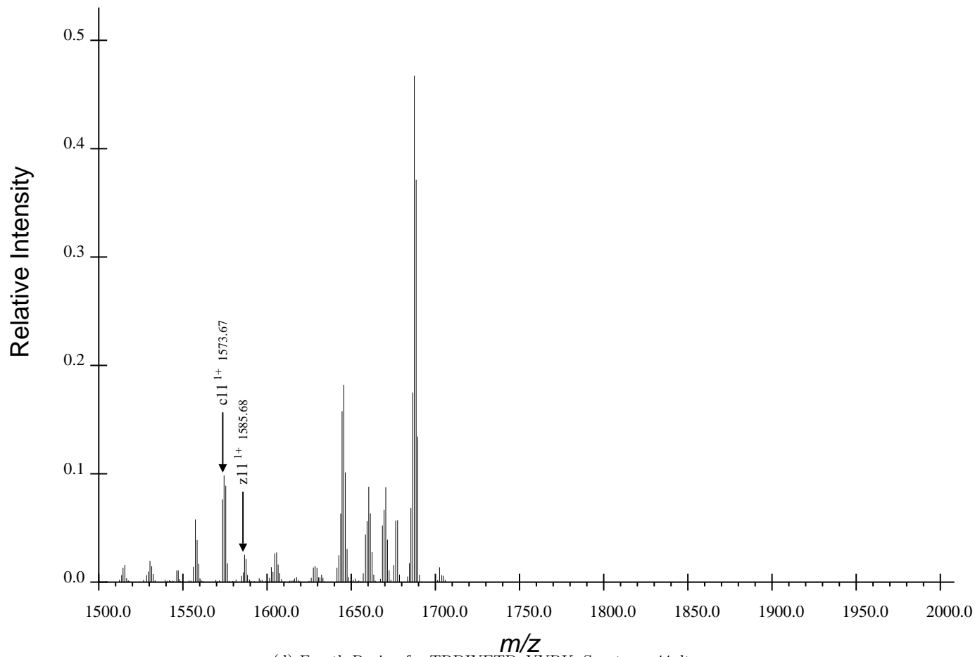
(d) Fourth Region for TRDIYETDpYYRK, Spectrum 44.dta
