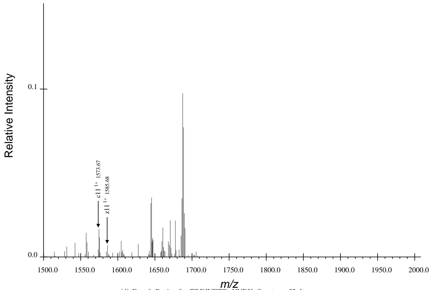
(d) Fourth Region for TRDIYETDpYYRK, Spectrum 55.dta
