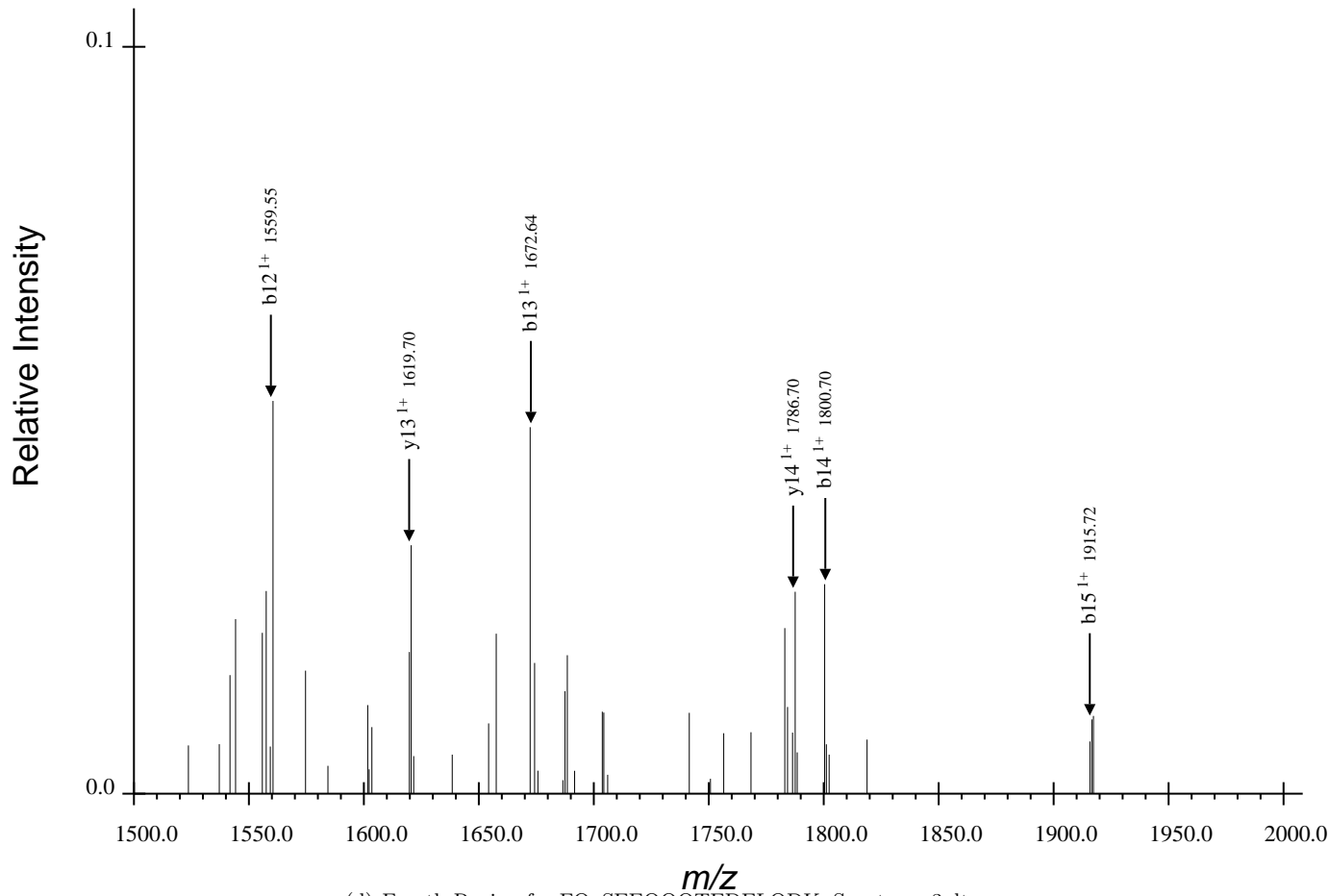
(d) Fourth Region for FQpSEEQQQTEDELQDK, Spectrum 3.dta
