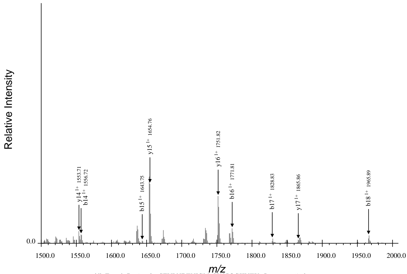
(d) Fourth Region for SFVLNPTNIGMpSKSSQGHVTK, Spectrum 17.dta
