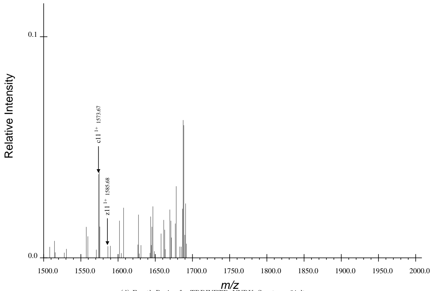
(d) Fourth Region for TRDIYETDpYYRK, Spectrum 64.dta
