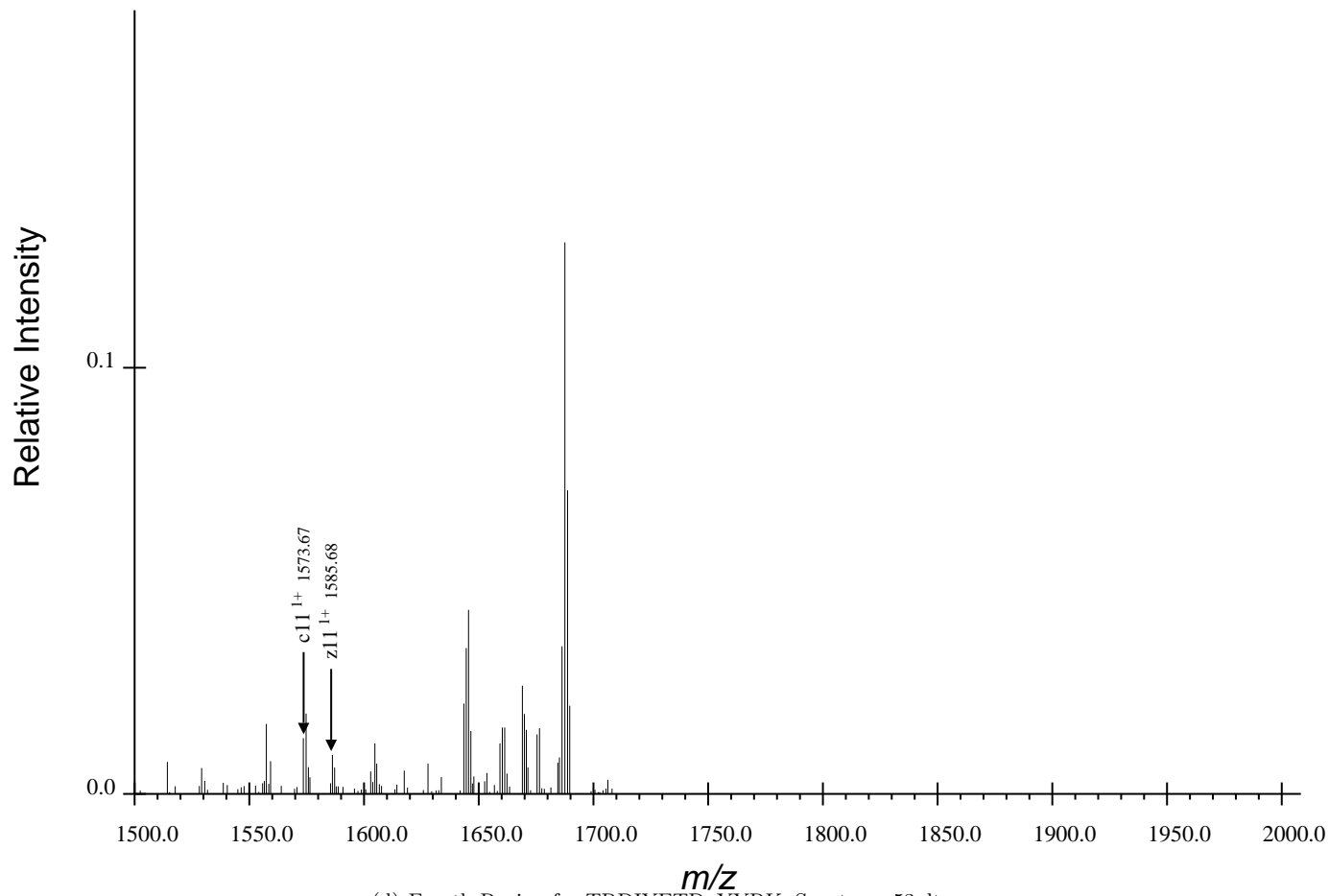
(d) Fourth Region for TRDIYETDpYYRK, Spectrum 53.dta
