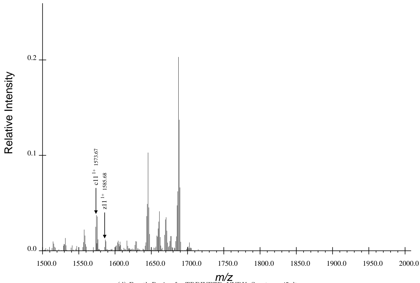
(d) Fourth Region for TRDIYETDpYYRK, Spectrum 45.dta
