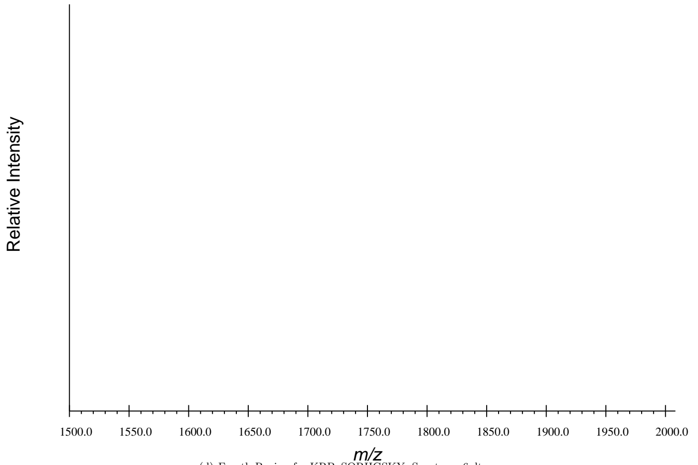
(d) Fourth Region for KRPpSQRHGSKY, Spectrum 6.dta
