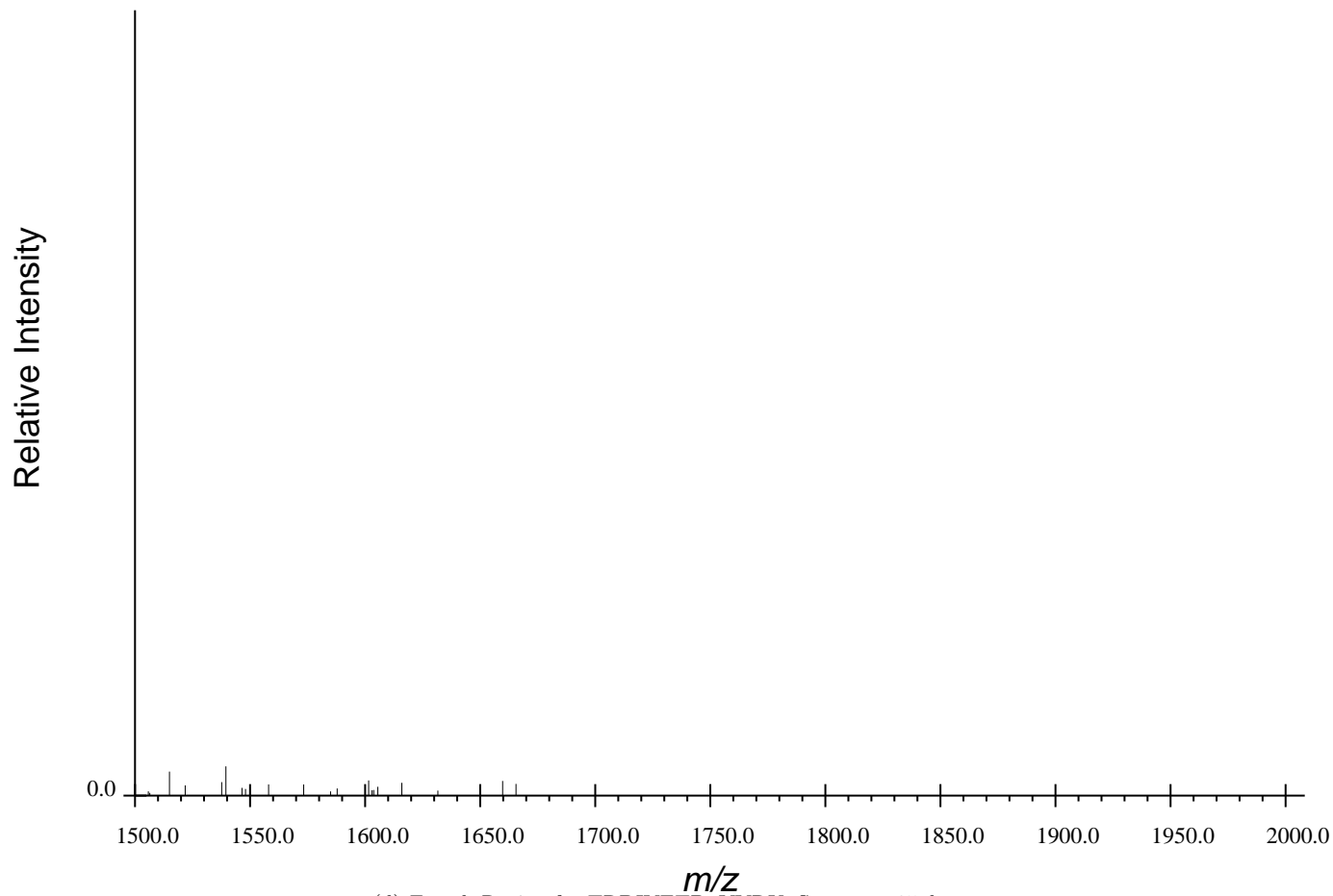
(d) Fourth Region for TRDIYETDpYYRK, Spectrum 35.dta
