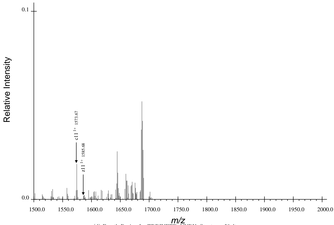
(d) Fourth Region for TRDIYETDpYYRK, Spectrum 52.dta
