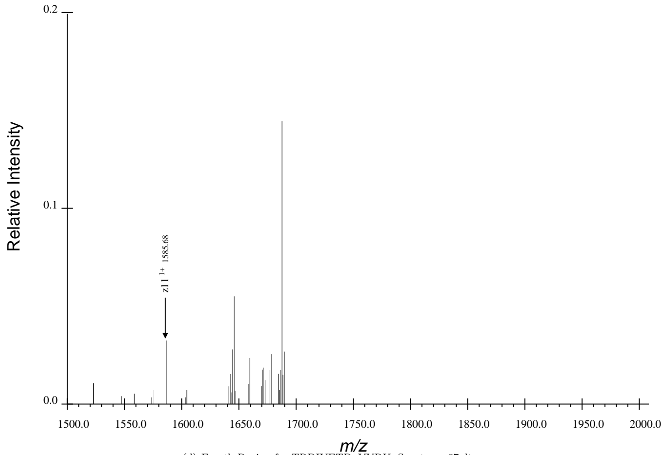
(d) Fourth Region for TRDIYETDpYYRK, Spectrum 67.dta
