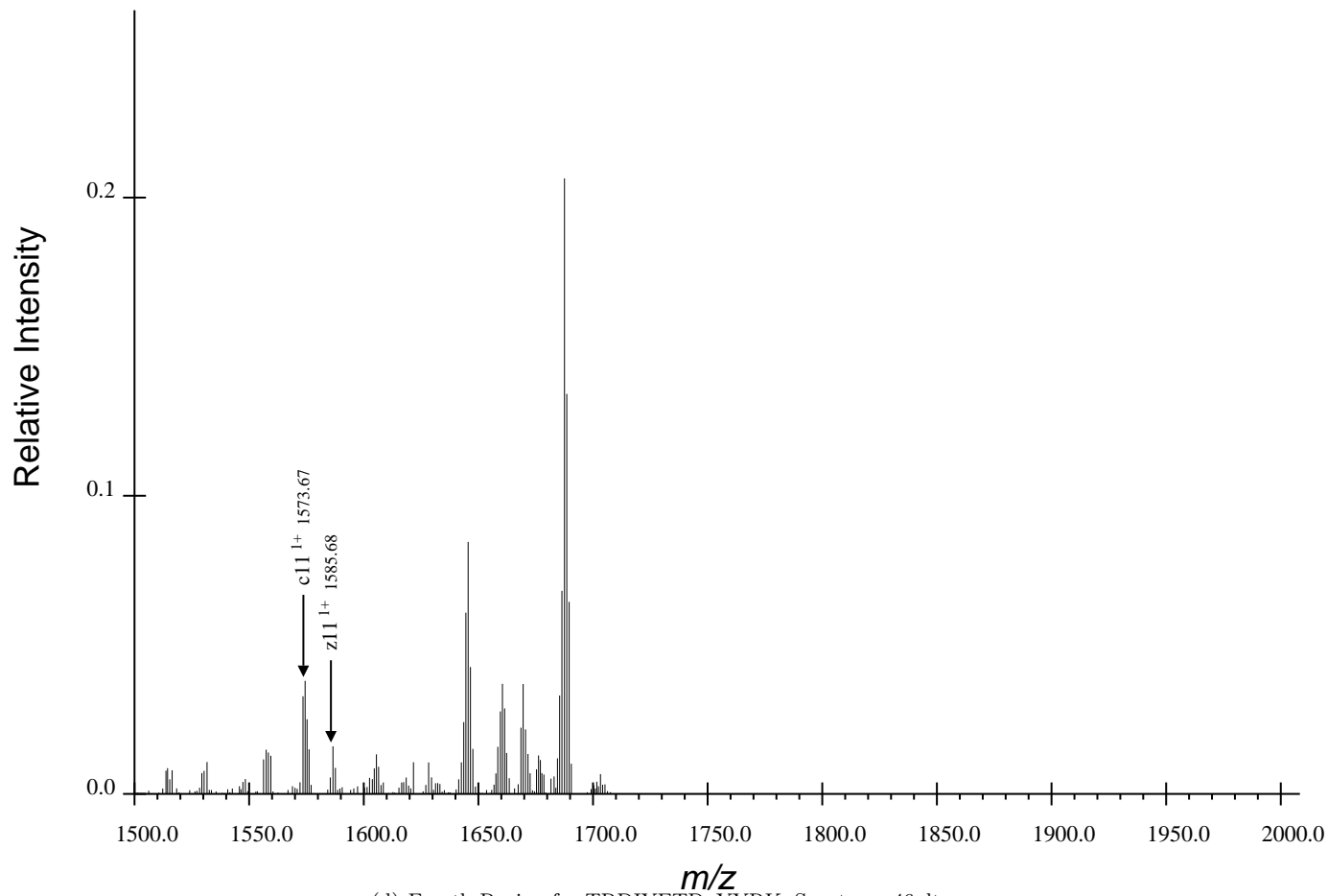
(d) Fourth Region for TRDIYETDpYYRK, Spectrum 46.dta
