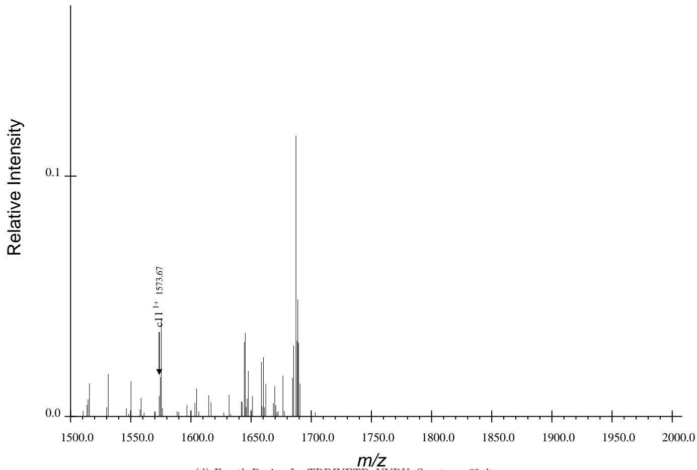
(d) Fourth Region for TRDIYETDpYYRK, Spectrum 60.dta
