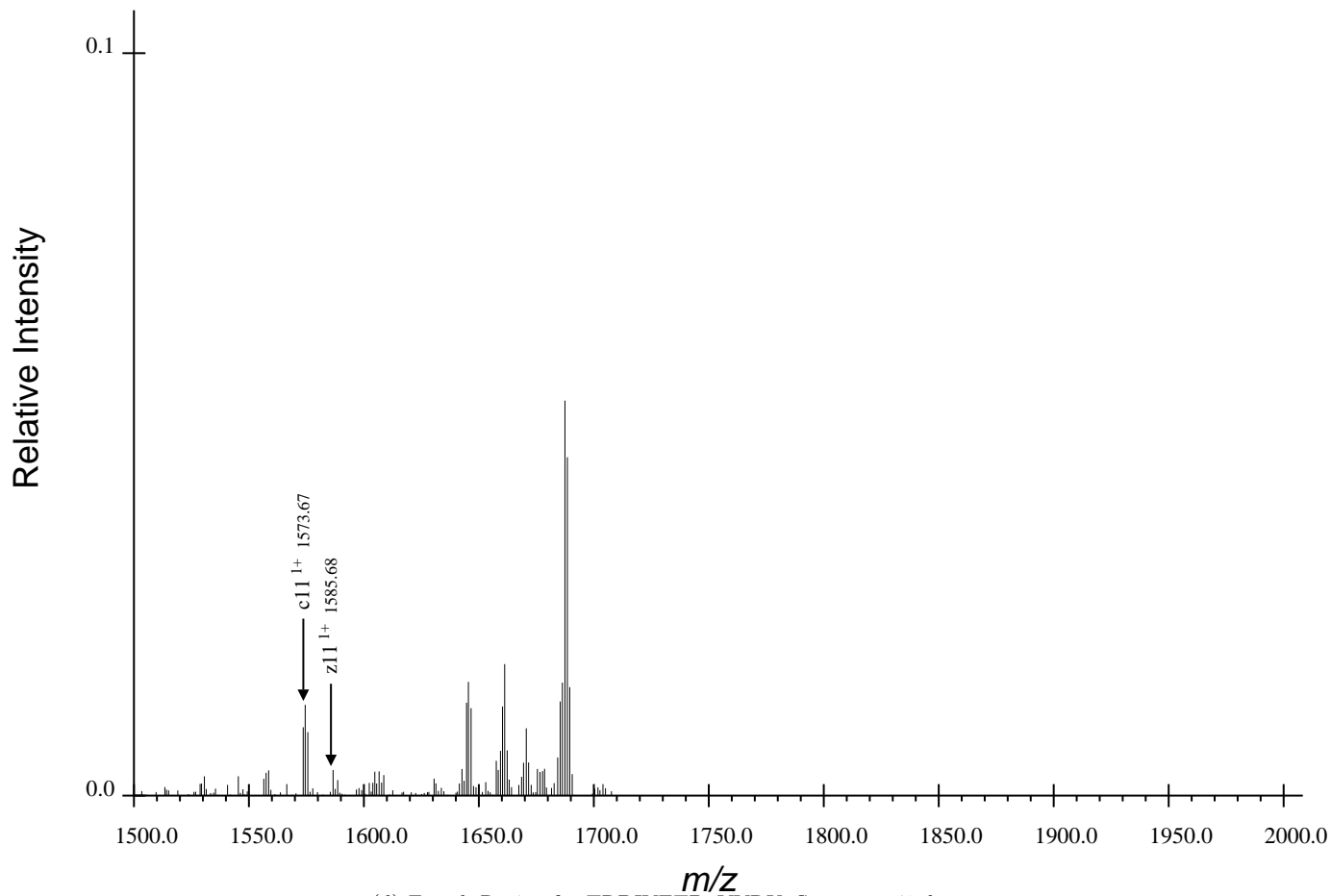
(d) Fourth Region for TRDIYETDpYYRK, Spectrum 49.dta
