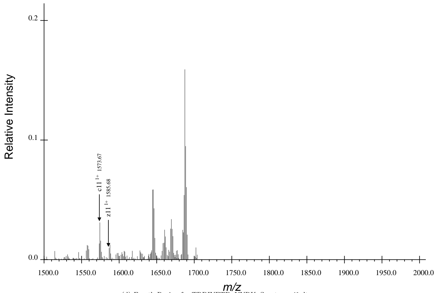
(d) Fourth Region for TRDIYETDpYYRK, Spectrum 41.dta
