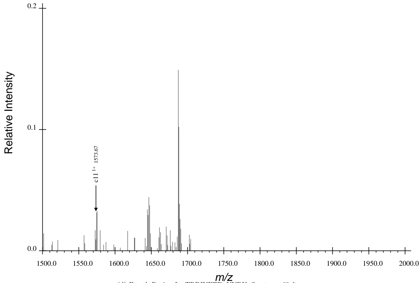
(d) Fourth Region for TRDIYETDpYYRK, Spectrum 63.dta
