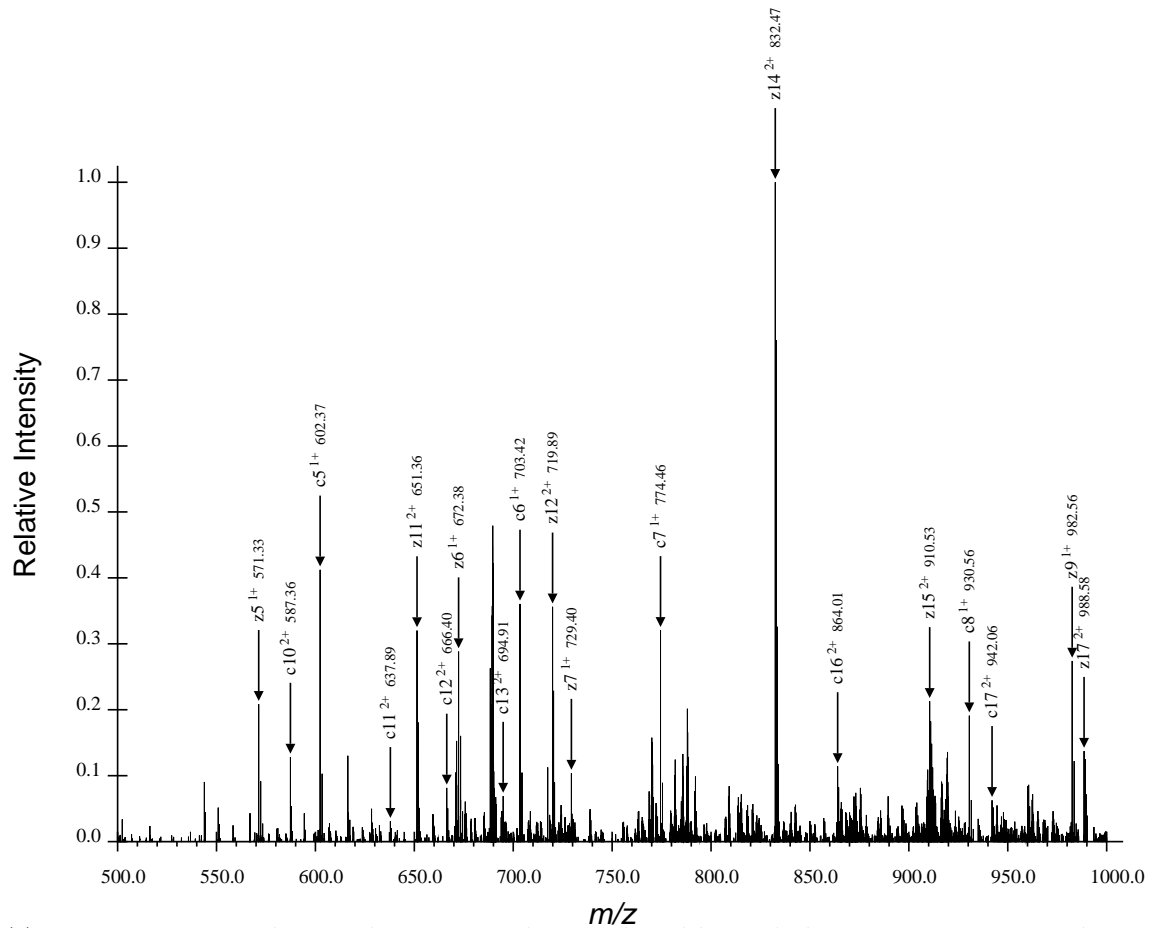
(b) Second Region for ARTKQTARdKSTGGaKAPRKQLATaKAARdKSAPATGGVdKKPHRYRPGTVALRE, Spectrum 50.dta
