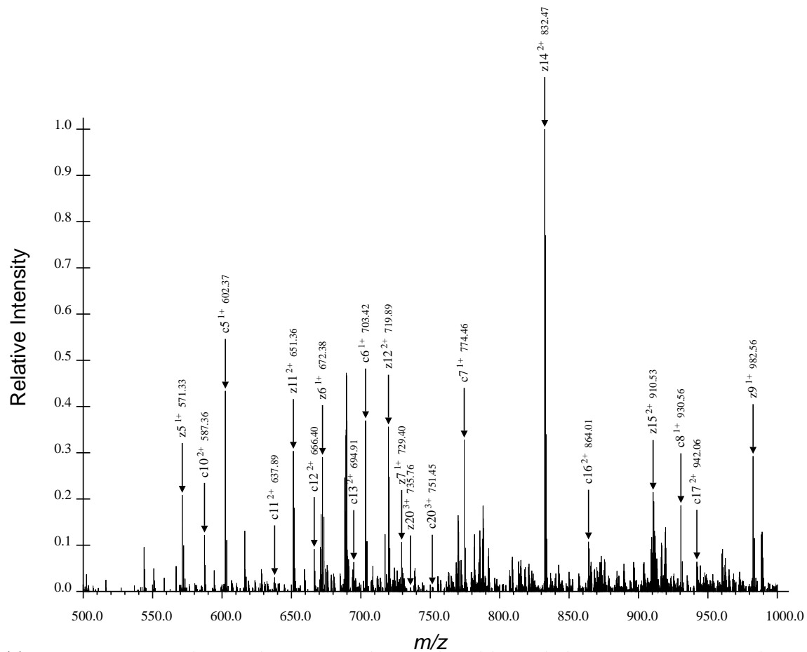
(b) Second Region for ARTKQTARdKSTGGaKAPRKQLATaKAARdKSAPATGGVdKKPHRYRPGTVALRE, Spectrum 57.dta
