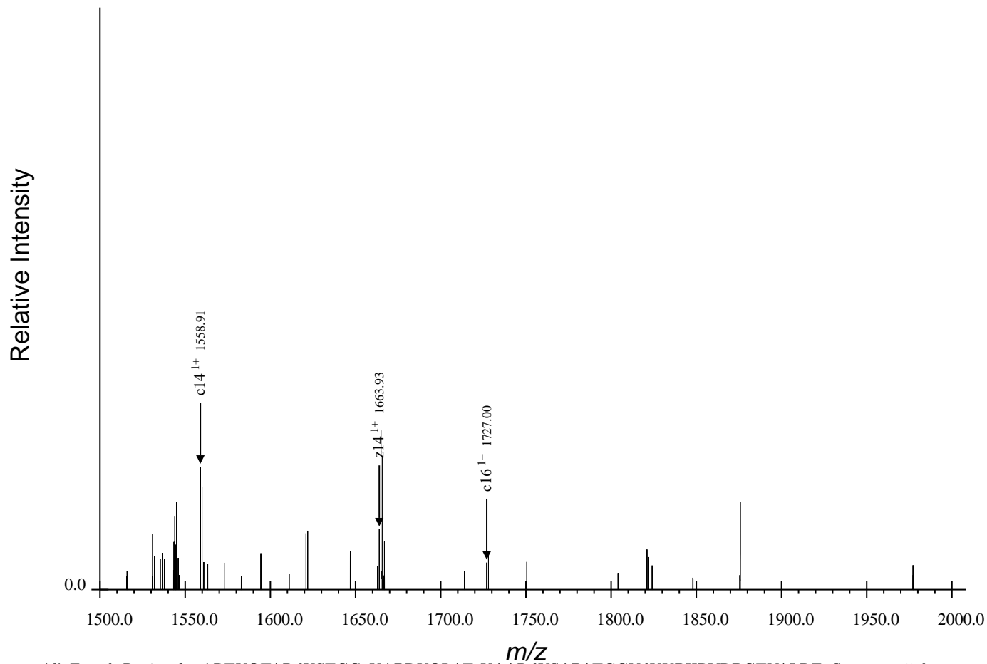
(d) Fourth Region for ARTKQTARdKSTGGaKAPRKQLATaKAARdKSAPATGGVdKKPHRYRPGTVALRE, Spectrum 5.dta
