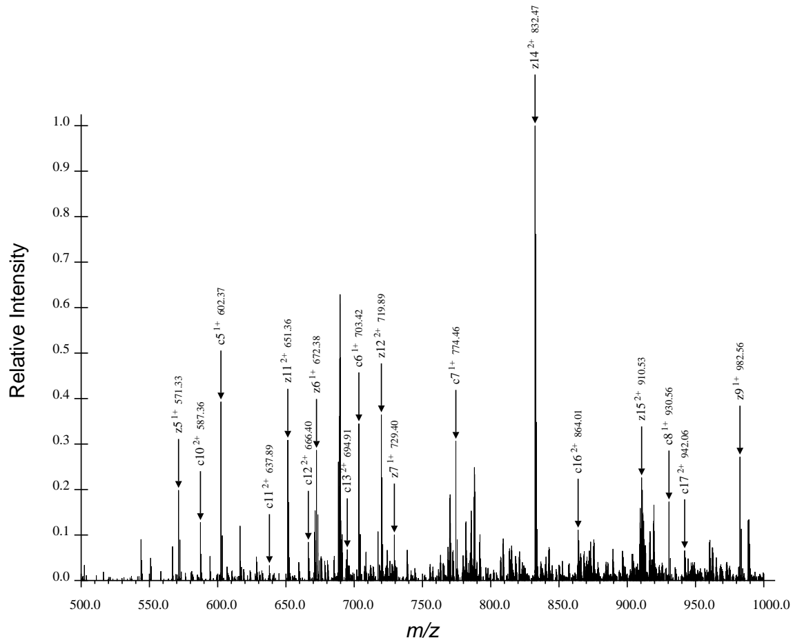
(b) Second Region for ARTKQTARdKSTGGaKAPRKQLATaKAARdKSAPATGGVdKKPHRYRPGTVALRE, Spectrum 33.dta
