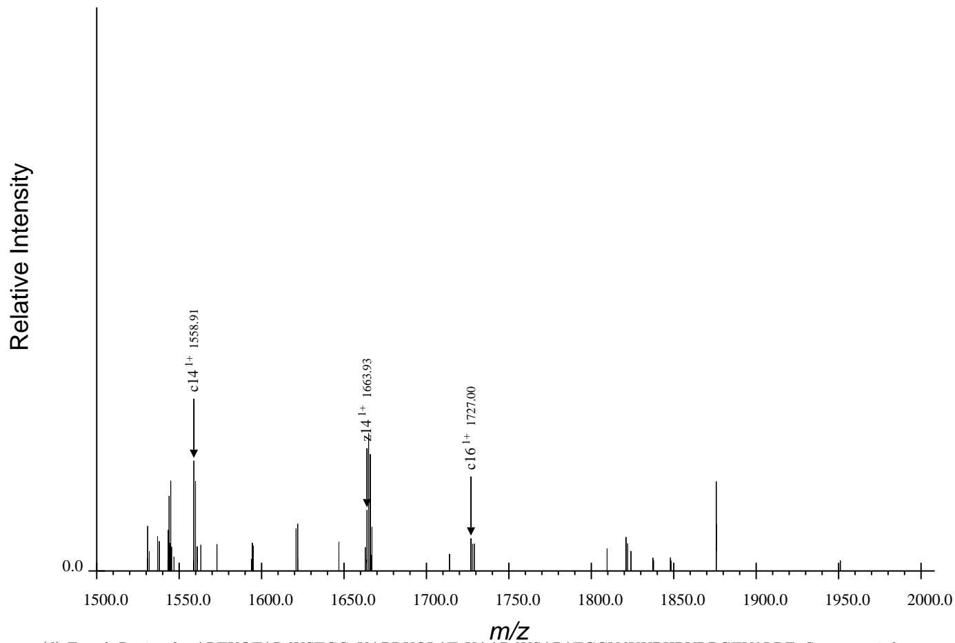
(d) Fourth Region for ARTKQTARdKSTGGaKAPRKQLATaKAARdKSAPATGGVdKKPHRYRPGTVALRE, Spectrum 2.dta
