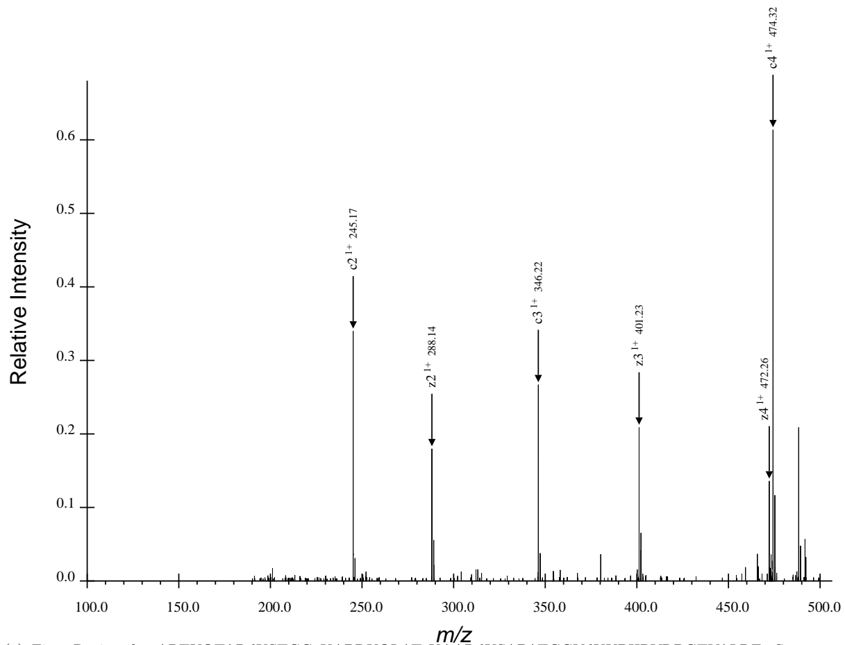
(a) First Region for ARTKQTARdKSTGGaKAPRKQLATaKAARdKSAPATGGVdKKPHRYRPGTVALRE, Spectrum 58.dta
