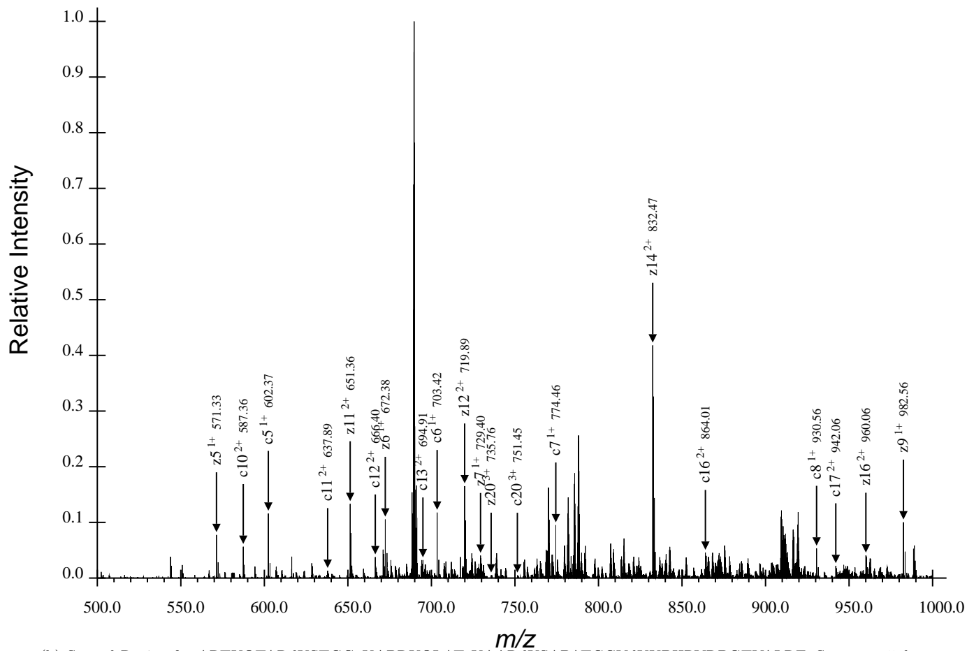
(b) Second Region for ARTKQTARdKSTGGaKAPRKQLATAKaARdKSAPATGGVdKKPHRYRPGTVALRE, Spectrum 5.dta
