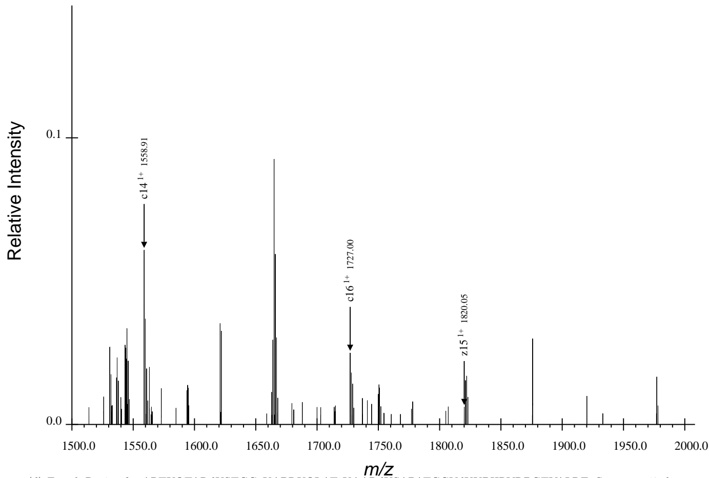
(d) Fourth Region for ARTKQTARdKSTGGaKAPRKQLATaKAARdKSAPATGGVdKKPHRYRPGTVALRE, Spectrum 37.dta
