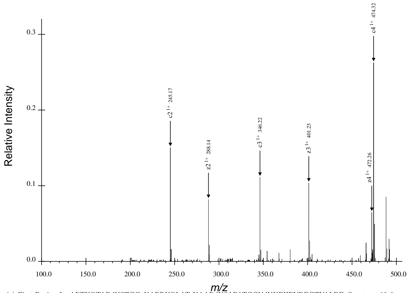
(a) First Region for ARTKQTARdKSTGGaKAPRKQLATaKAARdKSAPATGGVdKKPHRYRPGTVALRE, Spectrum 10.dta
