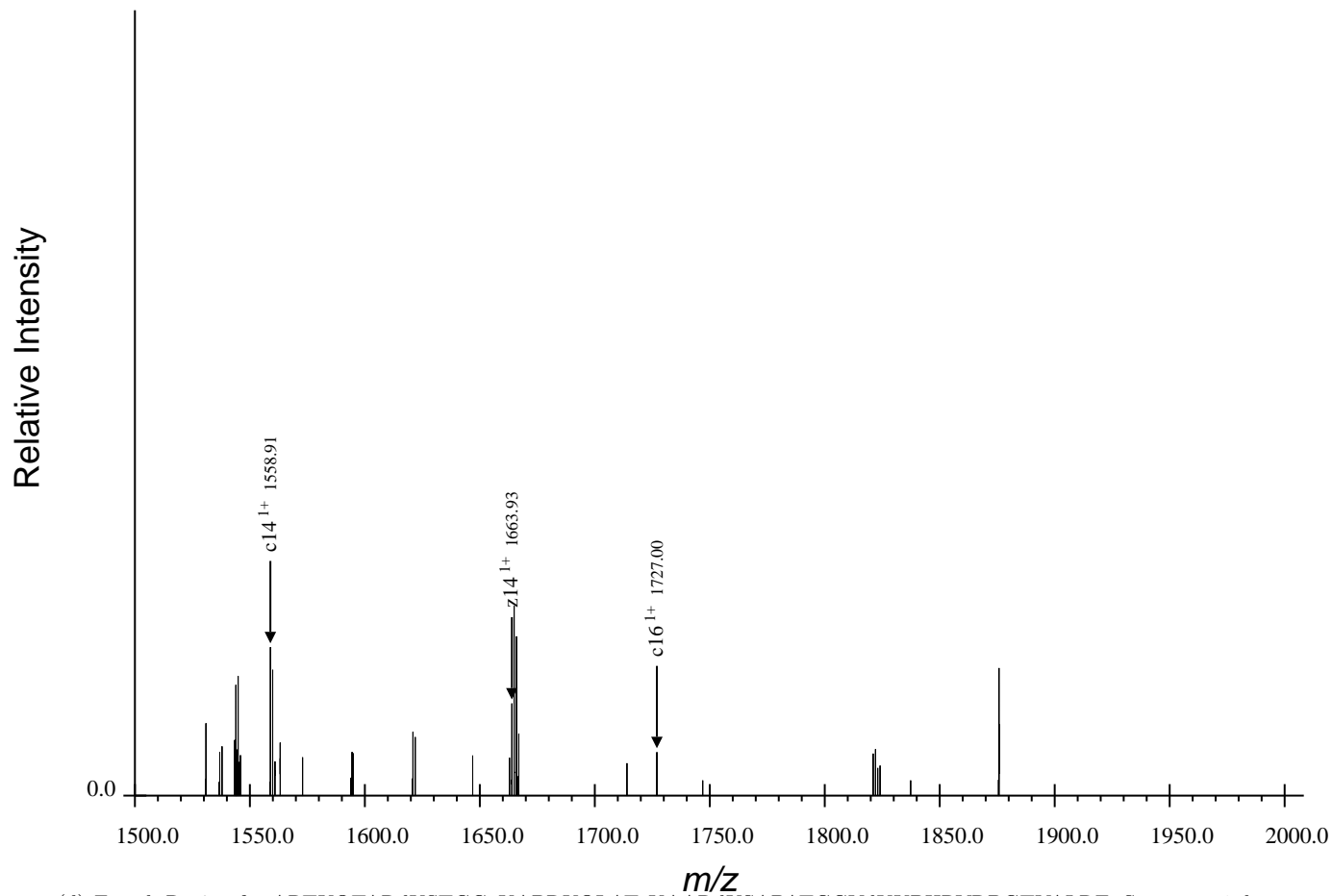
(d) Fourth Region for ARTKQTARdKSTGGaKAPRKQLATaKAARdKSAPATGGVdKKPHRYRPGTVALRE, Spectrum 1.dta
