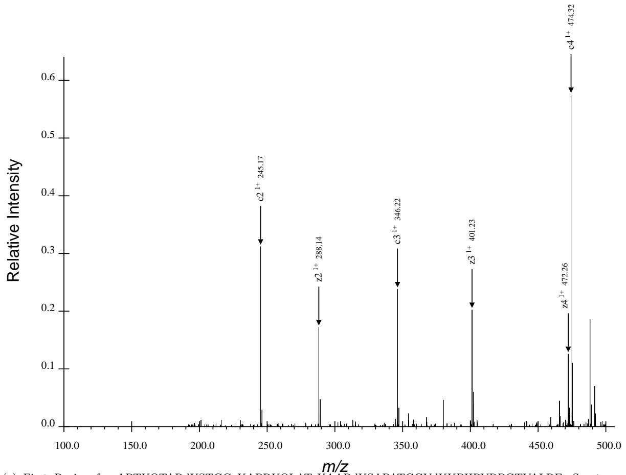
(a) First Region for ARTKQTARdKSTGGaKAPRKQLATaKAARdKSAPATGGVdKKPHRYRPGTVALRE, Spectrum 28.dta
