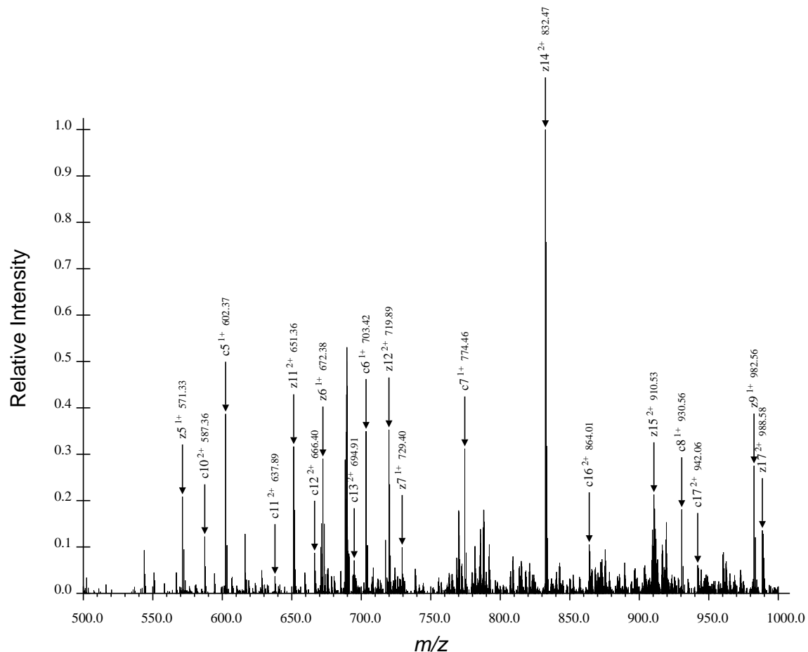
(b) Second Region for ARTKQTARdKSTGGaKAPRKQLATaKAARdKSAPATGGVdKKPHRYRPGTVALRE, Spectrum 41.dta
