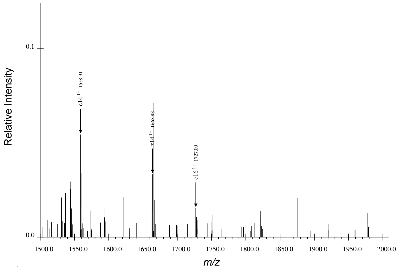
(d) Fourth Region for ARTKQTARdKSTGGaKAPRKQLATaKAARdKSAPATGGVdKKPHRYRPGTVALRE, Spectrum 23.dta
