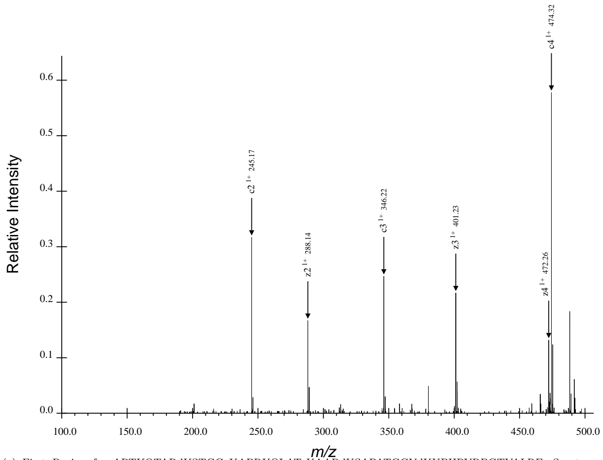
(a) First Region for ARTKQTARdKSTGGaKAPRKQLATaKAARdKSAPATGGVdKKPHRYRPGTVALRE, Spectrum 40.dta
