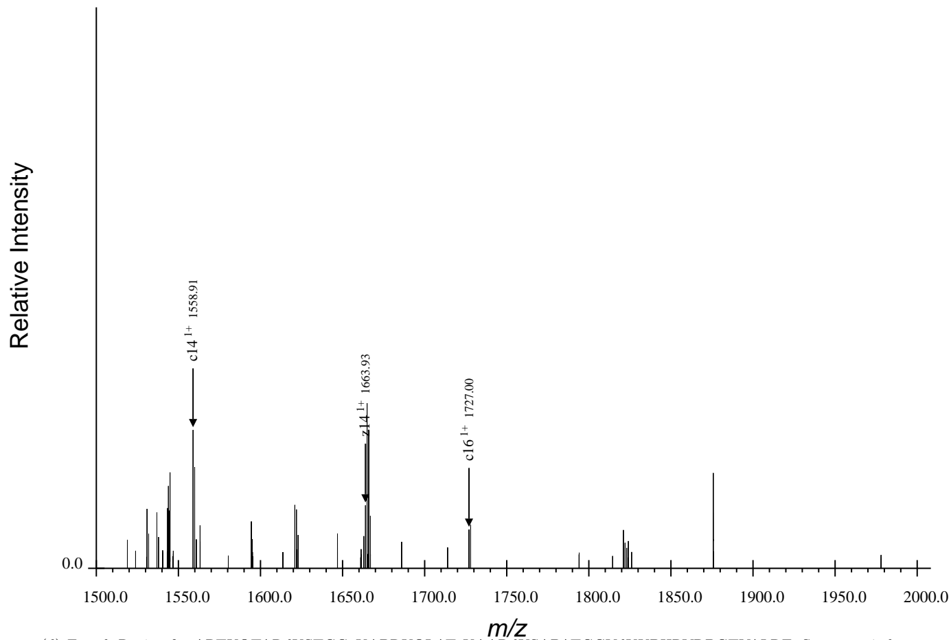
(d) Fourth Region for ARTKQTARdKSTGGaKAPRKQLATaKAARdKSAPATGGVdKKPHRYRPGTVALRE, Spectrum 7.dta
