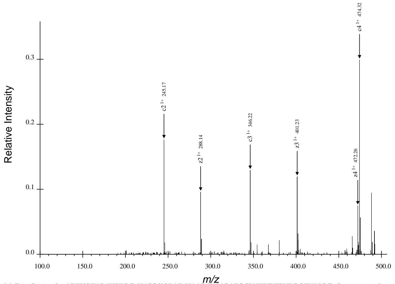
(a) First Region for ARTKQTARdKSTGGaKAPRKQLATaKAARdKSAPATGGVdKKPHRYRPGTVALRE, Spectrum 12.dta
