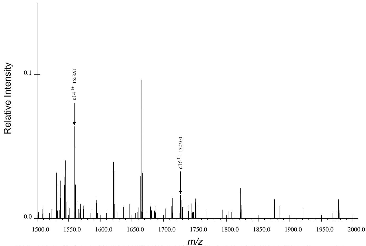
(d) Fourth Region for ARTKQTARdKSTGGaKAPRKQLATaKAARdKSAPATGGVdKKPHRYRPGTVALRE, Spectrum 56.dta
