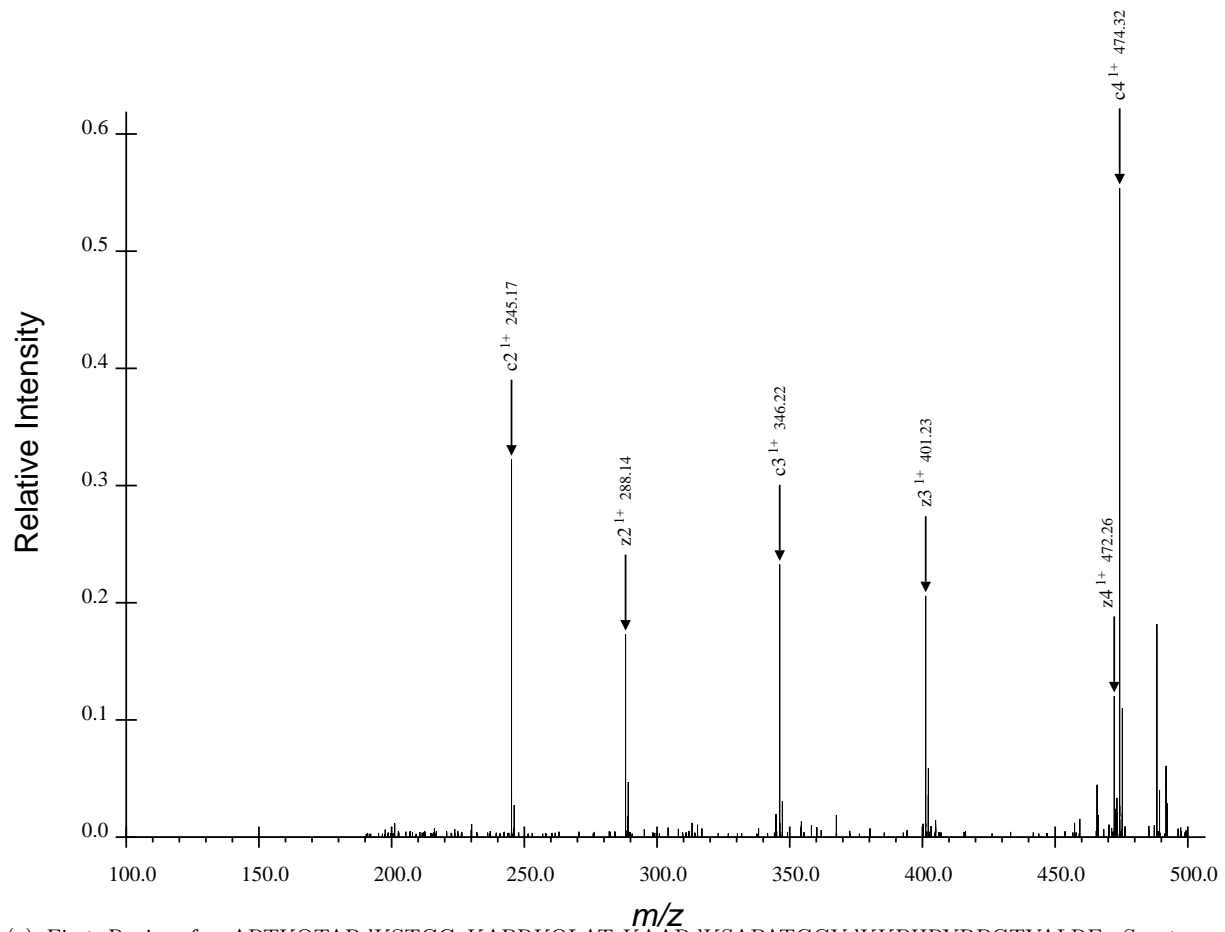
(a) First Region for ARTKQTARdKSTGGaKAPRKQLATaKAARdKSAPATGGVdKKPHRYRPGTVALRE, Spectrum 22.dta
