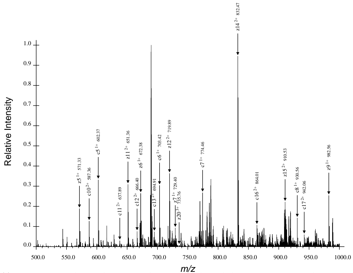
(b) Second Region for ARTKQTARdKSTGGaKAPRKQLATaKAARdKSAPATGGVdKKPHRYRPGTVALRE, Spectrum 20.dta
