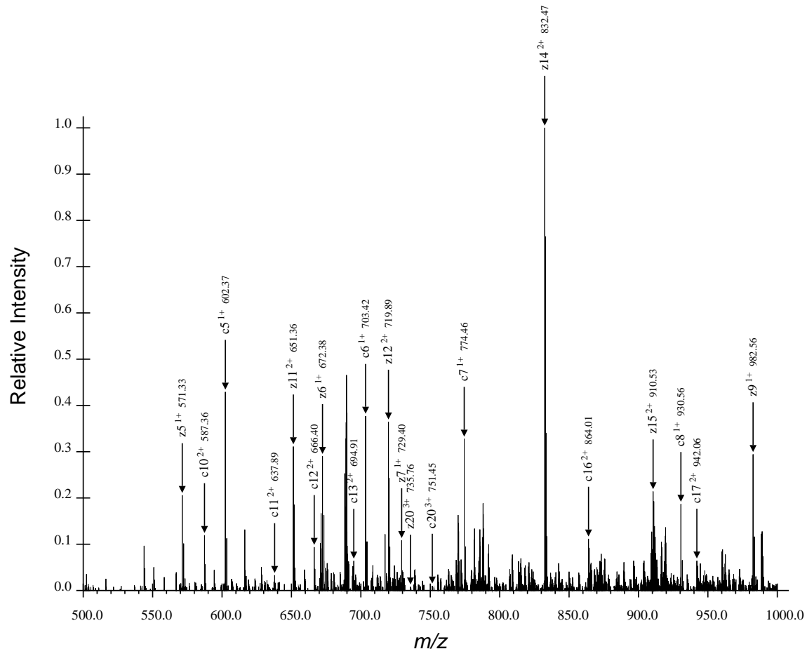
(b) Second Region for ARTKQTARdKSTGGaKAPRKQLATaKAARdKSAPATGGVdKKPHRYRPGTVALRE, Spectrum 56.dta
