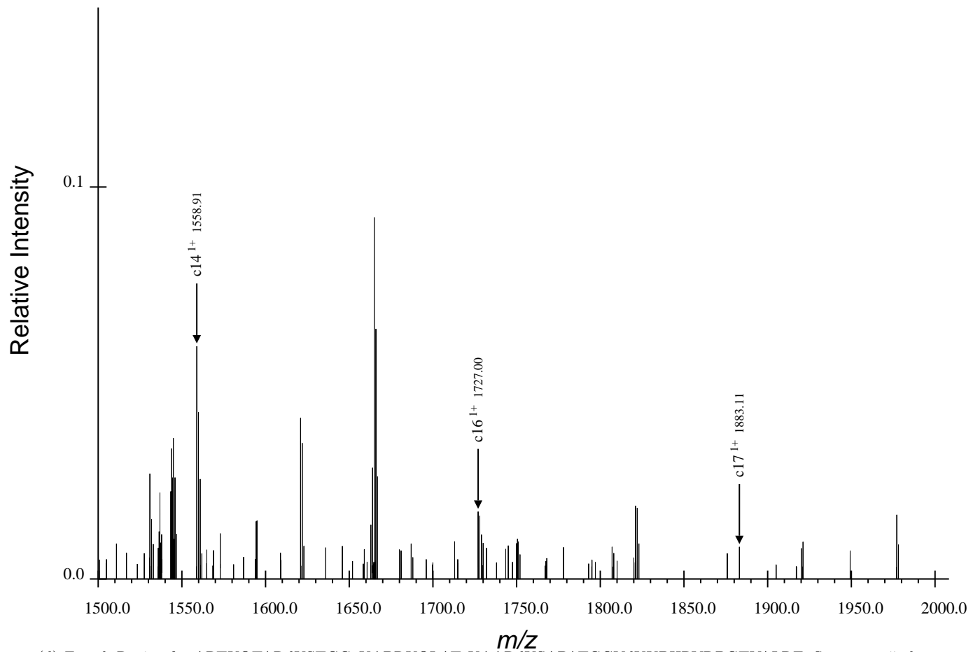
(d) Fourth Region for ARTKQTARdKSTGGaKAPRKQLATaKAARdKSAPATGGVdKKPHRYRPGTVALRE, Spectrum 47.dta
