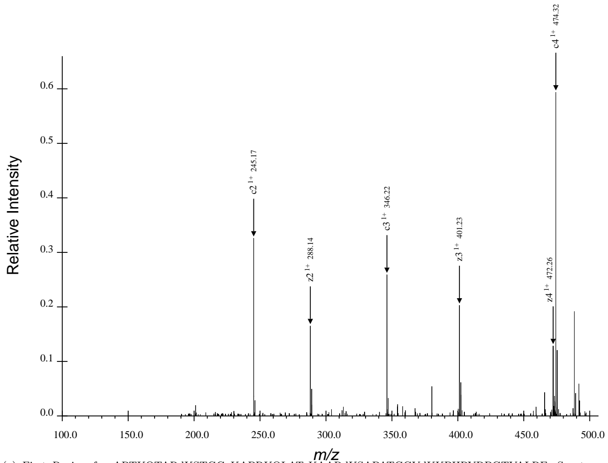
(a) First Region for ARTKQTARdKSTGGaKAPRKQLATaKAARdKSAPATGGVdKKPHRYRPGTVALRE, Spectrum 50.dta
