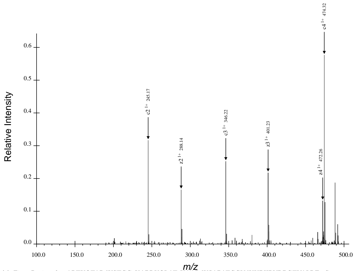
(a) First Region for ARTKQTARdKSTGGaKAPRKQLATaKAARdKSAPATGGVdKKPHRYRPGTVALRE, Spectrum 41.dta
