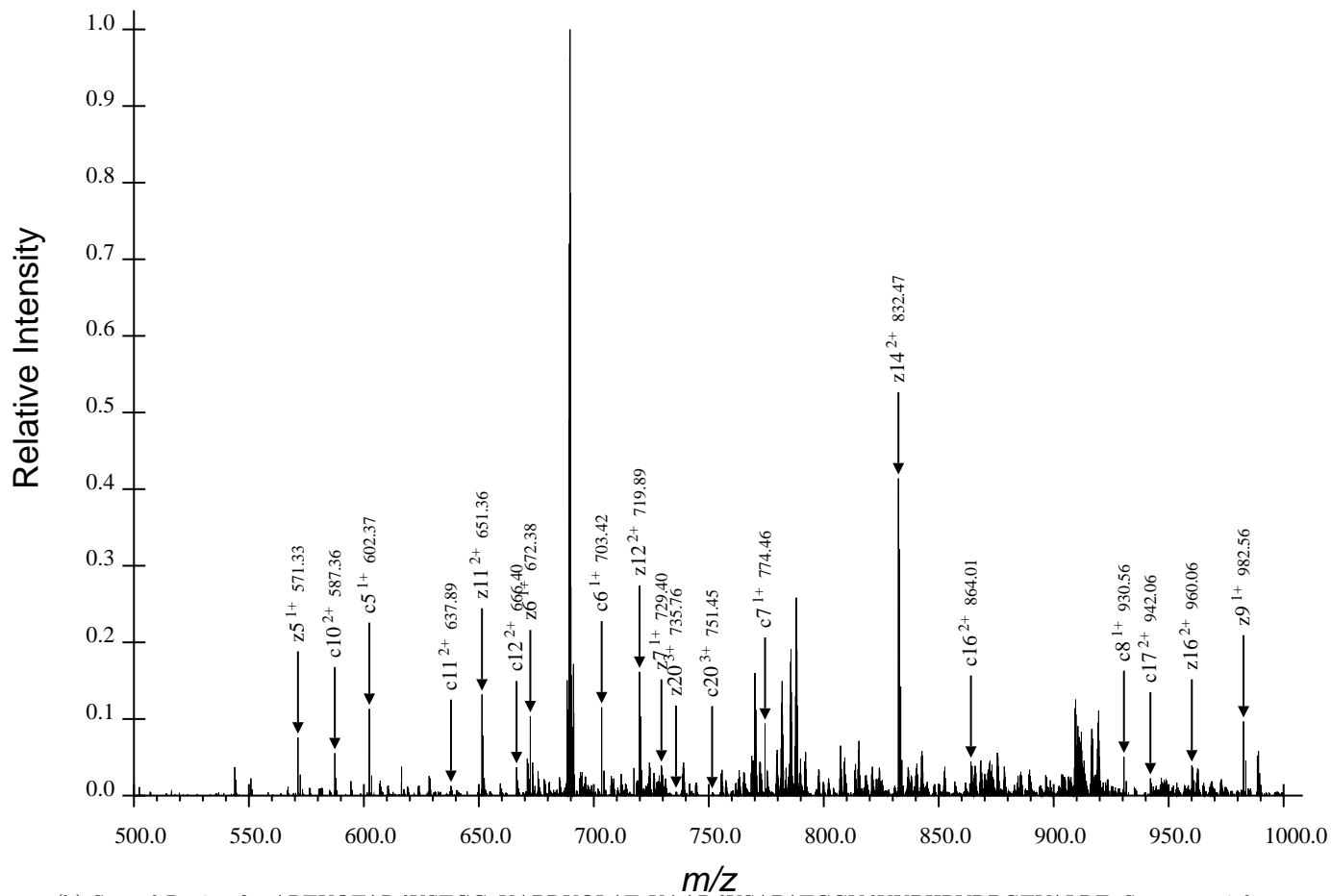
(b) Second Region for ARTKQTARdKSTGGaKAPRKQLATAKaARdKSAPATGGVdKKPHRYRPGTVALRE, Spectrum 4.dta
