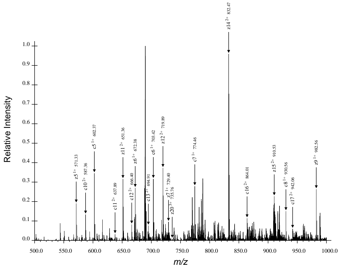
(b) Second Region for ARTKQTARdKSTGGaKAPRKQLATaKAARdKSAPATGGVdKKPHRYRPGTVALRE, Spectrum 21.dta
