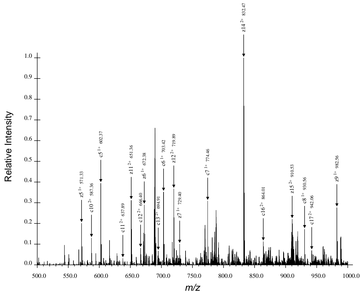
(b) Second Region for ARTKQTARdKSTGGaKAPRKQLATaKAARdKSAPATGGVdKKPHRYRPGTVALRE, Spectrum 32.dta
