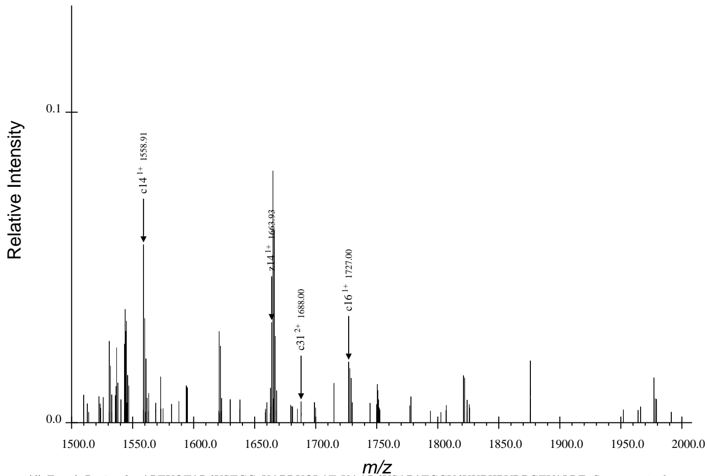
(d) Fourth Region for ARTKQTARdKSTGGaKAPRKQLATaKAARdKSAPATGGVdKKPHRYRPGTVALRE, Spectrum 31.dta
