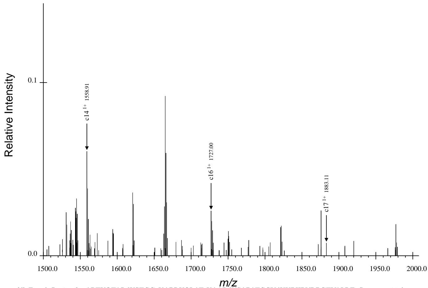
(d) Fourth Region for ARTKQTARdKSTGGaKAPRKQLATaKAARdKSAPATGGVdKKPHRYRPGTVALRE, Spectrum 39.dta
