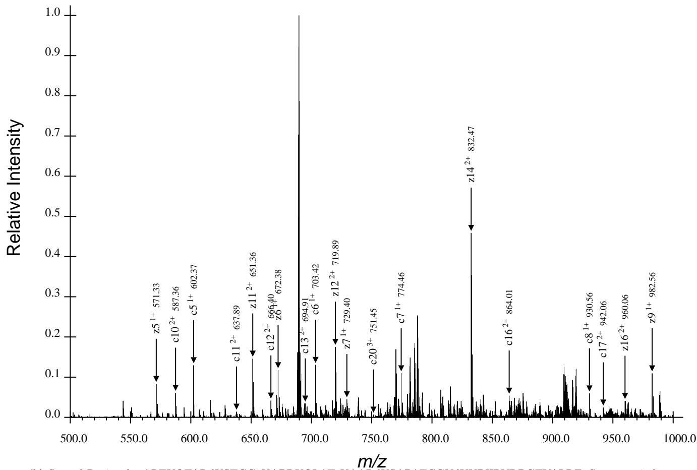
(b) Second Region for ARTKQTARdKSTGGaKAPRKQLATaKAARdKSAPATGGVdKKPHRYRPGTVALRE, Spectrum 7.dta
