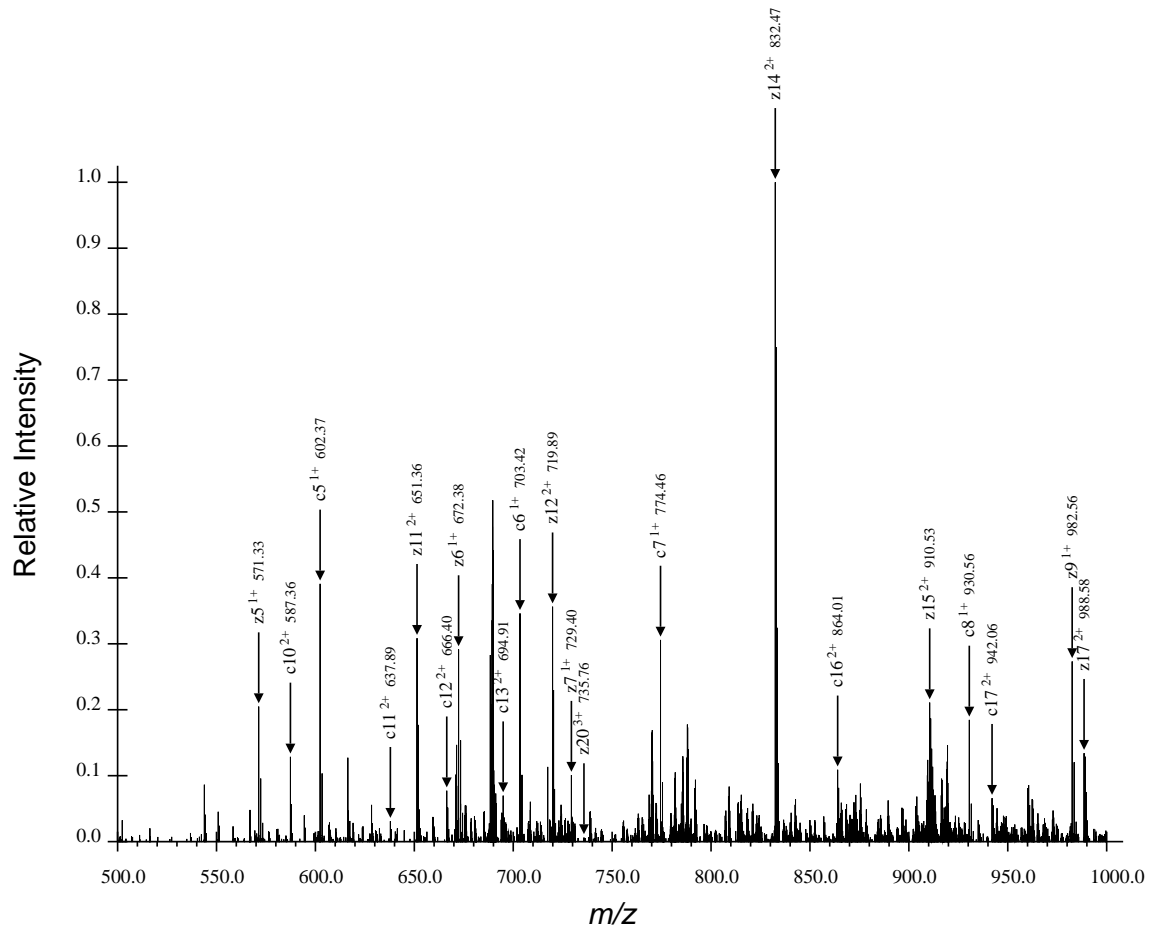
(b) Second Region for ARTKQTARdKSTGGaKAPRKQLATaKAARdKSAPATGGVdKKPHRYRPGTVALRE, Spectrum 45.dta
