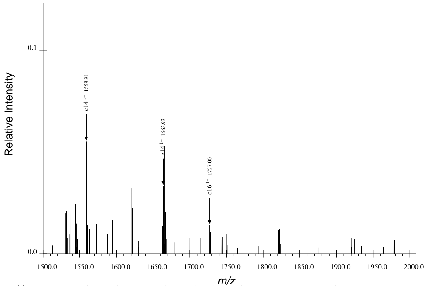
(d) Fourth Region for ARTKQTARdKSTGGaKAPRKQLATaKAARdKSAPATGGVdKKPHRYRPGTVALRE, Spectrum 24.dta
