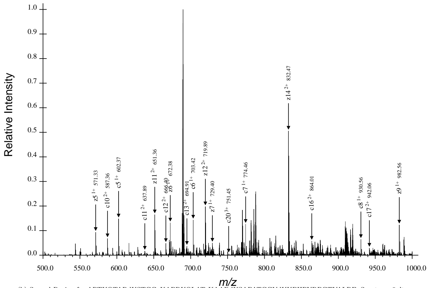
(b) Second Region for ARTKQTARdKSTGGaKAPRKQLATaKAARdKSAPATGGVdKKPHRYRPGTVALRE, Spectrum 9.dta
