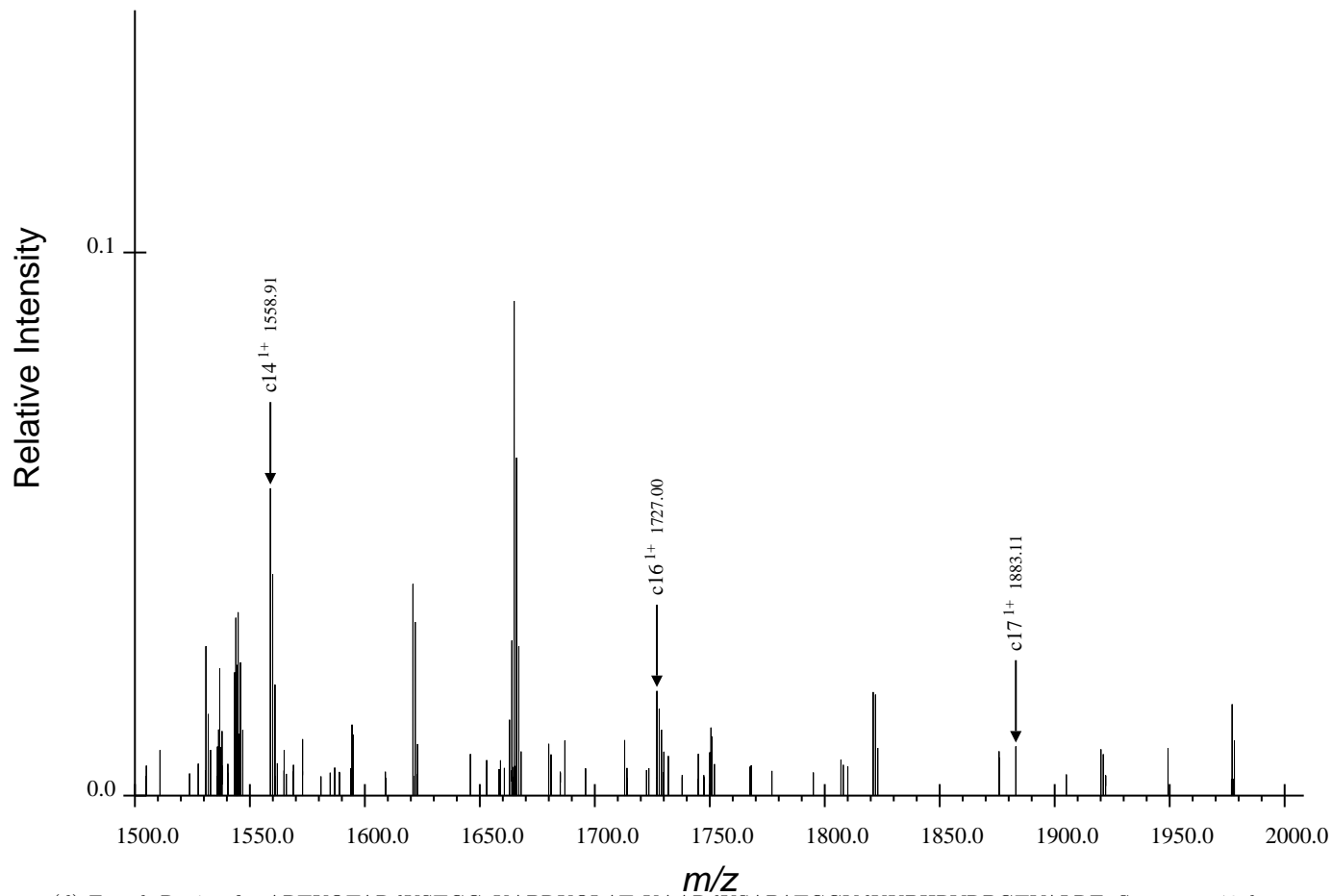
(d) Fourth Region for ARTKQTARdKSTGGaKAPRKQLATaKAARdKSAPATGGVdKKPHRYRPGTVALRE, Spectrum 46.dta
