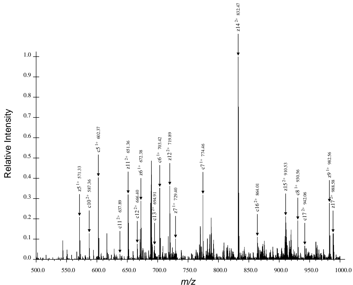
(b) Second Region for ARTKQTARdKSTGGaKAPRKQLATaKAARdKSAPATGGVdKKPHRYRPGTVALRE, Spectrum 48.dta
