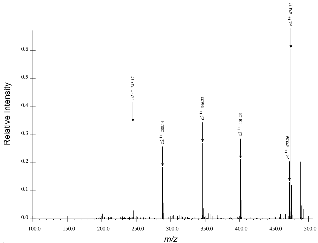
(a) First Region for ARTKQTARdKSTGGaKAPRKQLATaKAARdKSAPATGGVdKKPHRYRPGTVALRE, Spectrum 55.dta
