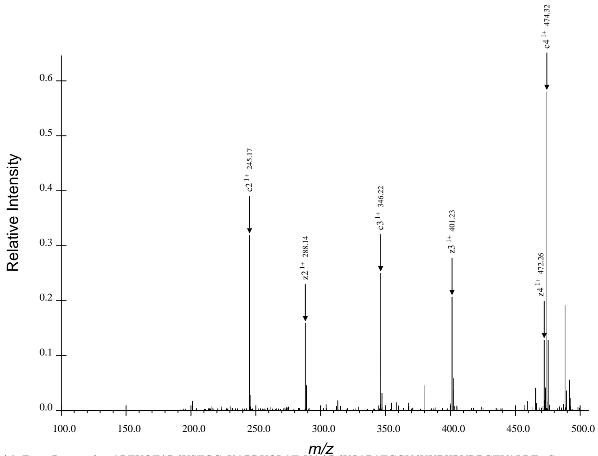
(a) First Region for ARTKQTARdKSTGGaKAPRKQLATaKAARdKSAPATGGVdKKPHRYRPGTVALRE, Spectrum 45.dta
