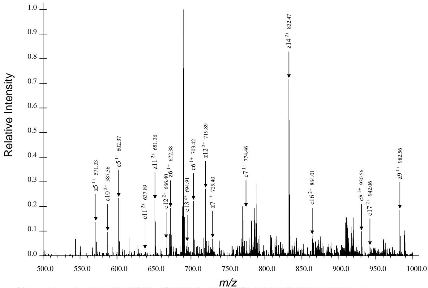
(b) Second Region for ARTKQTARdKSTGGaKAPRKQLATaKAARdKSAPATGGVdKKPHRYRPGTVALRE, Spectrum 15.dta
