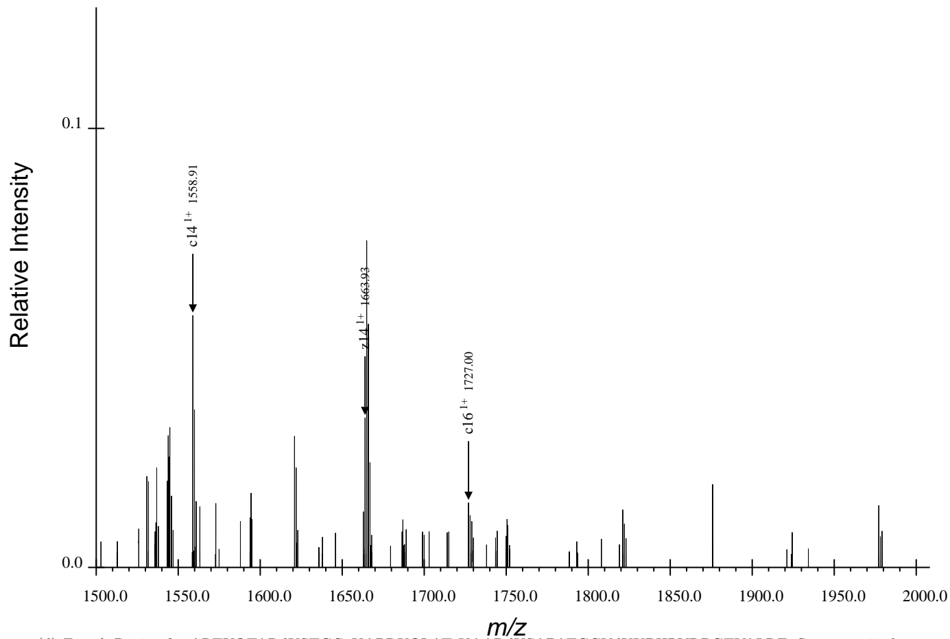
(d) Fourth Region for ARTKQTARdKSTGGaKAPRKQLATaKAARdKSAPATGGVdKKPHRYRPGTVALRE, Spectrum 25.dta
