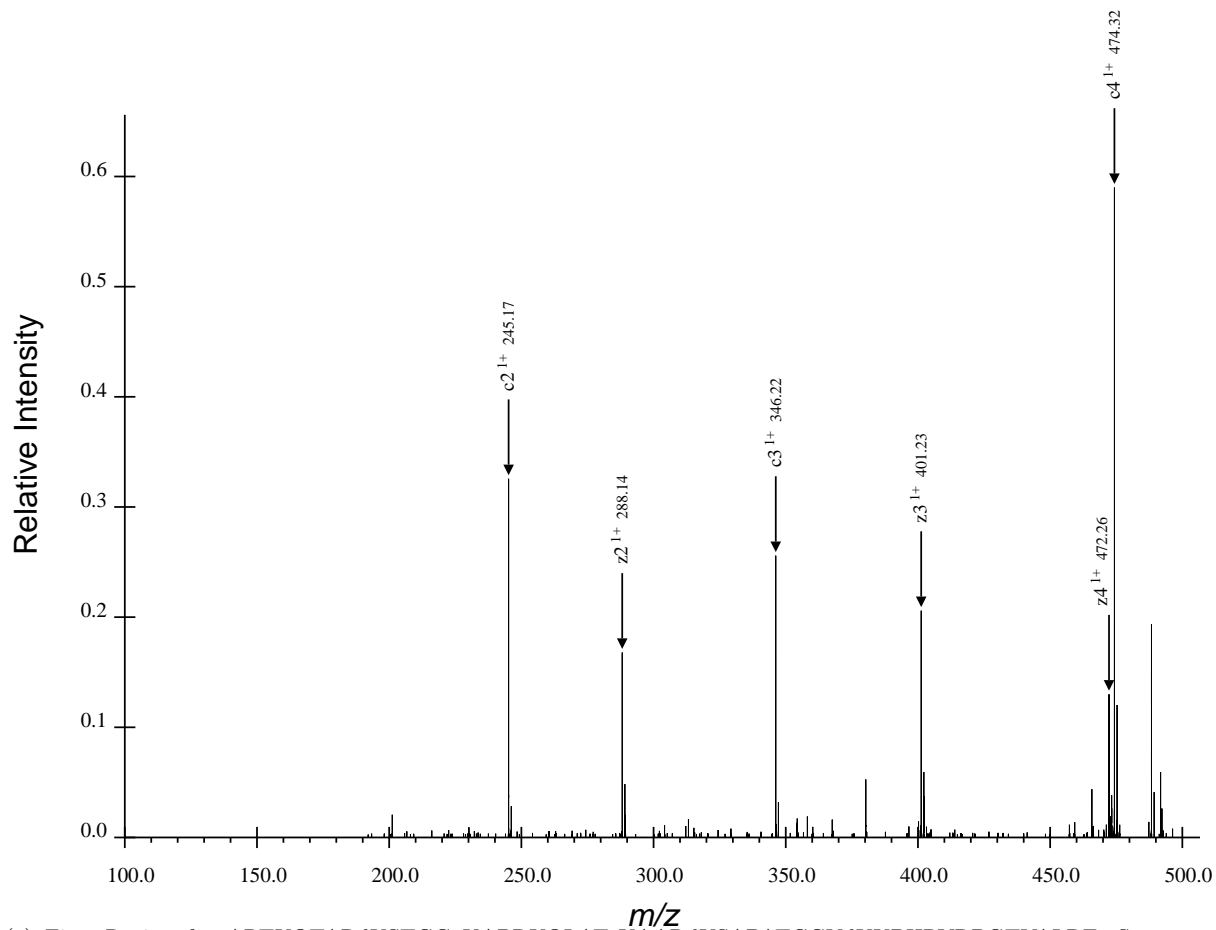
(a) First Region for ARTKQTARdKSTGGaKAPRKQLATaKAARdKSAPATGGVdKKPHRYRPGTVALRE, Spectrum 49.dta
