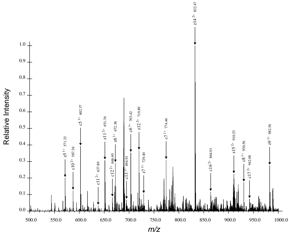
(b) Second Region for ARTKQTARdKSTGGaKAPRKQLATaKAARdKSAPATGGVdKKPHRYRPGTVALRE, Spectrum 31.dta
