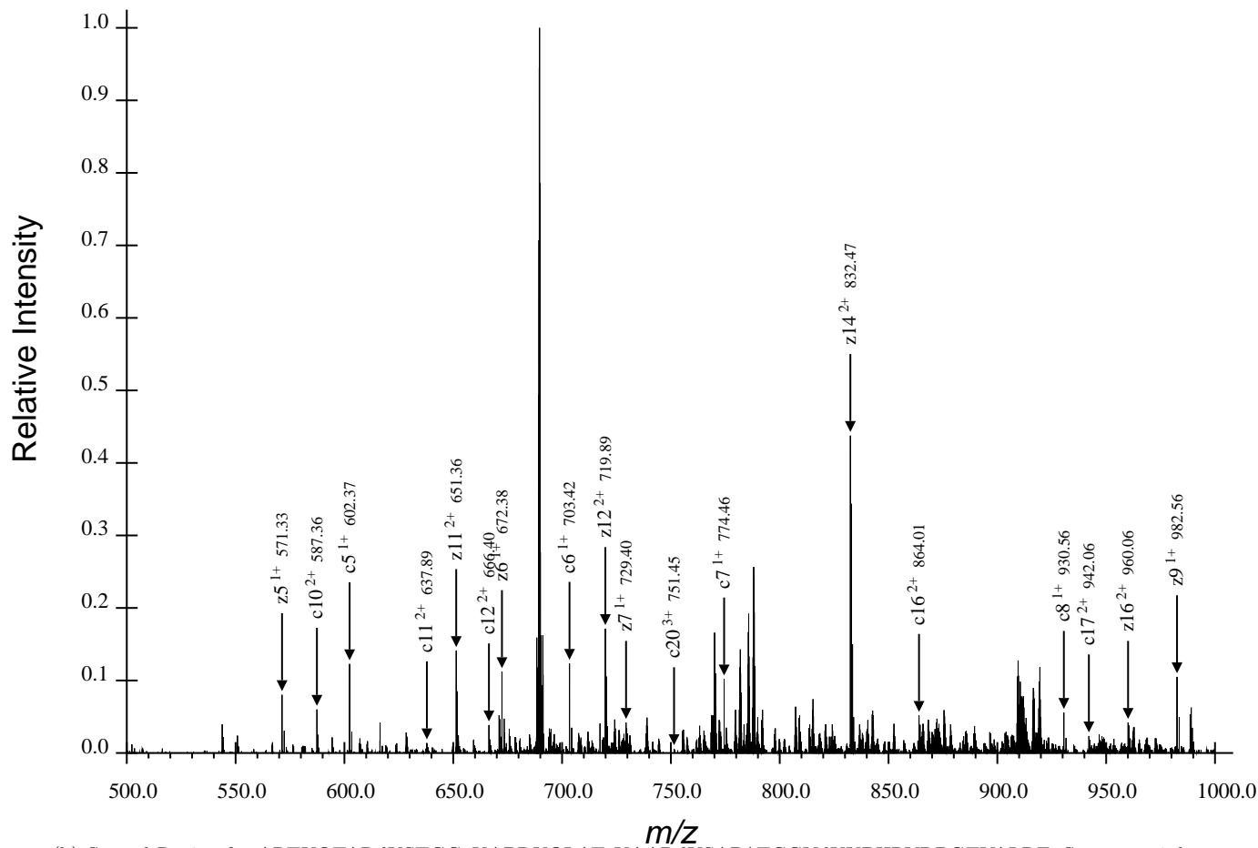
(b) Second Region for ARTKQTARdKSTGGaKAPRKQLATaKAARdKSAPATGGVdKKPHRYRPGTVALRE, Spectrum 6.dta
