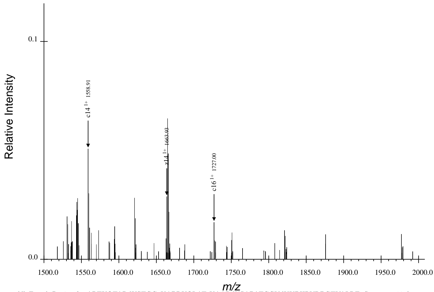
(d) Fourth Region for ARTKQTARdKSTGGaKAPRKQLATaKAARdKSAPATGGVdKKPHRYRPGTVALRE, Spectrum 20.dta
