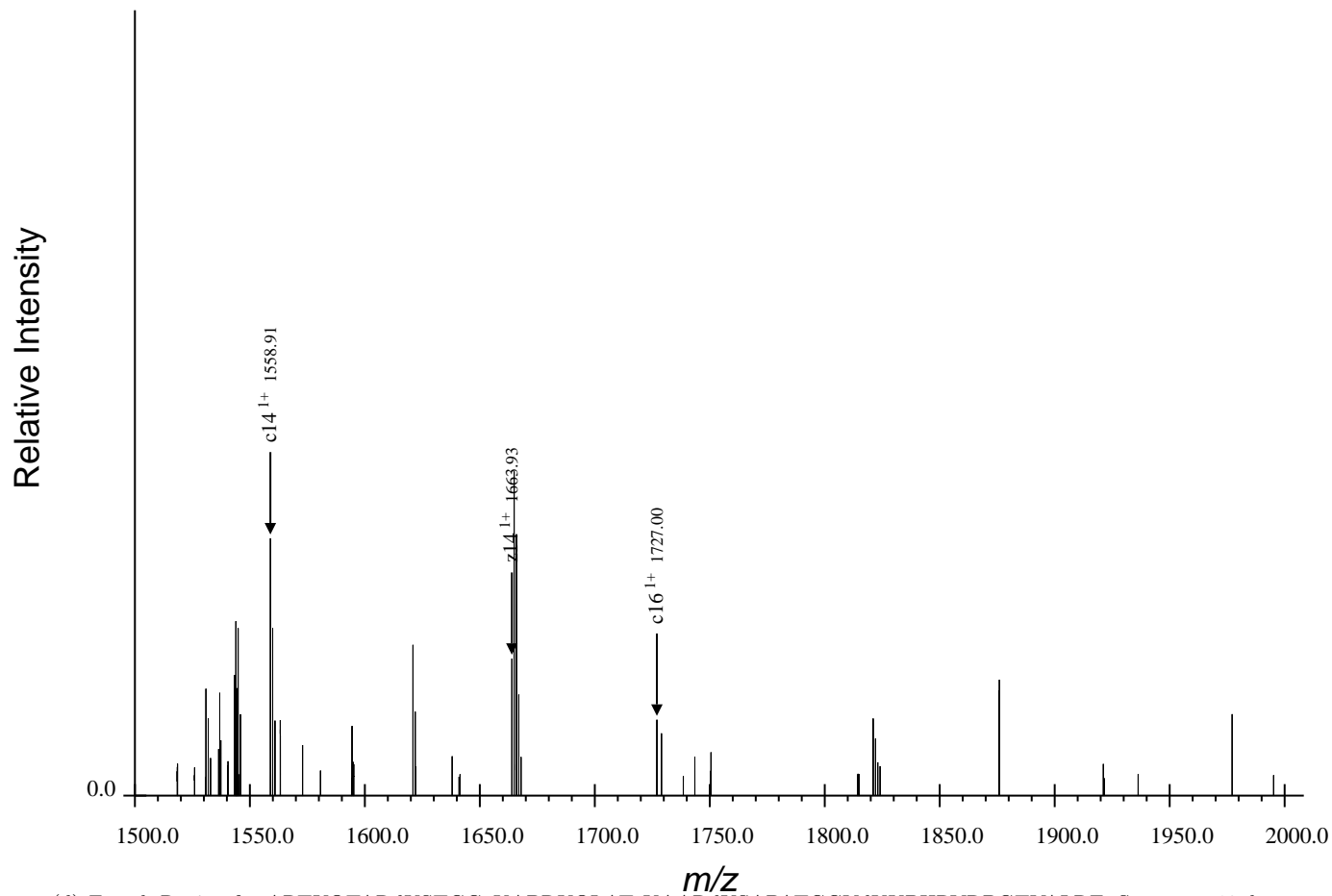
(d) Fourth Region for ARTKQTARdKSTGGaKAPRKQLATaKAARdKSAPATGGVdKKPHRYRPGTVALRE, Spectrum 13.dta
