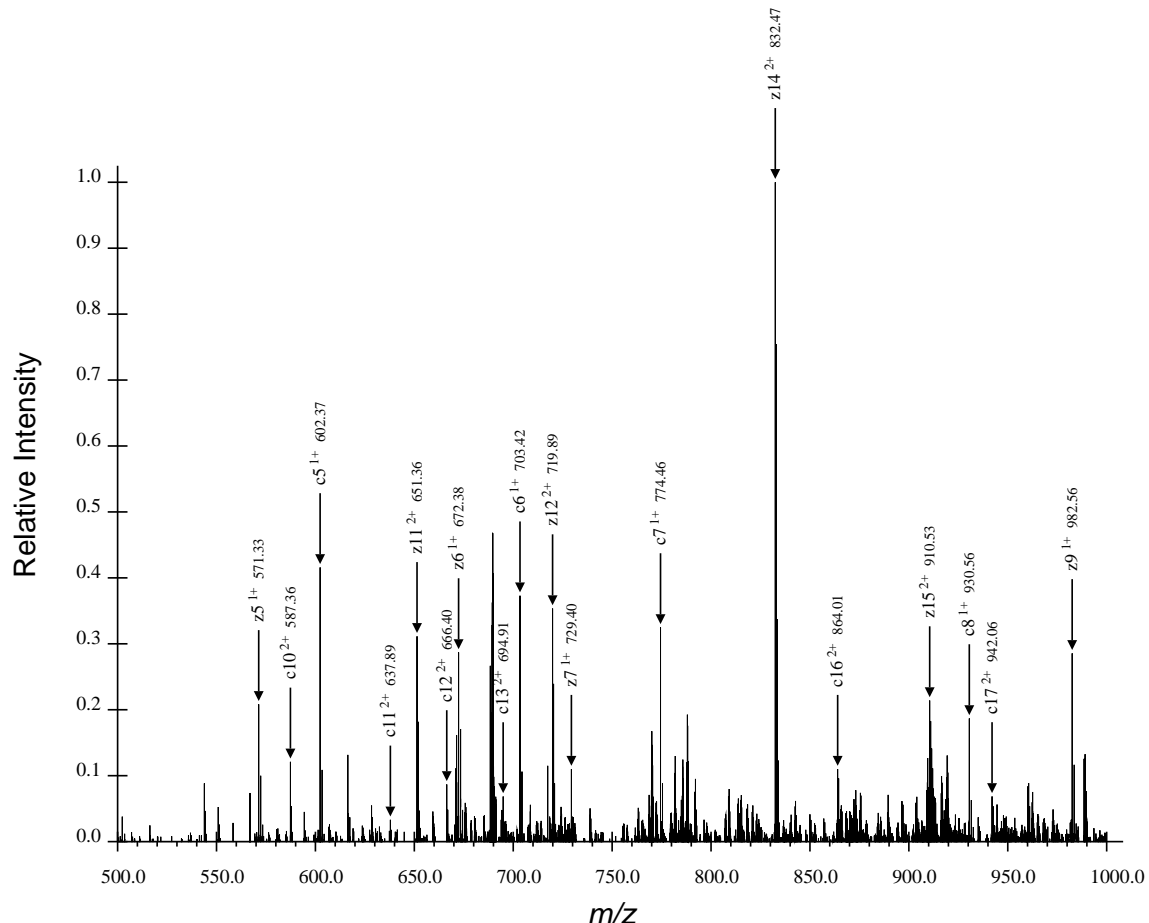
(b) Second Region for ARTKQTARdKSTGGaKAPRKQLATaKAARdKSAPATGGVdKKPHRYRPGTVALRE, Spectrum 53.dta
