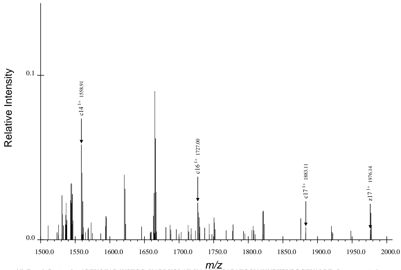
(d) Fourth Region for ARTKQTARdKSTGGaKAPRKQLATaKAARdKSAPATGGVdKKPHRYRPGTVALRE, Spectrum 44.dta
