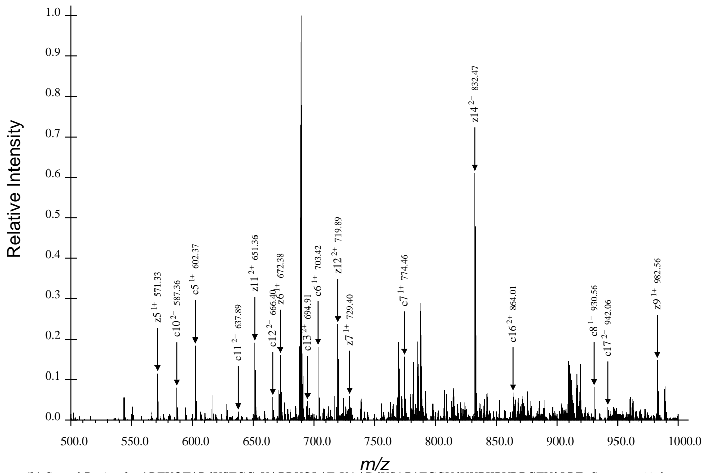
(b) Second Region for ARTKQTARdKSTGGaKAPRKQLATaKAARdKSAPATGGVdKKPHRYRPGTVALRE, Spectrum 12.dta
