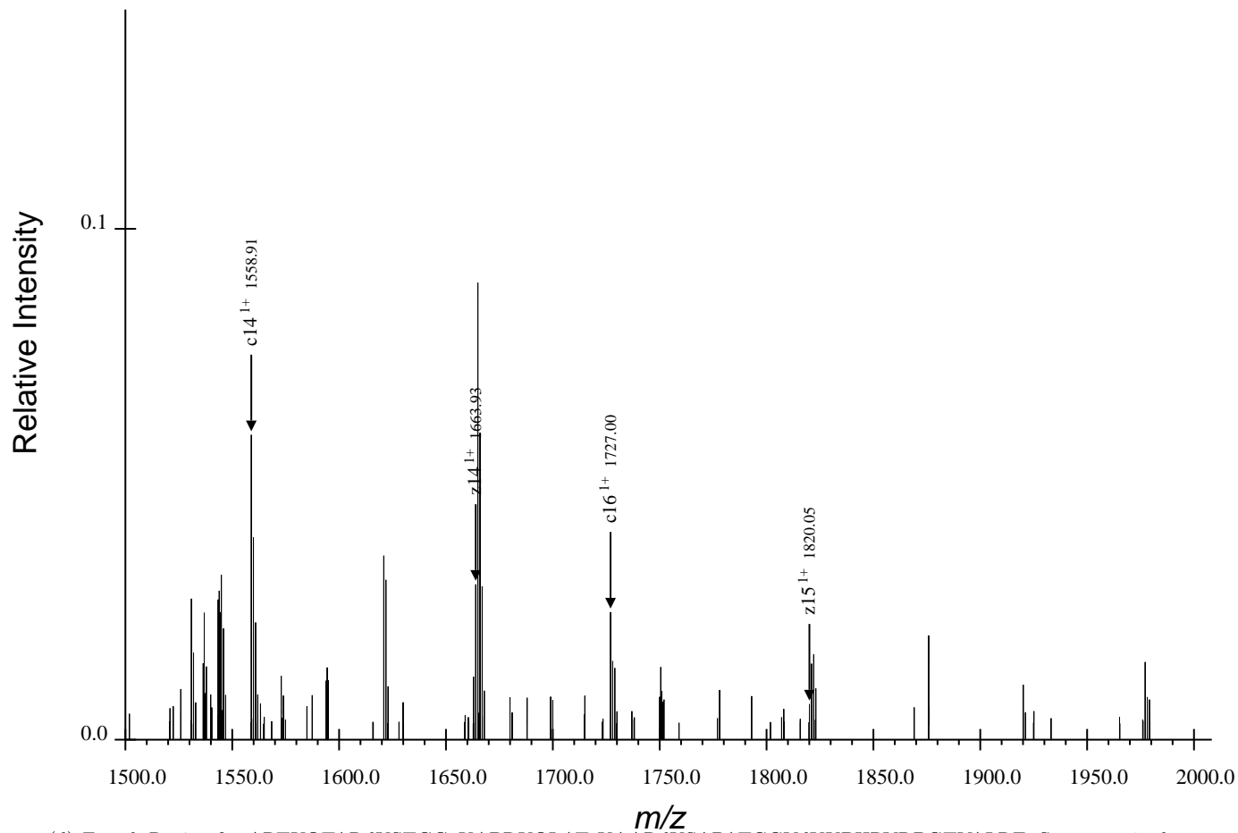
(d) Fourth Region for ARTKQTARdKSTGGaKAPRKQLATaKAARdKSAPATGGVdKKPHRYRPGTVALRE, Spectrum 35.dta
