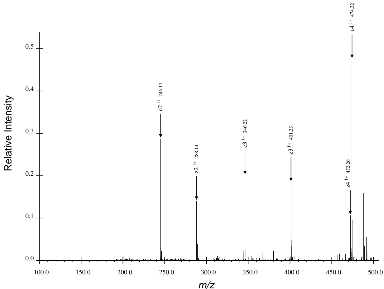
(a) First Region for ARTKQTARdKSTGGaKAPRKQLATaKAARdKSAPATGGVdKKPHRYRPGTVALRE, Spectrum 19.dta
