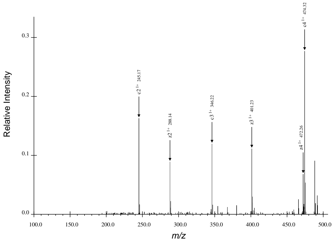
(a) First Region for ARTKQTARdKSTGGaKAPRKQLATaKAARdKSAPATGGVdKKPHRYRPGTVALRE, Spectrum 11.dta
