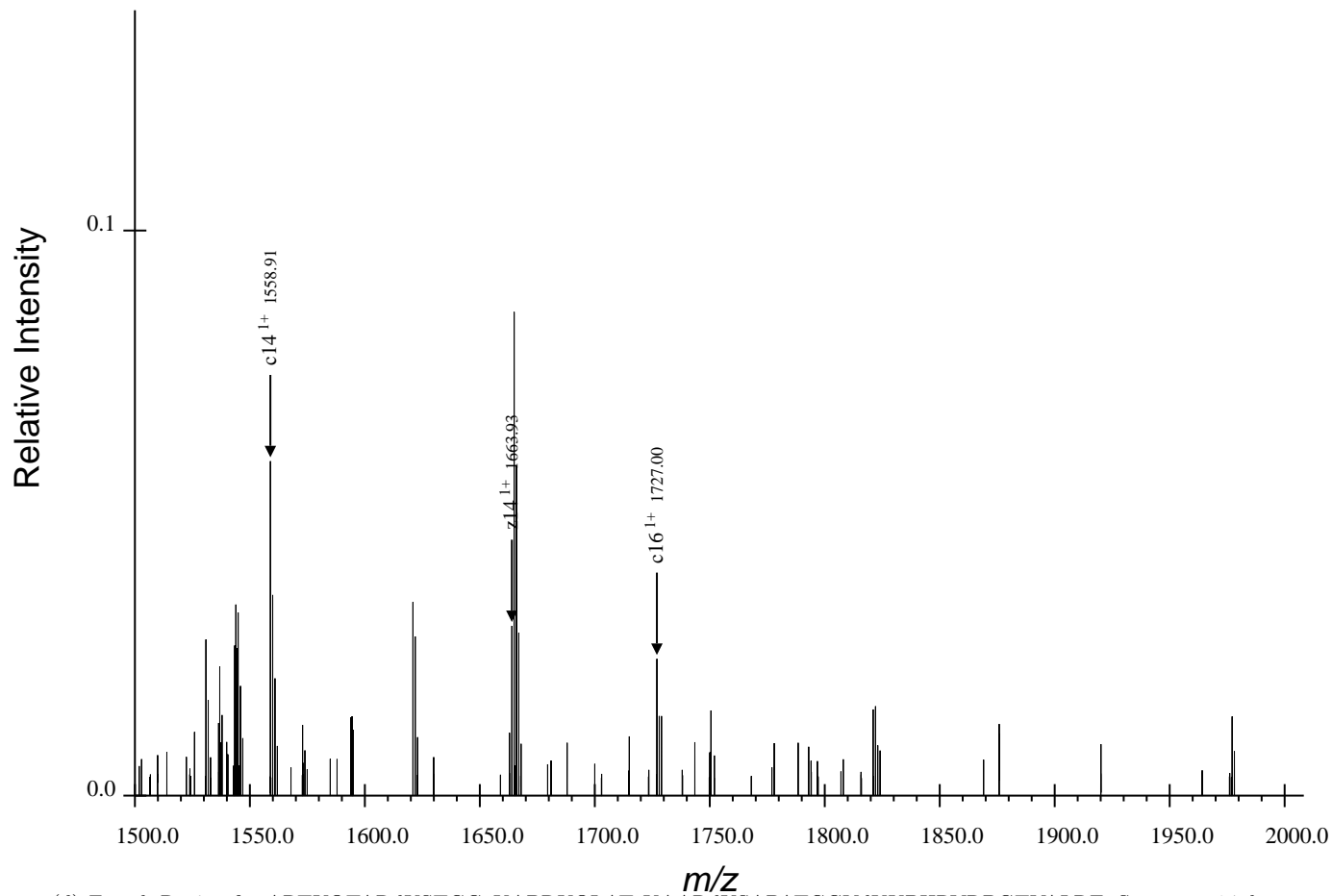
(d) Fourth Region for ARTKQTARdKSTGGaKAPRKQLATaKAARdKSAPATGGVdKKPHRYRPGTVALRE, Spectrum 34.dta
