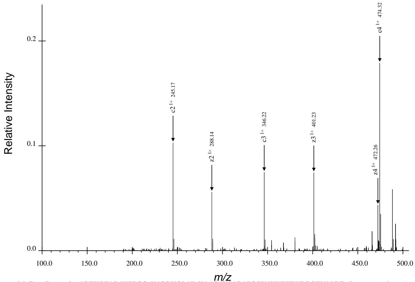
(a) First Region for ARTKQTARdKSTGGaKAPRKQLATaKAARdKSAPATGGVdKKPHRYRPGTVALRE, Spectrum 2.dta
