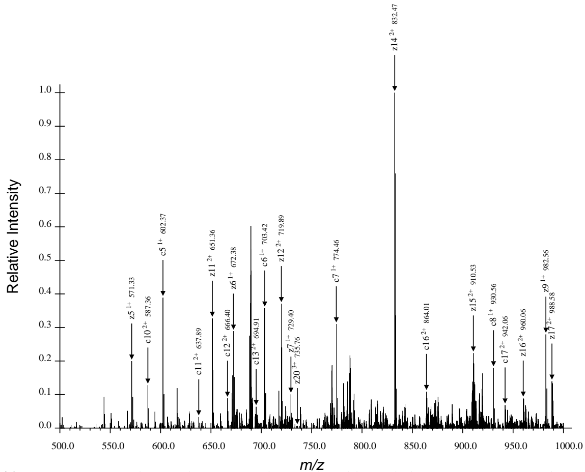
(b) Second Region for ARTKQTARdKSTGGaKAPRKQLATaKAARdKSAPATGGVdKKPHRYRPGTVALRE, Spectrum 37.dta
