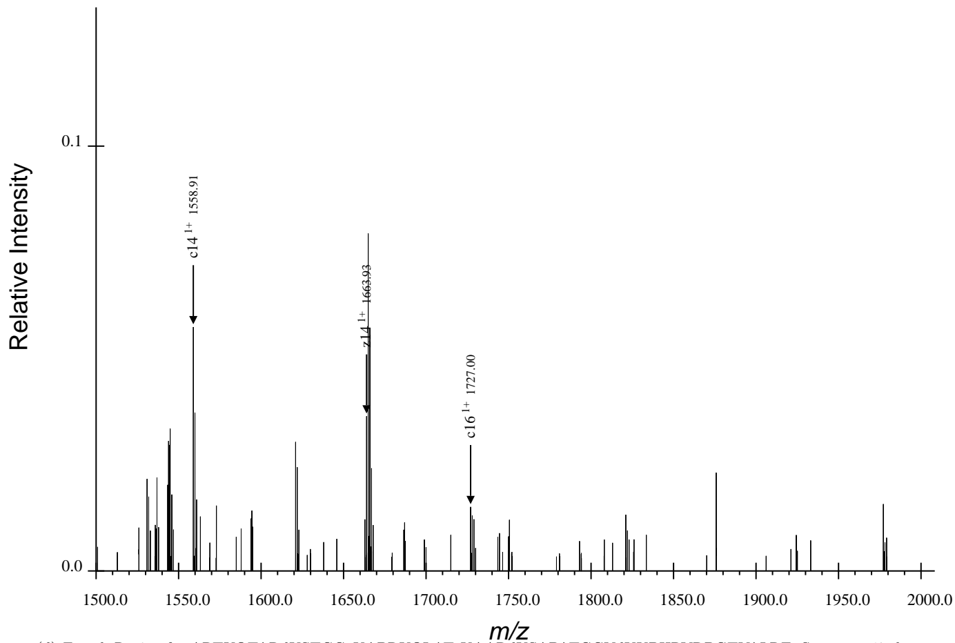
(d) Fourth Region for ARTKQTARdKSTGGaKAPRKQLATaKAARdKSAPATGGVdKKPHRYRPGTVALRE, Spectrum 27.dta
