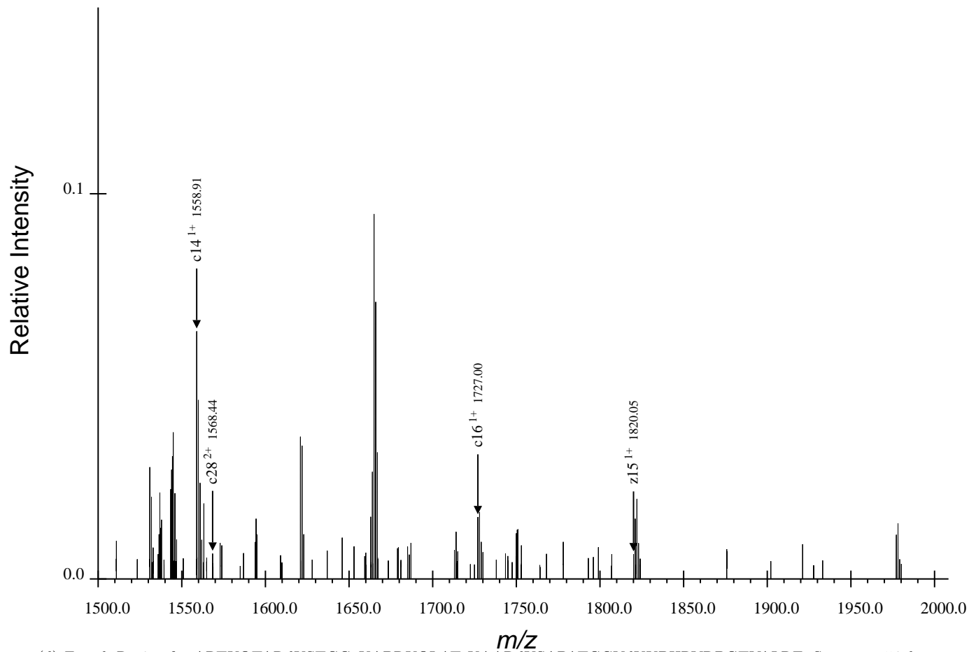
(d) Fourth Region for ARTKQTARdKSTGGaKAPRKQLATaKAARdKSAPATGGVdKKPHRYRPGTVALRE, Spectrum 54.dta
