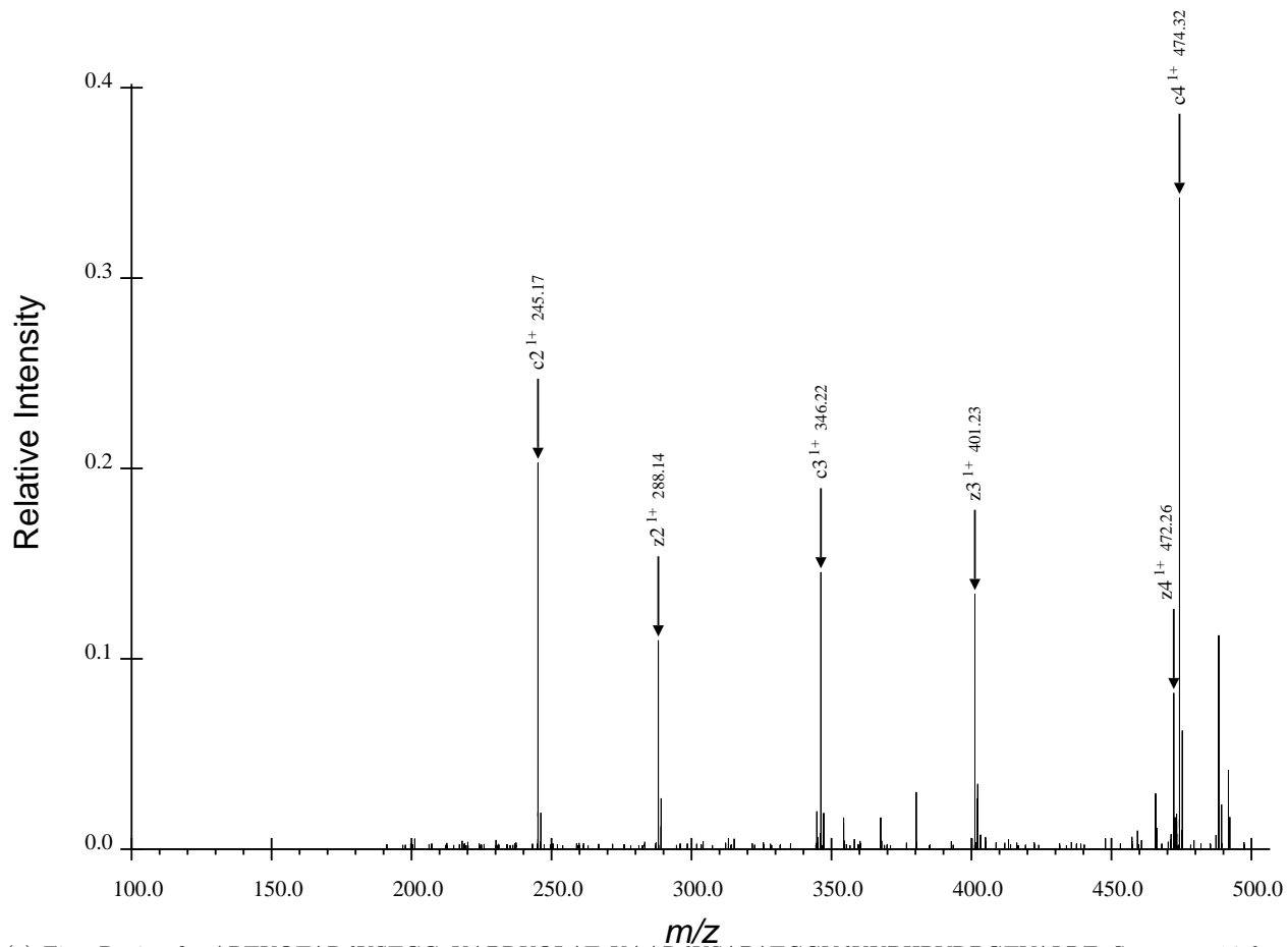
(a) First Region for ARTKQTARdKSTGGaKAPRKQLATaKAARdKSAPATGGVdKKPHRYRPGTVALRE, Spectrum 14.dta
