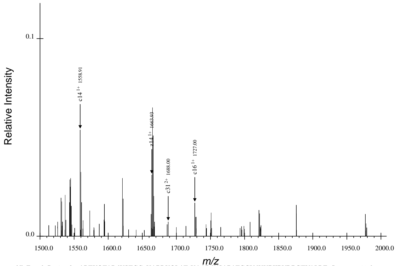
(d) Fourth Region for ARTKQTARdKSTGGaKAPRKQLATaKAARdKSAPATGGVdKKPHRYRPGTVALRE, Spectrum 21.dta
