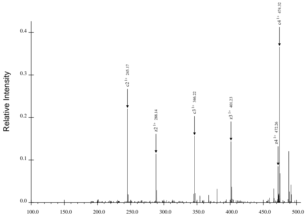
(a) First Region for ARTKQTARdKSTGGaKAPRKQLATaKAARdKSAPATGGVdKKPHRYRPGTVALRE, Spectrum 15.dta
