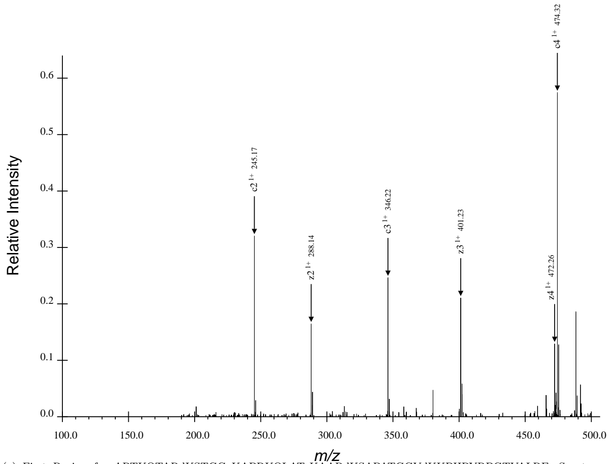
(a) First Region for ARTKQTARdKSTGGaKAPRKQLATaKAARdKSAPATGGVdKKPHRYRPGTVALRE, Spectrum 43.dta
