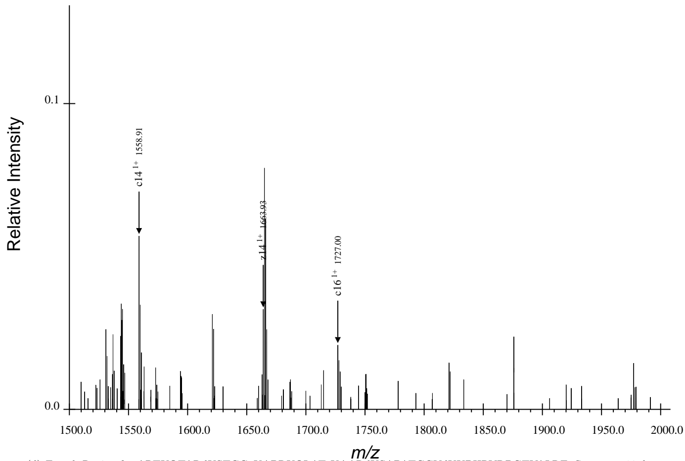
(d) Fourth Region for ARTKQTARdKSTGGaKAPRKQLATaKAARdKSAPATGGVdKKPHRYRPGTVALRE, Spectrum 30.dta
