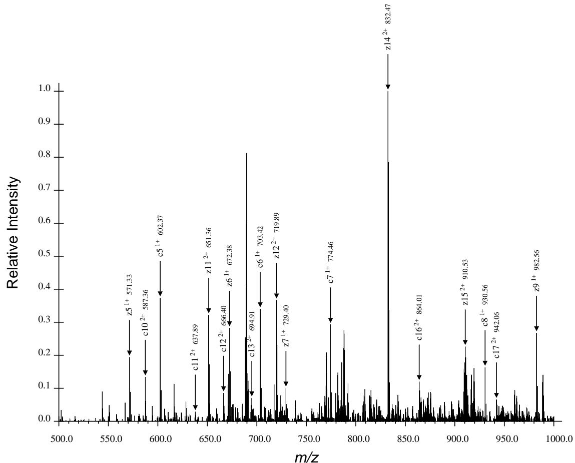
(b) Second Region for ARTKQTARdKSTGGaKAPRKQLATaKAARdKSAPATGGVdKKPHRYRPGTVALRE, Spectrum 26.dta
