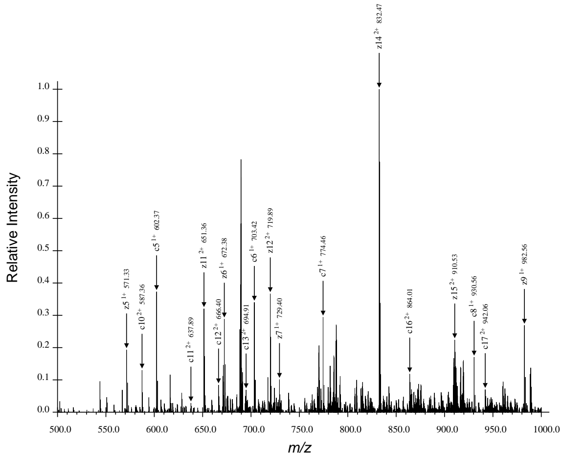
(b) Second Region for ARTKQTARdKSTGGaKAPRKQLATaKAARdKSAPATGGVdKKPHRYRPGTVALRE, Spectrum 27.dta
