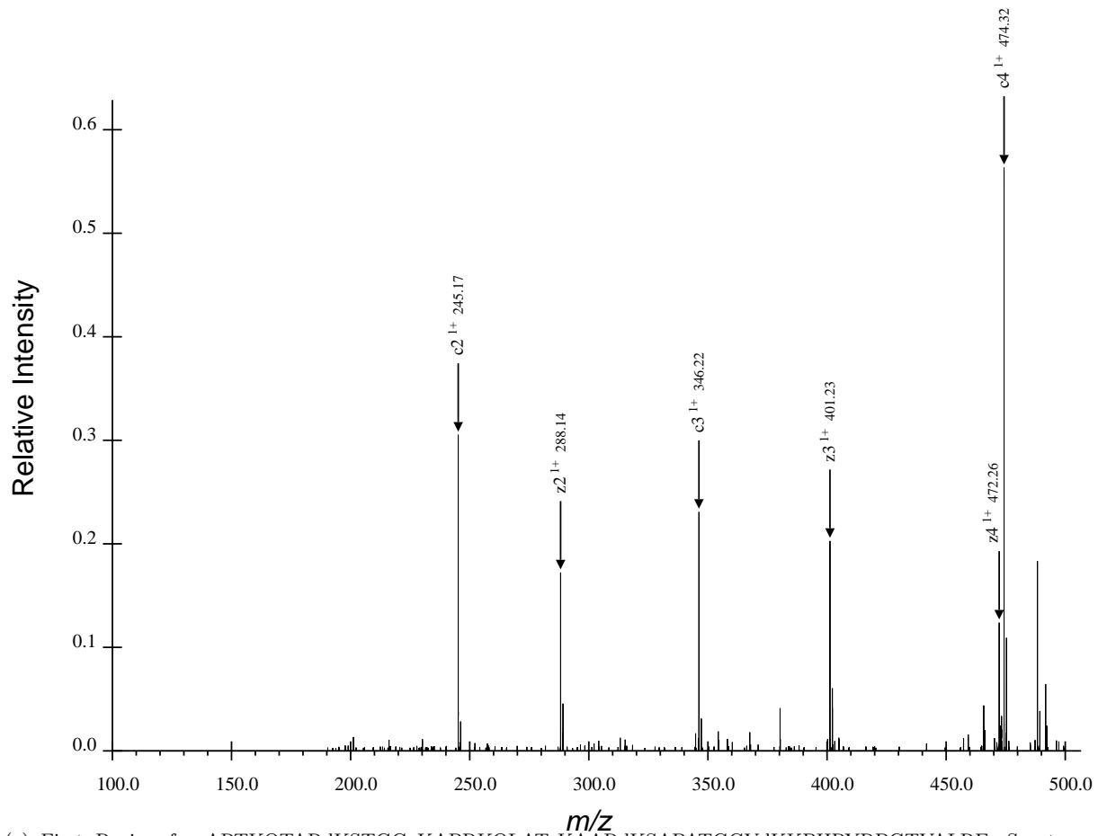
(a) First Region for ARTKQTARdKSTGGaKAPRKQLATaKAARdKSAPATGGVdKKPHRYRPGTVALRE, Spectrum 26.dta
