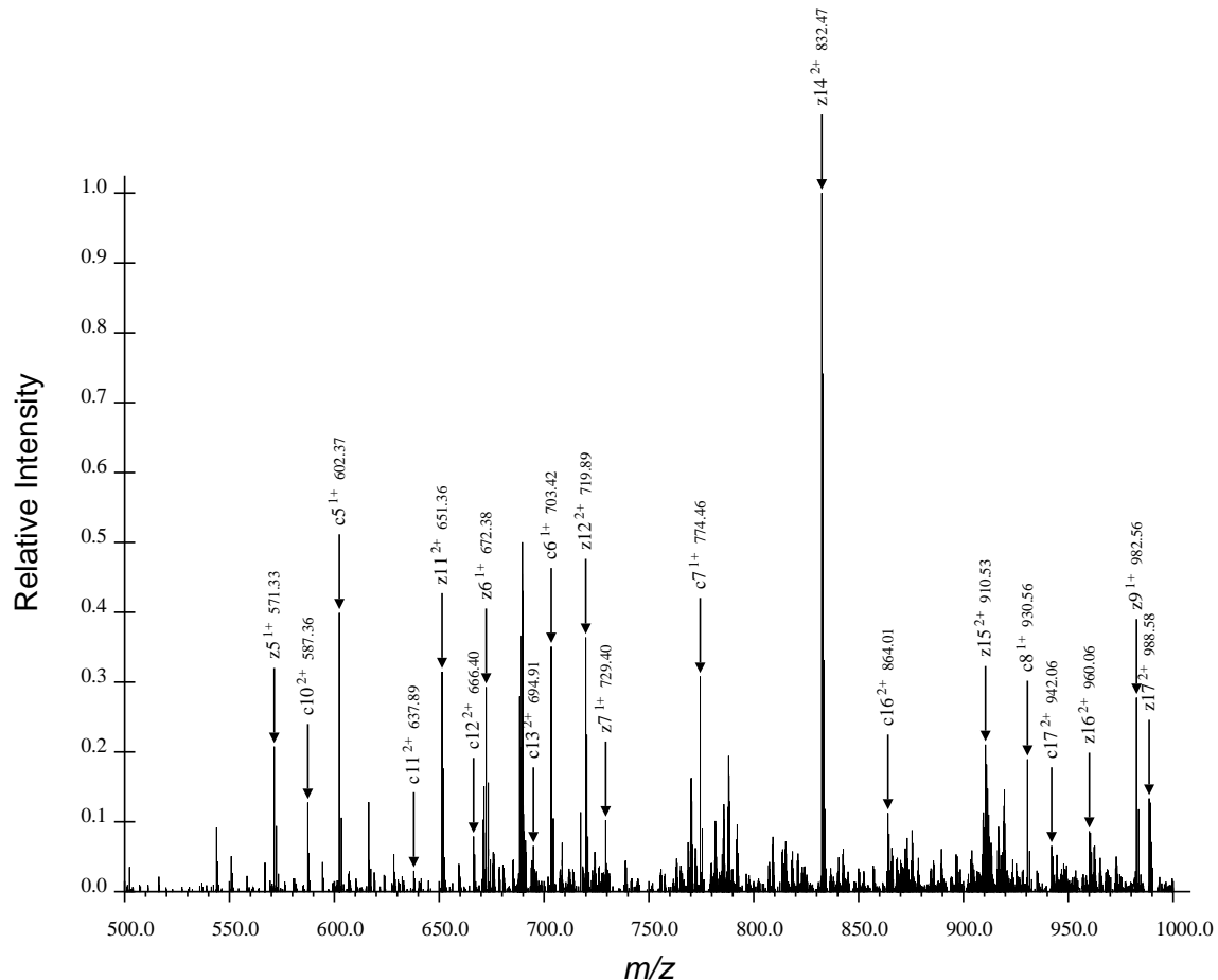
(b) Second Region for ARTKQTARdKSTGGaKAPRKQLATaKAARdKSAPATGGVdKKPHRYRPGTVALRE, Spectrum 47.dta
