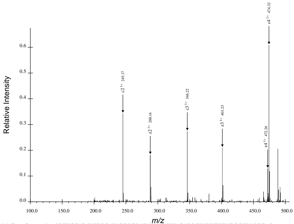
(a) First Region for ARTKQTARdKSTGGaKAPRKQLATaKAARdKSAPATGGVdKKPHRYRPGTVALRE, Spectrum 56.dta
