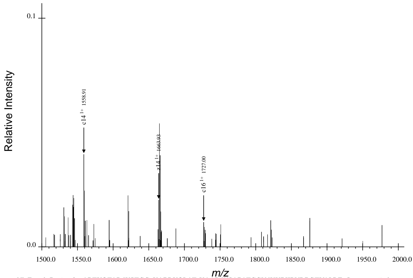
(d) Fourth Region for ARTKQTARdKSTGGaKAPRKQLATaKAARdKSAPATGGVdKKPHRYRPGTVALRE, Spectrum 17.dta
