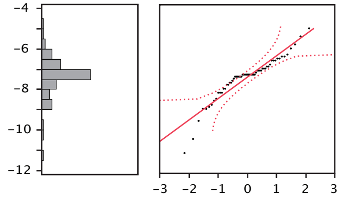
E) \delta^{13}\text{C}
