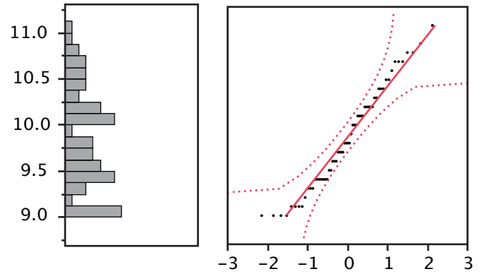
F) \delta^{15}\text{N}
