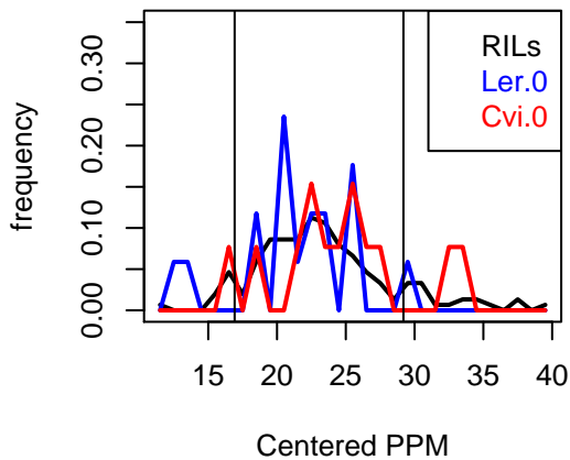
Co59
