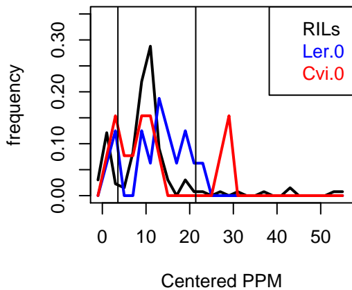
Ni60
