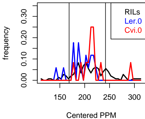
Fe56
