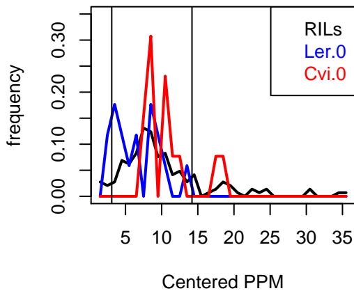
Cu65
