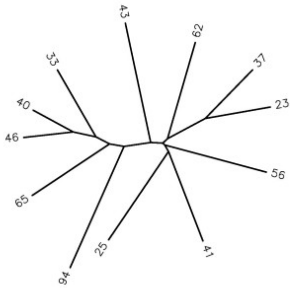
Group 1 : S2
