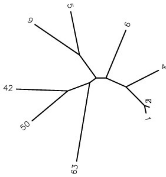
Group 2 : S1
