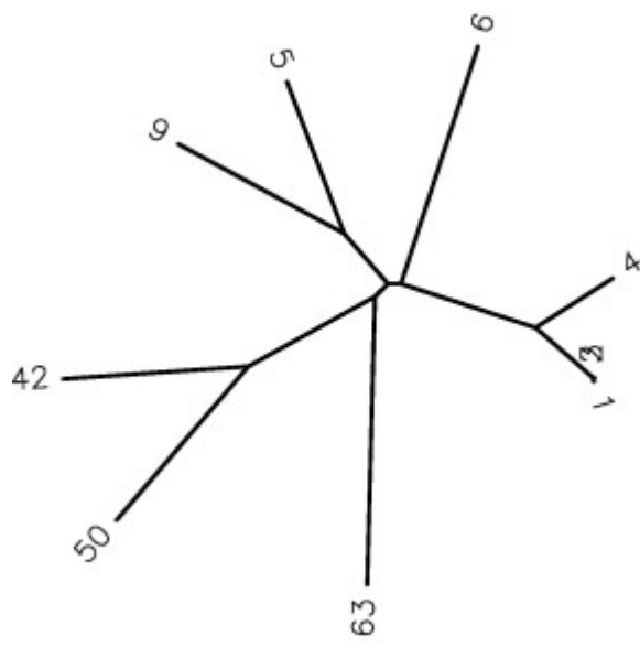
Group 2 : S2
