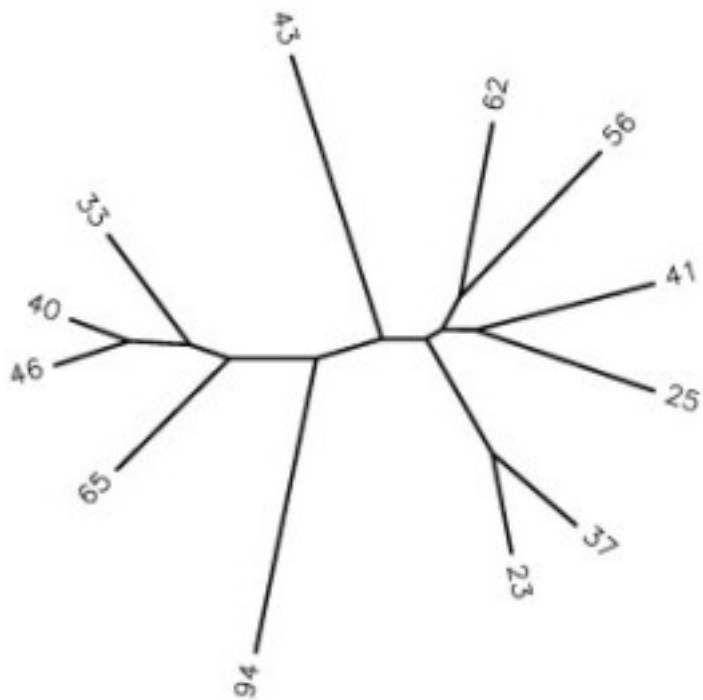
Group 1 : S2
