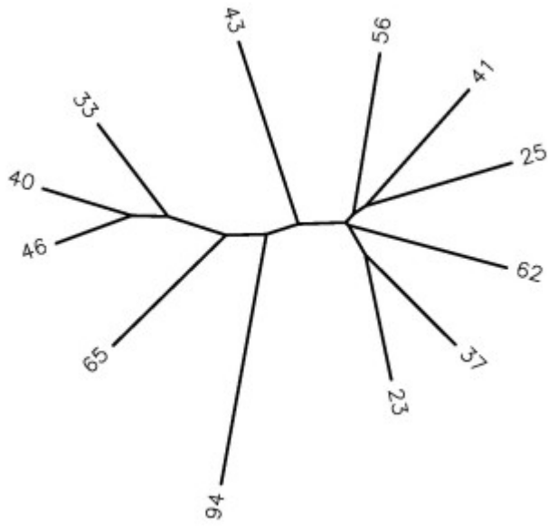
Group 1 : S1
