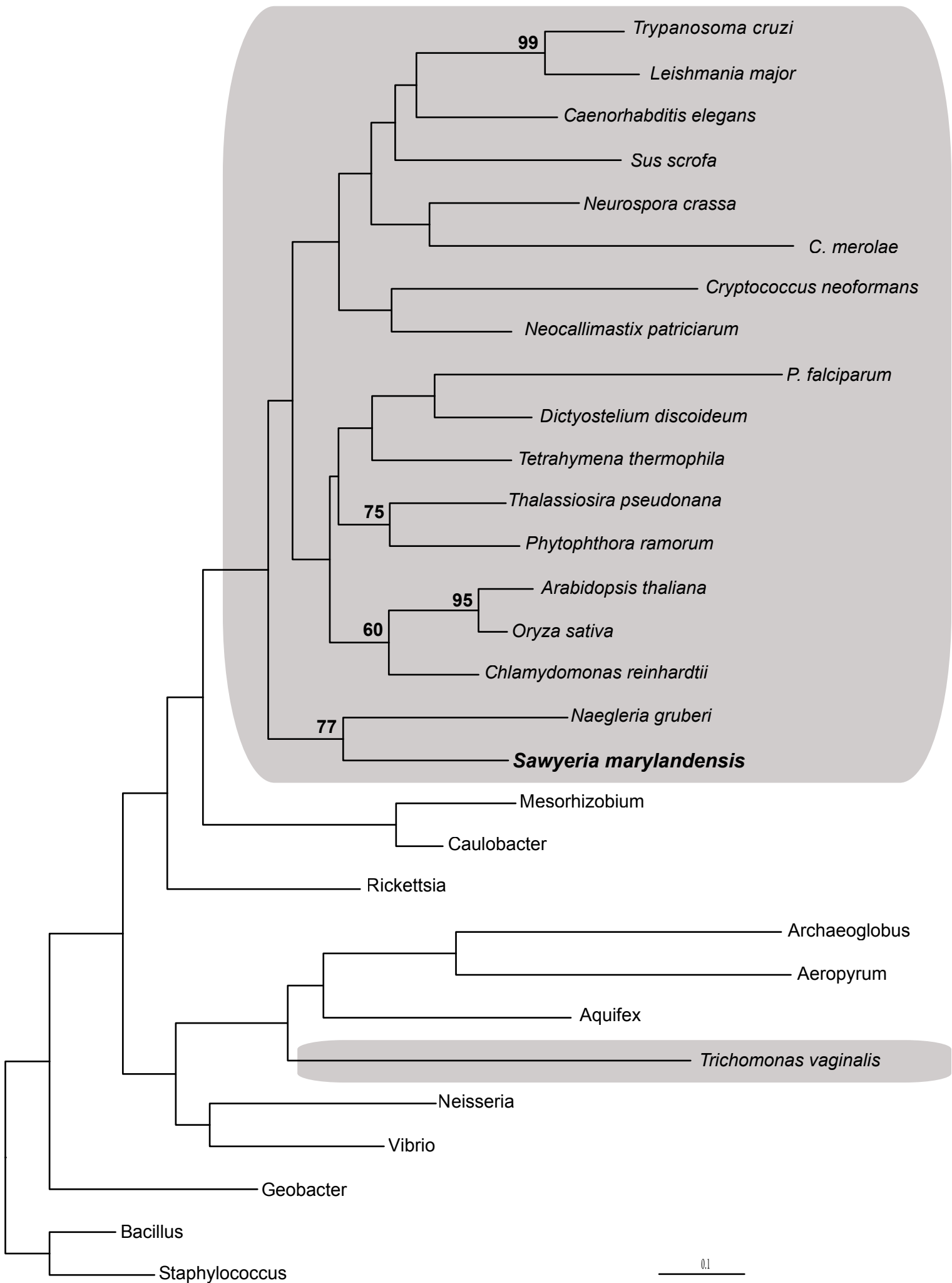
Fig. S1-SCSalpha ML tree
