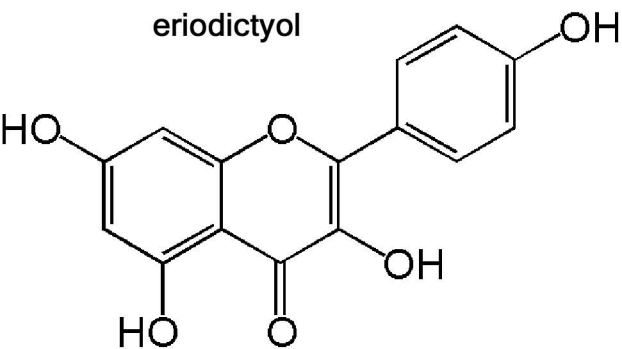
kaempferol
