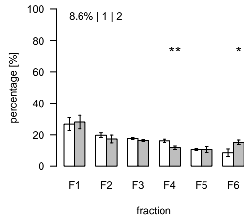
L1675 (m/z=253.200643; rt=8.70638) T/S Cluster: L-8.7-5
