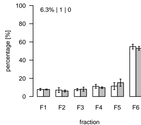
L1385 (m/z=924.497716; rt=7.57355) T/S Cluster: L-7.6-1
