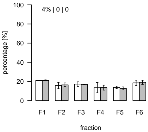
L2158 (m/z=421.336095; rt=10.61354) T/S Cluster: L-10.6-4
