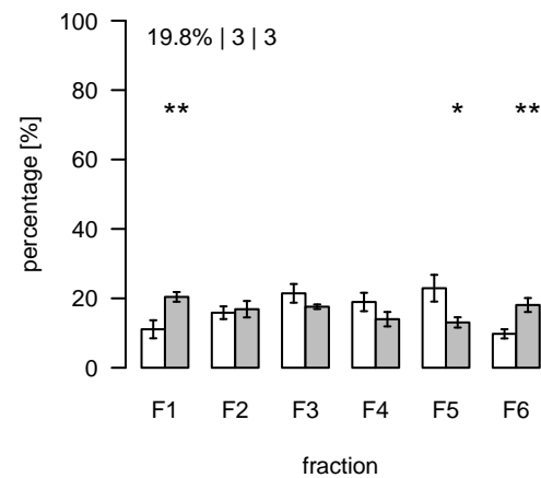
L2274 (m/z=1412.996974; rt=11.32776) T/S Cluster: L-11.3-2
