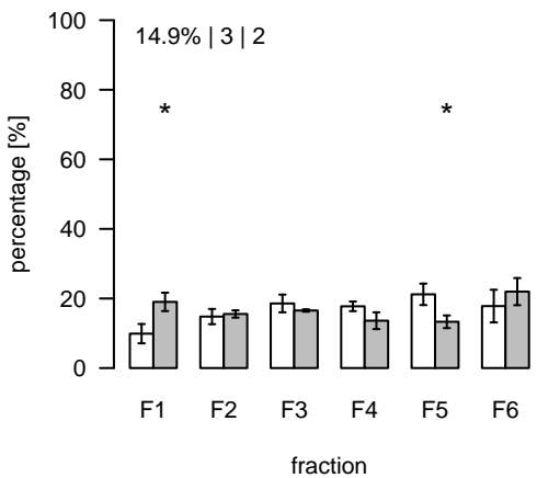
L2263 (m/z=136.097301; rt=11.32771) T/S Cluster: L-11.3-4
