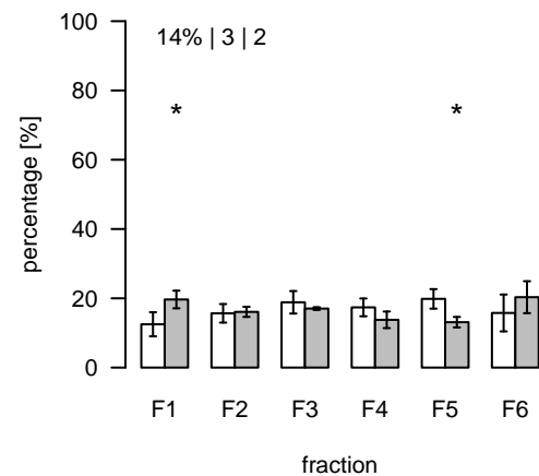
L2249 (m/z=221.489556; rt=11.32731) T/S Cluster: L-11.3-4
