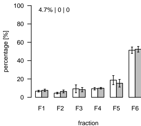
L2036 (m/z=925.494526; rt=10.21264) T/S Cluster: L-10.2-2
