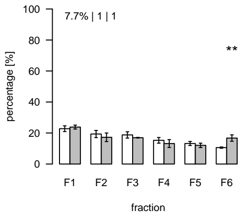
L2685 (m/z=924.862333; rt=16.0421) T/S Cluster: L-16-2
