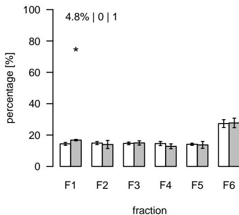
L2107 (m/z=447.77271; rt=10.50484) T/S Cluster: L-10.5-13
