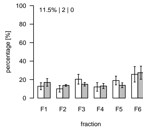
L2004 (m/z=885.556269; rt=10.09039) T/S Cluster: L-10.1-6
