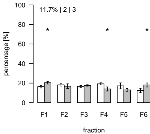
L2385 (m/z=1056.756066; rt=11.3302) T/S Cluster: L-11.3-35
