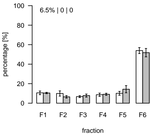
L76 (m/z=814.525245; rt=3.46649) T/S Cluster: L-3.5-2
