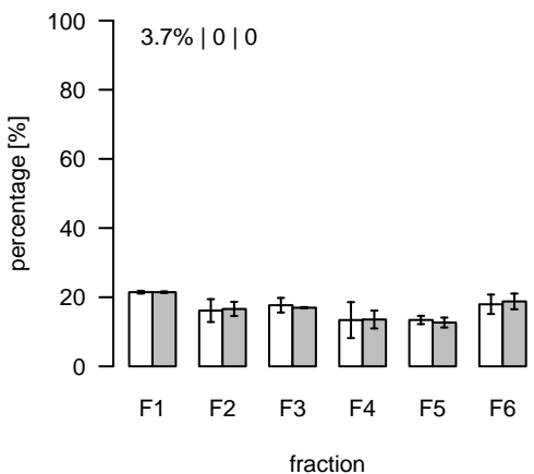
L2156 (m/z=842.677186; rt=10.61318) T/S Cluster: L-10.6-4
