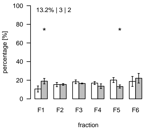
L2292 (m/z=226.830657; rt=11.32795) T/S Cluster: L-11.3-4
