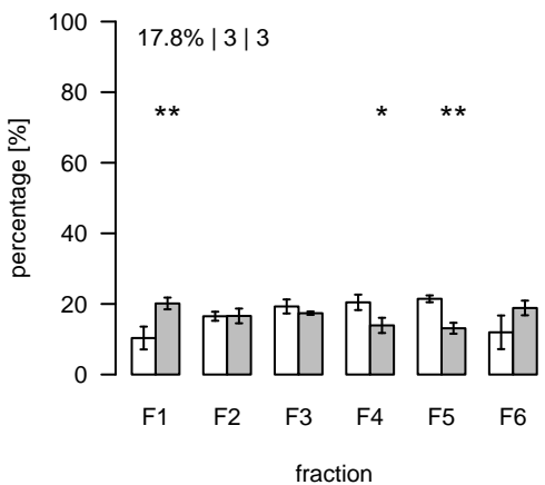
L2366 (m/z=1363.871541; rt=11.32867) T/S Cluster: L-11.3-2
