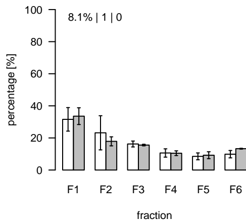
L730 (m/z=826.518435; rt=5.28653) T/S Cluster: L-5.3-2
