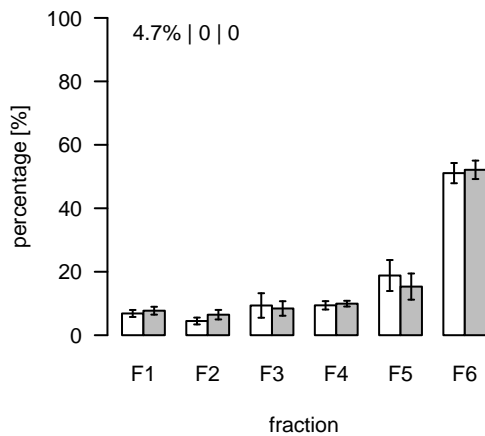
L2032 (m/z=927.509817; rt=10.21243) T/S Cluster: L-10.2-2
