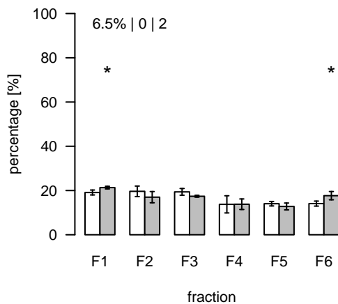
L2418 (m/z=867.676689; rt=11.72504) T/S Cluster: L-11.7-1
