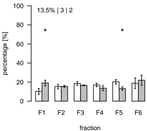
L2262 (m/z=227.162009; rt=11.32769) T/S Cluster: L-11.3-4
