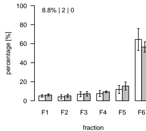
L37 (m/z=848.508507; rt=3.2258) T/S Cluster: L-3.2-1
