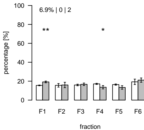
L2373 (m/z=1050.797211; rt=11.32884) T/S Cluster: L-11.3-30
