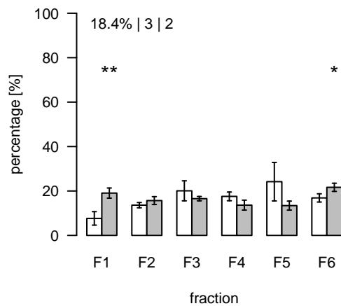
L2411 (m/z=681.486847; rt=11.58174) T/S Cluster: L-11.6-1
