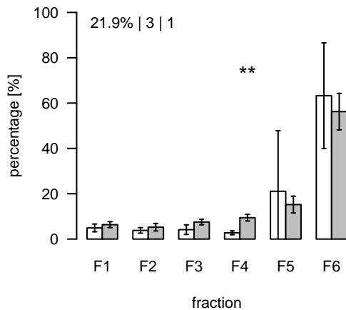
L2228 (m/z=904.570561; rt=11.23078) T/S Cluster: L-11.2-2
