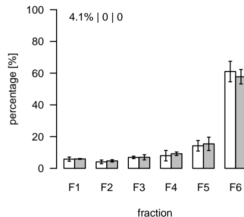
L546 (m/z=389.258146; rt=4.83539) T/S Cluster: L-4.8-10
