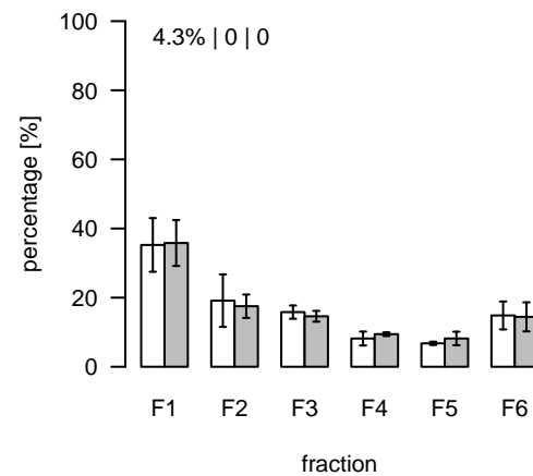
S322 (m/z=299.150847; rt=10.06144) T/S Cluster: S-10.1-1
