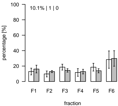
L2000 (m/z=886.559732; rt=10.09015) T/S Cluster: L-10.1-6
