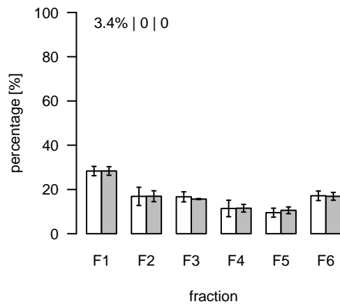
L1258 (m/z=244.191717; rt=7.16393) T/S Cluster: L-7.2-1
