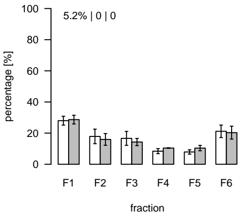
L737 (m/z=825.549221; rt=5.29179) T/S Cluster: L-5.3-3
