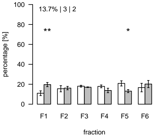
L2387 (m/z=1213.08701; rt=11.33755) T/S Cluster: L-11.3-37
