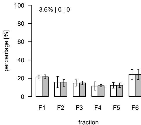
L285 (m/z=651.447207; rt=4.09576) T/S Cluster: L-4.1-2
