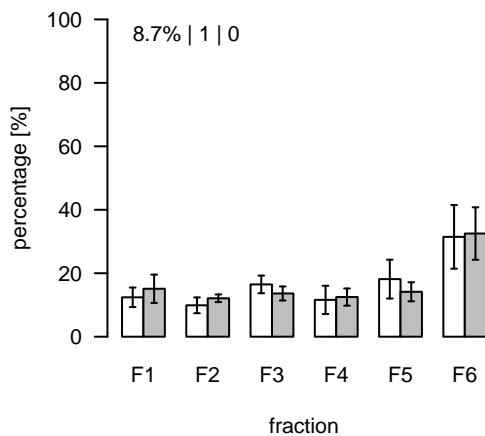
L2019 (m/z=874.531562; rt=10.11931) T/S Cluster: L-10.1-6
