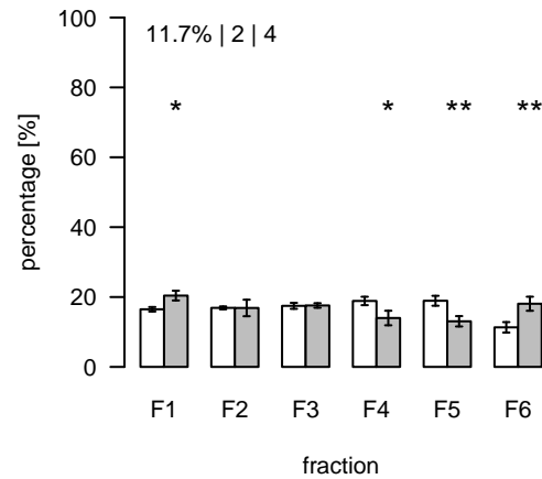
L2386 (m/z=1055.752726; rt=11.33073) T/S Cluster: L-11.3-36
