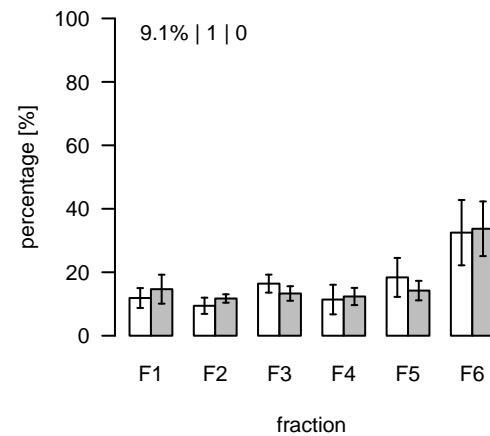
L2020 (m/z=874.562071; rt=10.11935) T/S Cluster: L-10.1-6
