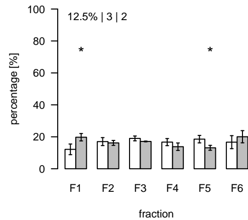
L2284 (m/z=665.448976; rt=11.32786) T/S Cluster: L-11.3-4
