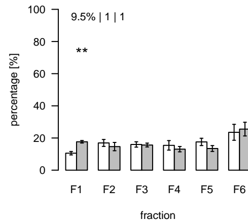
L2743 (m/z=565.162984; rt=16.54648) T/S Cluster: L-16.5-6
