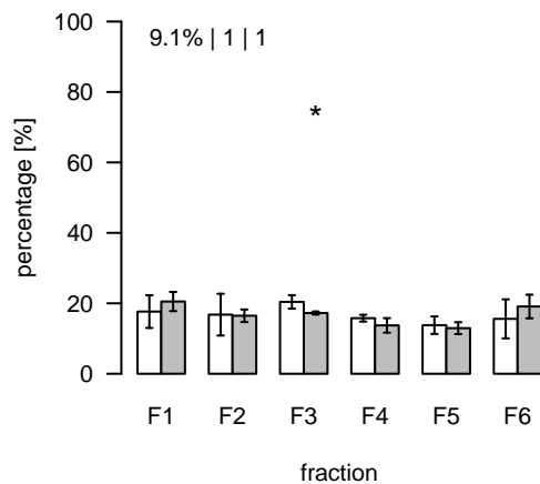
L1993 (m/z=907.574614; rt=10.08396) T/S Cluster: L-10.1-5
