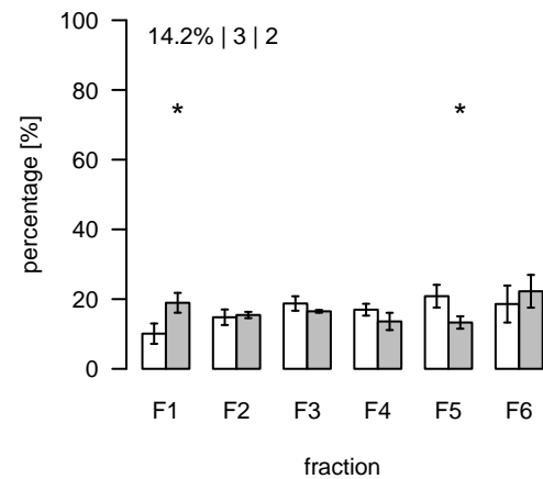
L2245 (m/z=227.499745; rt=11.32719) T/S Cluster: L-11.3-4
