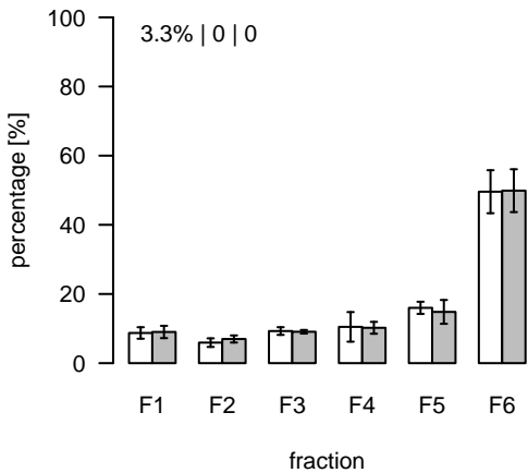
L1463 (m/z=384.283293; rt=7.91847) T/S Cluster: L-7.9-9
