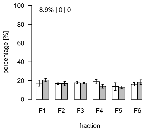
L1801 (m/z=437.748343; rt=8.91949) T/S Cluster: L-8.9-15
