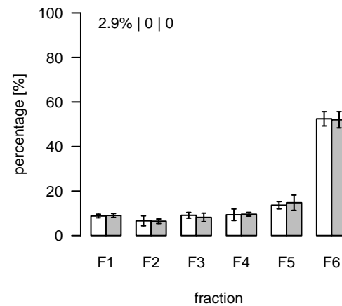
L940 (m/z=389.135681; rt=6.12859) T/S Cluster: L-6.1-1
