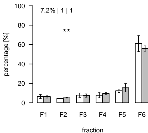
L2067 (m/z=889.565099; rt=10.39685) T/S Cluster: L-10.4-1
