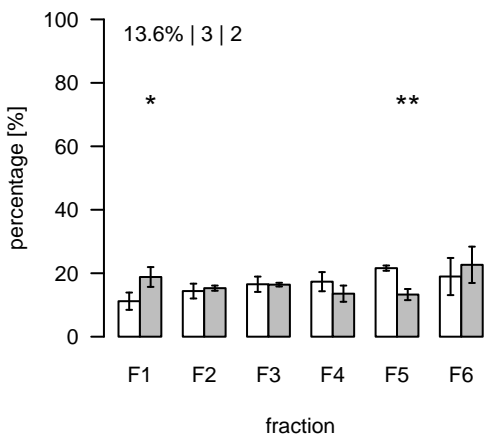
L2368 (m/z=1386.973574; rt=11.32872) T/S Cluster: L-11.3-23
