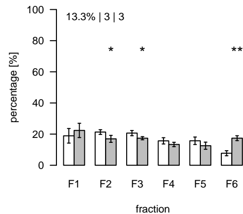
L2327 (m/z=1371.976616; rt=11.32836) T/S Cluster: L-11.3-17
