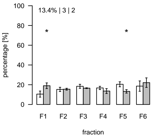
L2261 (m/z=341.248093; rt=11.32769) T/S Cluster: L-11.3-4
