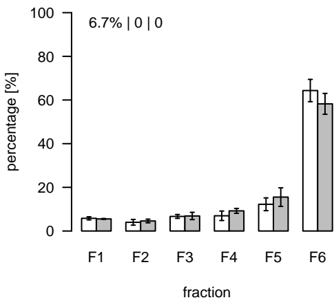
L776 (m/z=806.508493; rt=5.36257) T/S Cluster: L-5.4-2
