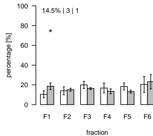
L2416 (m/z=663.457354; rt=11.59843) T/S Cluster: L-11.6-1
