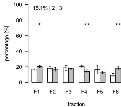
L2238 (m/z=231.116613; rt=11.32021) T/S Cluster: L-11.3-7
