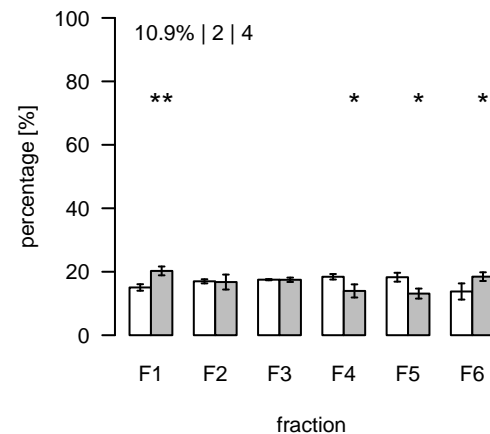
L2334 (m/z=686.444243; rt=11.3284) T/S Cluster: L-11.3-15
