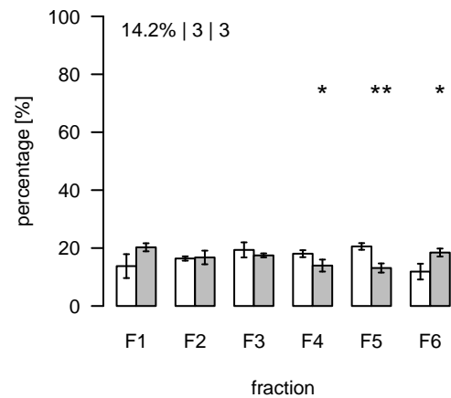
L2332 (m/z=1412.007156; rt=11.32839) T/S Cluster: L-11.3-4
