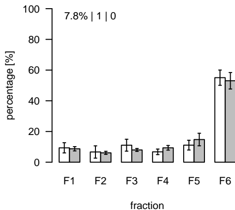
L2053 (m/z=885.557761; rt=10.33861) T/S Cluster: L-10.3-2
