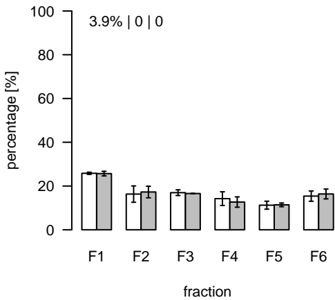
L686 (m/z=804.547664; rt=5.07773) T/S Cluster: L-5.1-3
