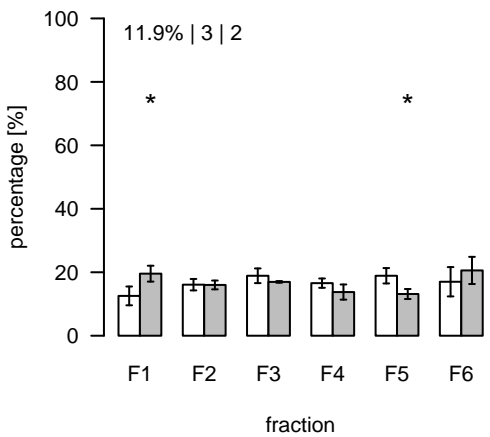
L2281 (m/z=664.441896; rt=11.32785) T/S Cluster: L-11.3-4
