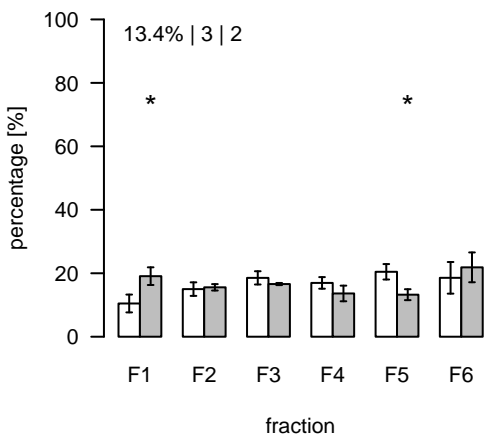
L2272 (m/z=227.1653; rt=11.32776) T/S Cluster: L-11.3-4
