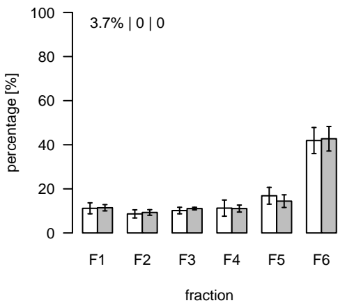
L692 (m/z=1007.594574; rt=5.09929) T/S Cluster: L-5.1-1
