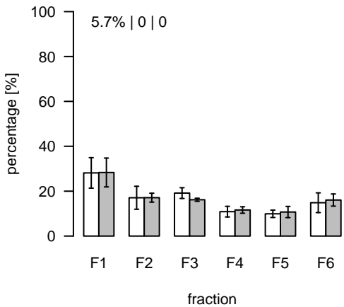
L1991 (m/z=828.659377; rt=10.05891) T/S Cluster: L-10.1-3
