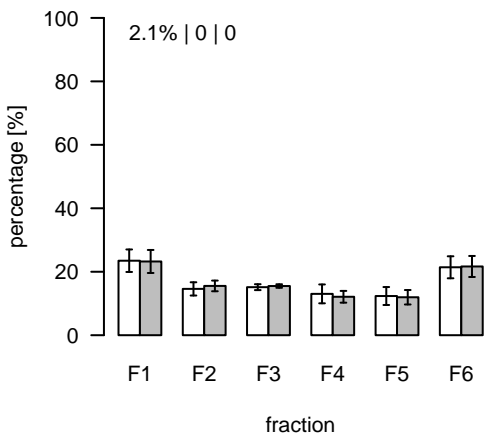
L370 (m/z=803.53172; rt=4.36589) T/S Cluster: L-4.4-1
