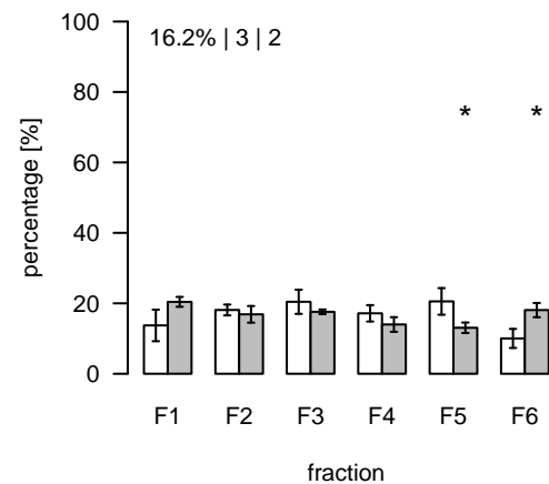
L2293 (m/z=1400.007172; rt=11.32798) T/S Cluster: L-11.3-4
