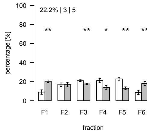
L2378 (m/z=1347.810842; rt=11.32904) T/S Cluster: L-11.3-2
