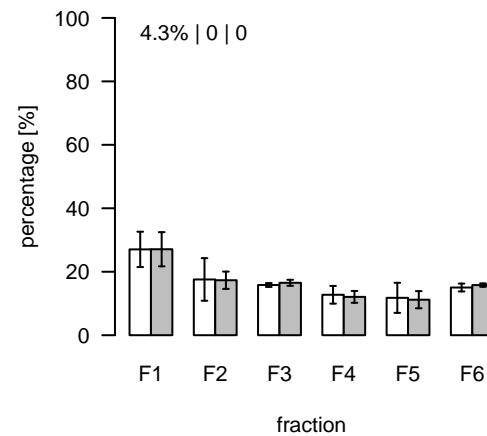
L84 (m/z=681.458616; rt=3.48283) T/S Cluster: L-3.5-6
