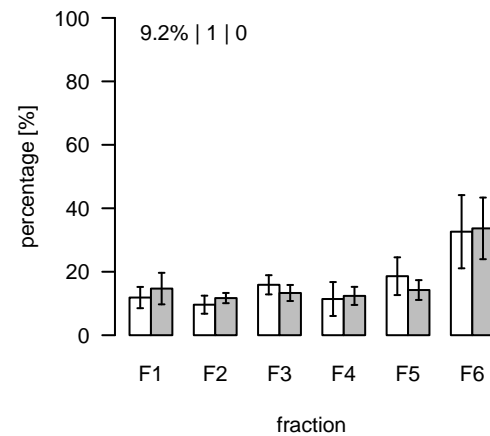
L2022 (m/z=873.559632; rt=10.11943) T/S Cluster: L-10.1-6
