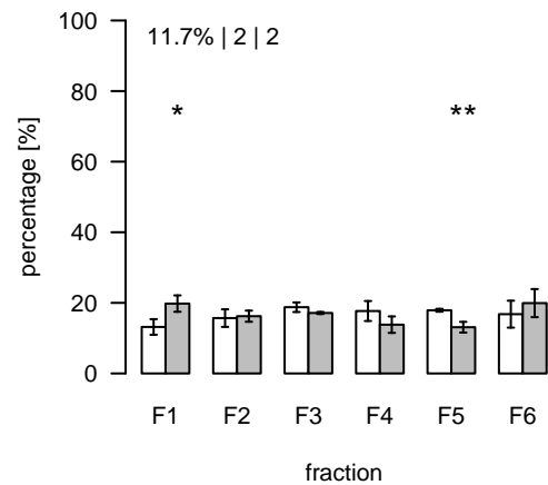
L2248 (m/z=607.394169; rt=11.32731) T/S Cluster: L-11.3-4
