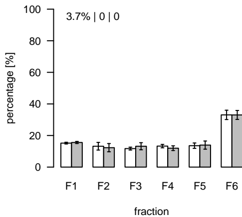
L2451 (m/z=291.20023; rt=11.84631) T/S Cluster: L-11.8-5
