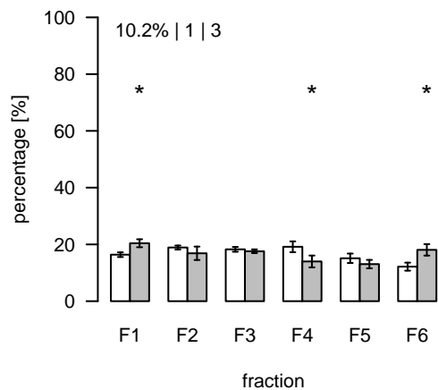
L2088 (m/z=457.766456; rt=10.49974) T/S Cluster: L-10.5-10
