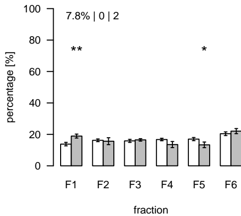
L2376 (m/z=1052.80444; rt=11.32897) T/S Cluster: L-11.3-32
