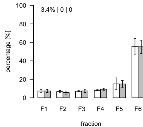
L30 (m/z=813.52333; rt=2.93787) T/S Cluster: L-2.9-1
