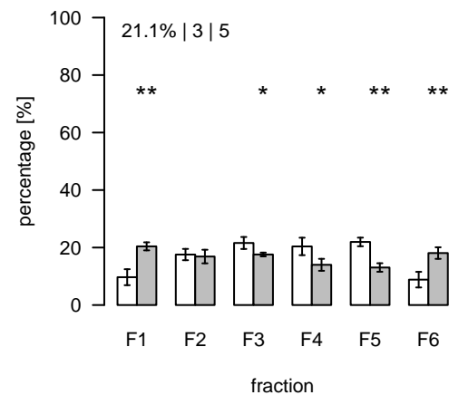
L2231 (m/z=1364.876543; rt=11.30551) T/S Cluster: L-11.3-2
