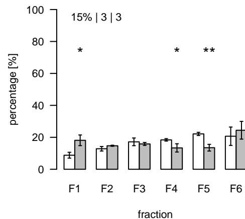
L2358 (m/z=1384.986335; rt=11.32858) T/S Cluster: L-11.3-23
