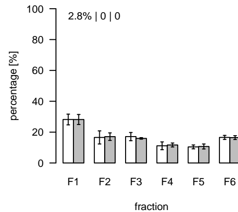
L1268 (m/z=570.511571; rt=7.16476) T/S Cluster: L-7.2-1
