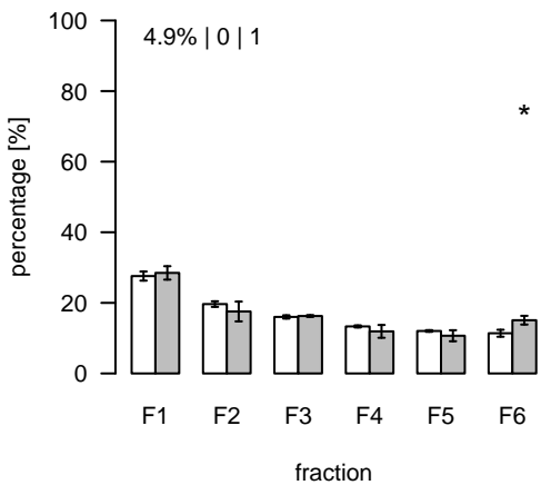
L2258 (m/z=236.50934; rt=11.32756) T/S Cluster: L-11.3-11
