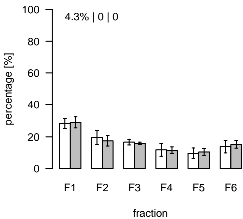
L1370 (m/z=776.56853; rt=7.47593) T/S Cluster: L-7.5-1
