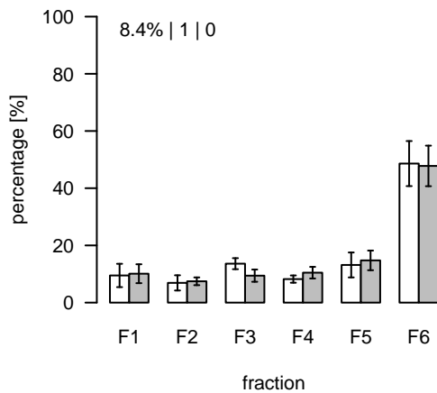
L2015 (m/z=888.574551; rt=10.11546) T/S Cluster: L-10.1-6
