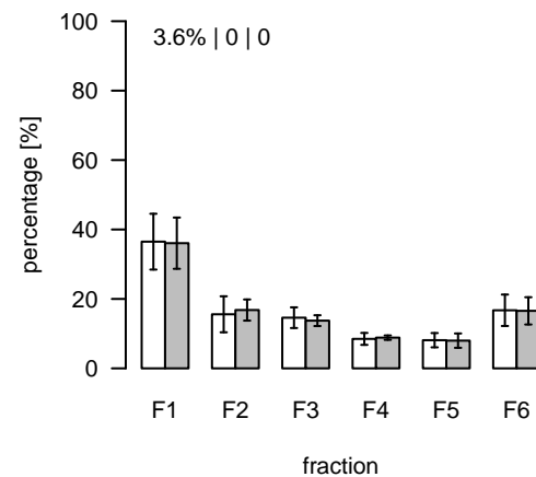
S304 (m/z=570.305658; rt=9.5678) T/S Cluster: S-9.6-1
