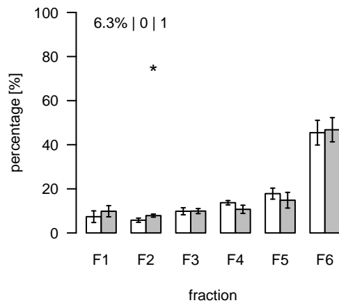
L777 (m/z=811.500492; rt=5.36597) T/S Cluster: L-5.4-2
