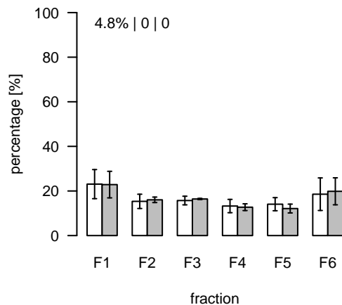
L1309 (m/z=195.142814; rt=7.32632) T/S Cluster: L-7.3-5
