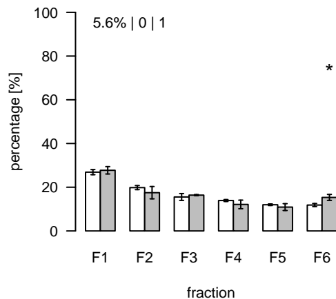
L2278 (m/z=236.17483; rt=11.32781) T/S Cluster: L-11.3-11
