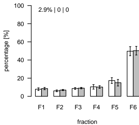
L1648 (m/z=311.551099; rt=8.63872) T/S Cluster: L-8.6-6
