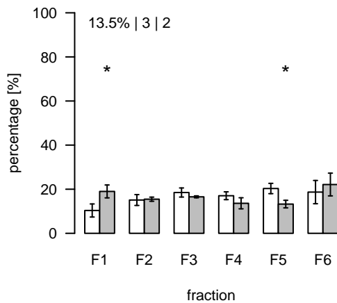
L2285 (m/z=681.454687; rt=11.32788) T/S Cluster: L-11.3-4
