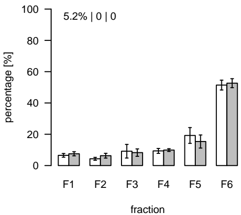
L2037 (m/z=462.766652; rt=10.21265) T/S Cluster: L-10.2-2
