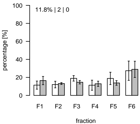
L2005 (m/z=295.190323; rt=10.09039) T/S Cluster: L-10.1-6
