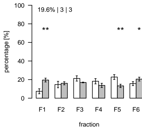
L2338 (m/z=671.974756; rt=11.32842) T/S Cluster: L-11.3-4
