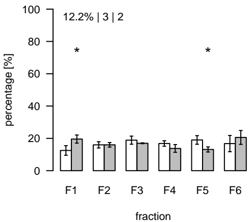
L2254 (m/z=332.233386; rt=11.32752) T/S Cluster: L-11.3-4
