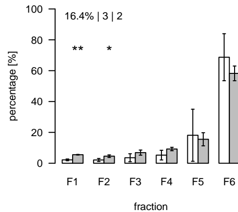
L2009 (m/z=909.541936; rt=10.09429) T/S Cluster: L-10.1-9
