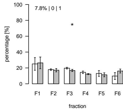
L1542 (m/z=805.559321; rt=8.05647) T/S Cluster: L-8.1-3
