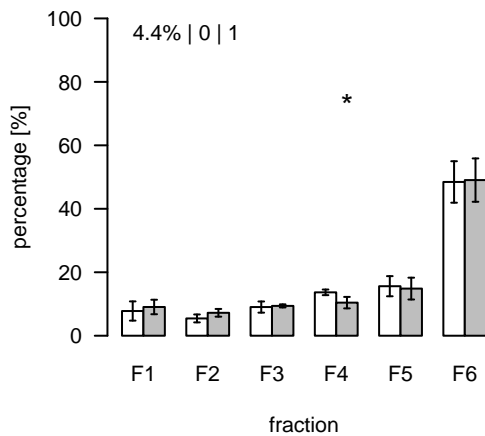
L1349 (m/z=613.468058; rt=7.34797) T/S Cluster: L-7.3-3
