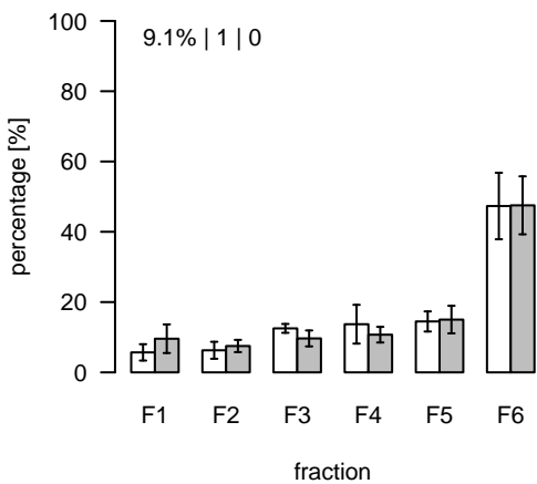
L1871 (m/z=909.531657; rt=9.46389) T/S Cluster: L-9.5-2
