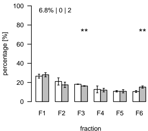
L2134 (m/z=818.666694; rt=10.58444) T/S Cluster: L-10.6-2
