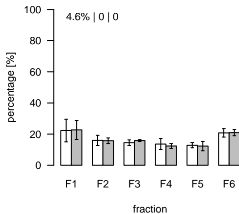
L2222 (m/z=842.649935; rt=11.04041) T/S Cluster: L-11-4
