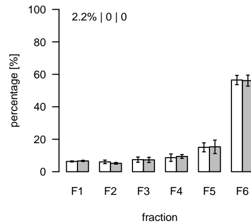
L91 (m/z=984.579967; rt=3.50054) T/S Cluster: L-3.5-1
