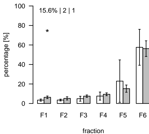
L2011 (m/z=909.486693; rt=10.09542) T/S Cluster: L-10.1-9
