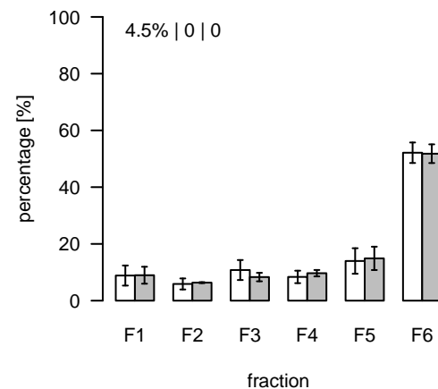
L2224 (m/z=899.552683; rt=11.07588) T/S Cluster: L-11.1-1
