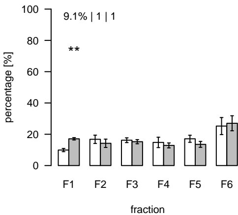
L2771 (m/z=1206.341835; rt=16.96556) T/S Cluster: L-17-2
