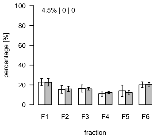
L2396 (m/z=827.683695; rt=11.4115) T/S Cluster: L-11.4-2
