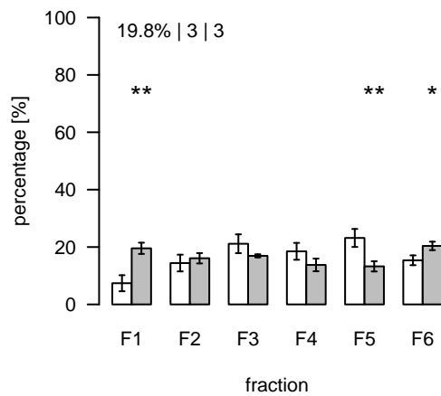
L2309 (m/z=1345.952447; rt=11.32815) T/S Cluster: L-11.3-4
