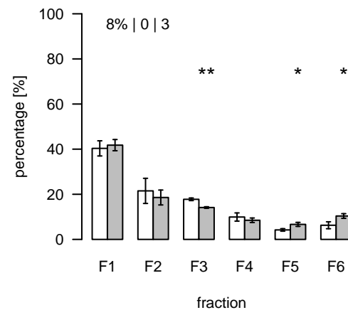
S221 (m/z=290.592957; rt=7.19578) T/S Cluster: S-7.2-2
