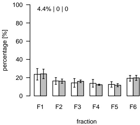
L690 (m/z=830.511992; rt=5.09241) T/S Cluster: L-5.1-5
