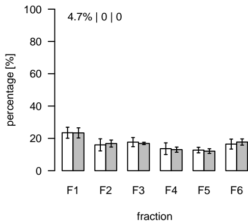
L2170 (m/z=859.701981; rt=10.66193) T/S Cluster: L-10.7-1
