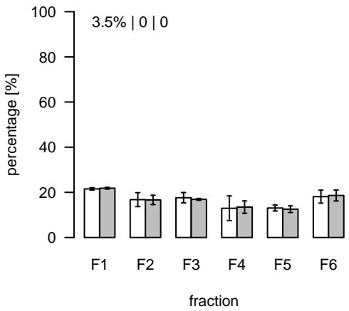
L2150 (m/z=421.845743; rt=10.6126) T/S Cluster: L-10.6-4
