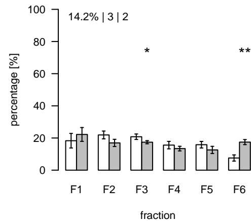
L2302 (m/z=1373.989103; rt=11.32804) T/S Cluster: L-11.3-17
