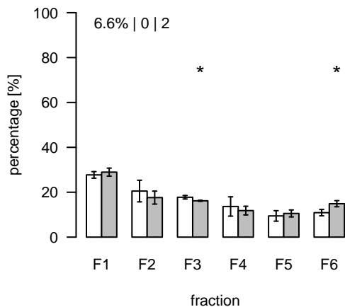
L1916 (m/z=190.147171; rt=9.59703) T/S Cluster: L-9.6-3
