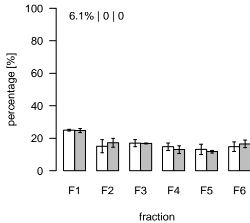
L685 (m/z=804.566647; rt=5.0755) T/S Cluster: L-5.1-3
