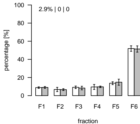
L941 (m/z=389.12999; rt=6.12866) T/S Cluster: L-6.1-1
