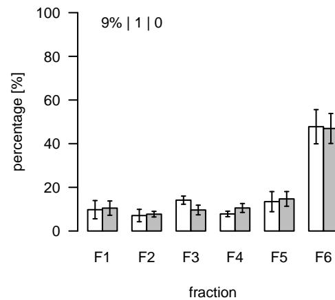
L2014 (m/z=888.553119; rt=10.11389) T/S Cluster: L-10.1-6
