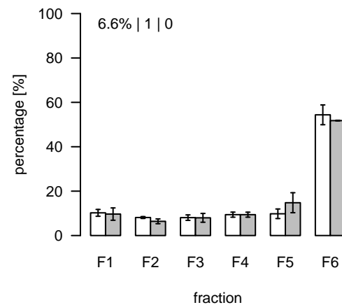
L1599 (m/z=903.568455; rt=8.27632) T/S Cluster: L-8.3-2
