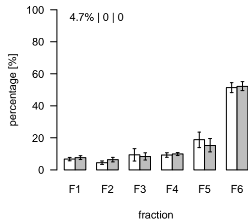
L2031 (m/z=927.542139; rt=10.21243) T/S Cluster: L-10.2-2
