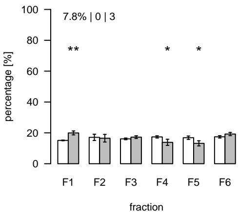
L2239 (m/z=347.250391; rt=11.32183) T/S Cluster: L-11.3-8
