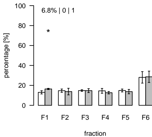
L2090 (m/z=955.610966; rt=10.5041) T/S Cluster: L-10.5-12
