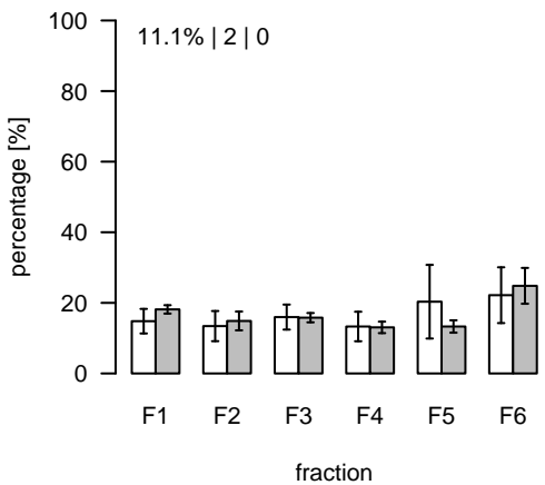
L2007 (m/z=908.543622; rt=10.09159) T/S Cluster: L-10.1-8
