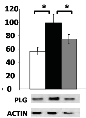
J PLASMINOGEN
