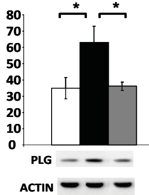
E PLASMINOGEN
