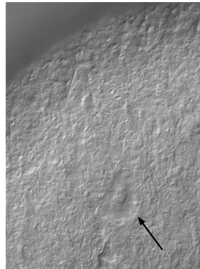
otxA RNAi
