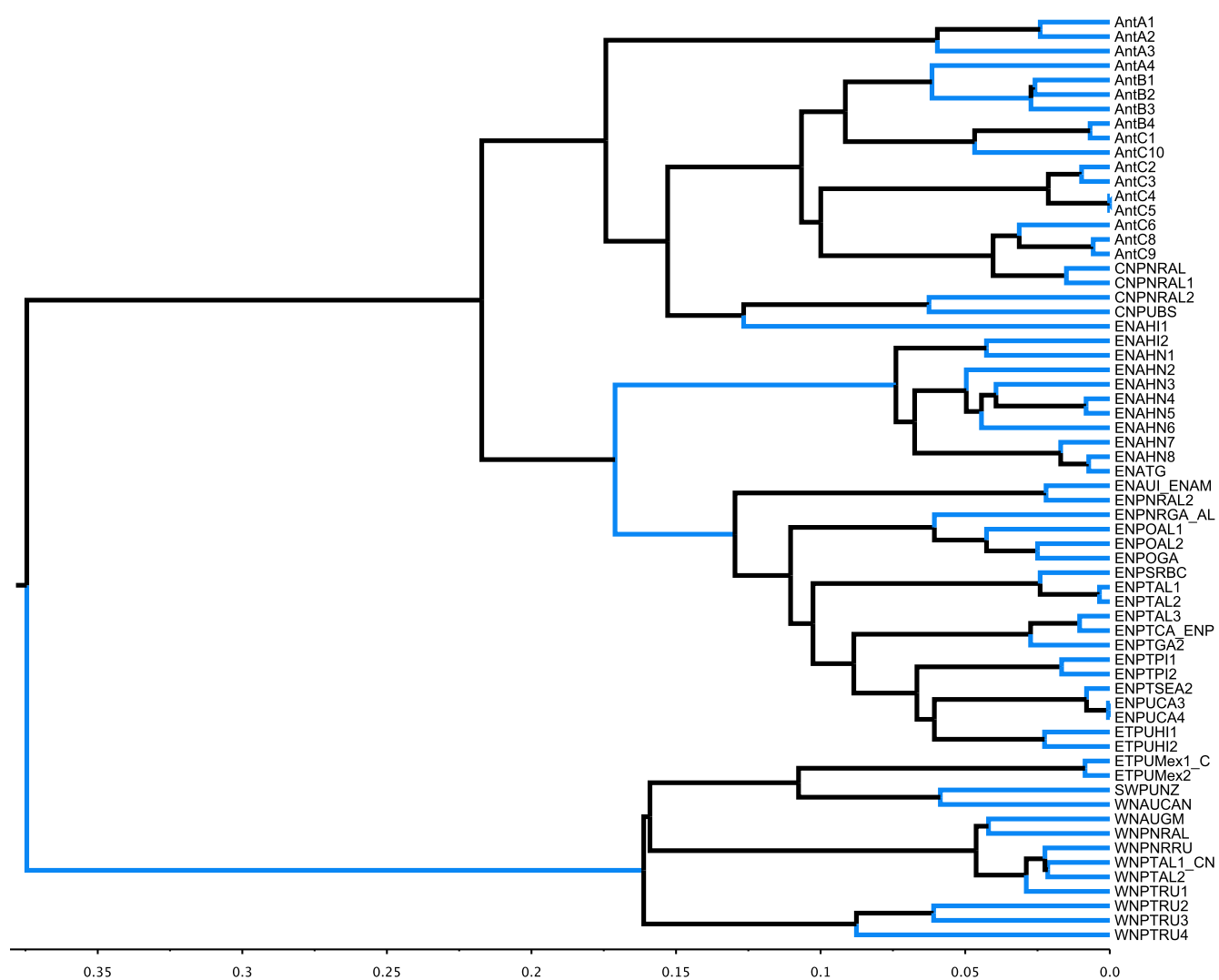
COX3
