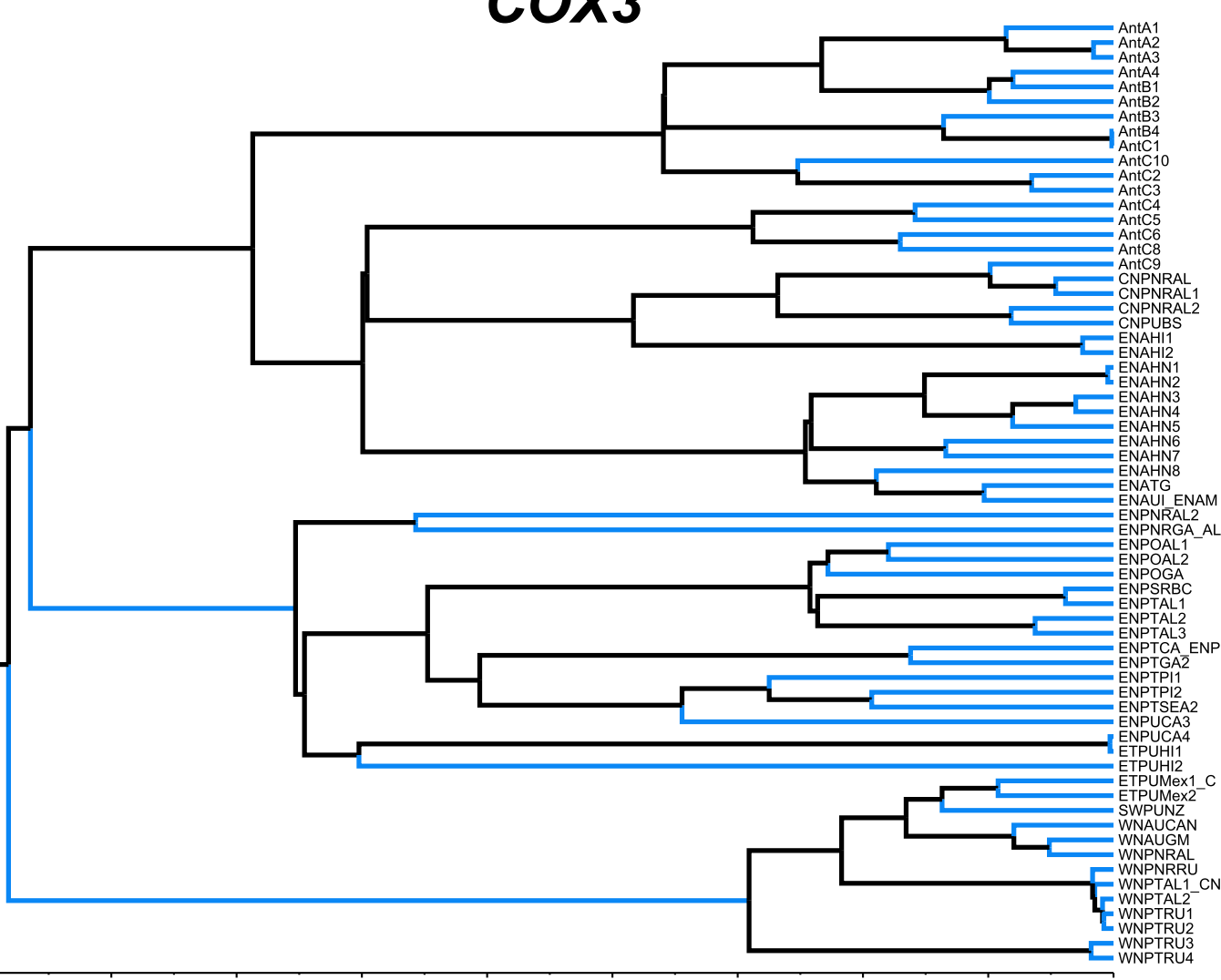
ND4L
