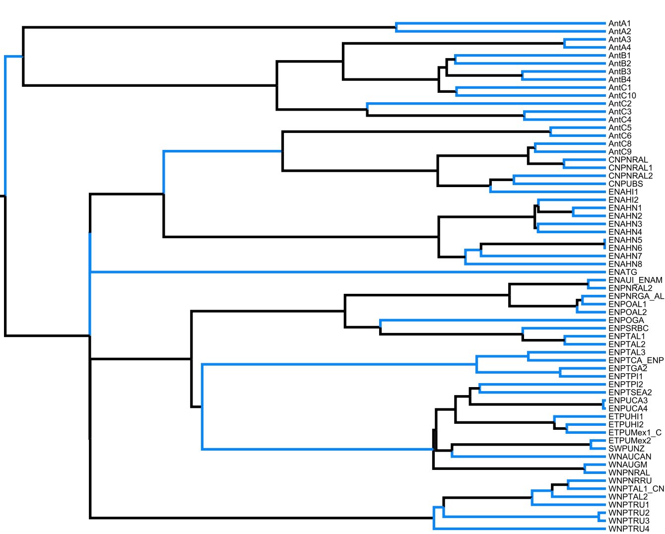
ND5
