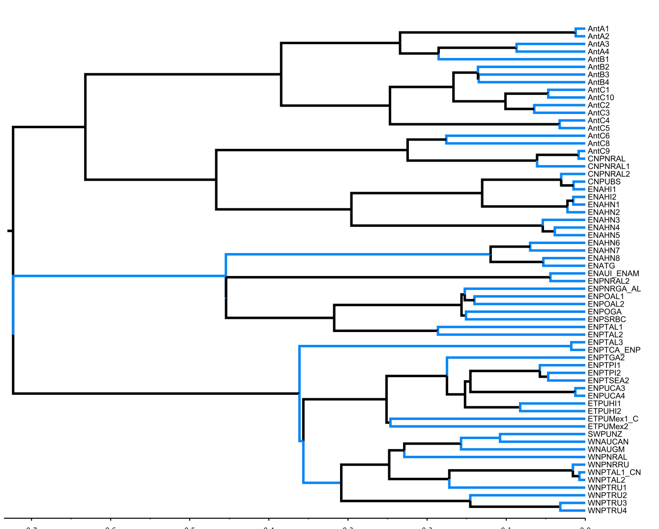
ND3
