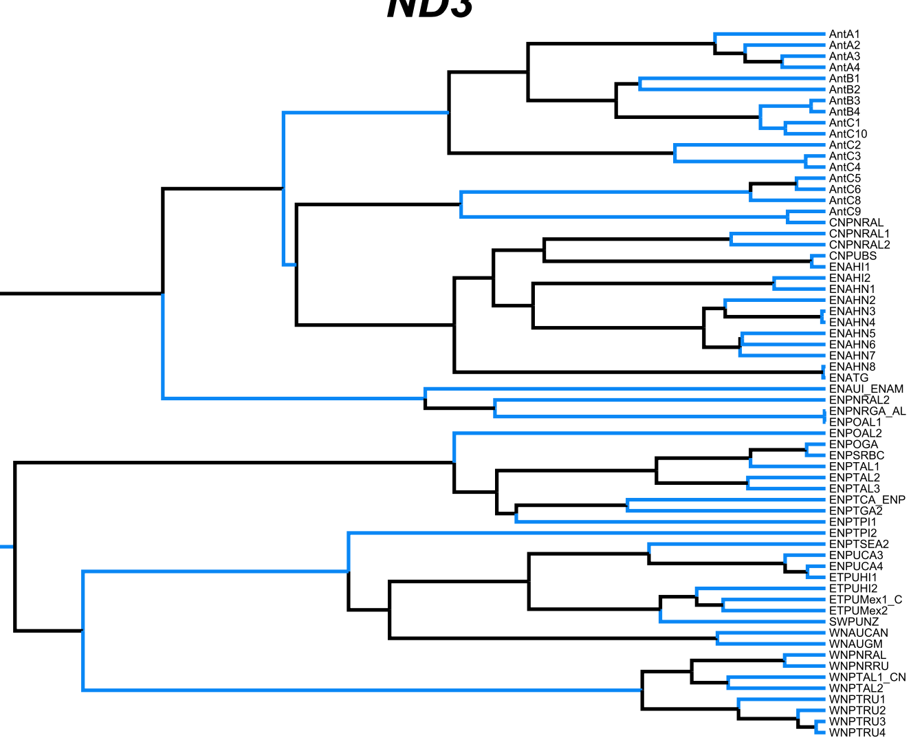
ND4
