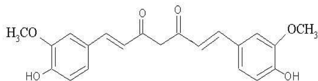
Curcumin
