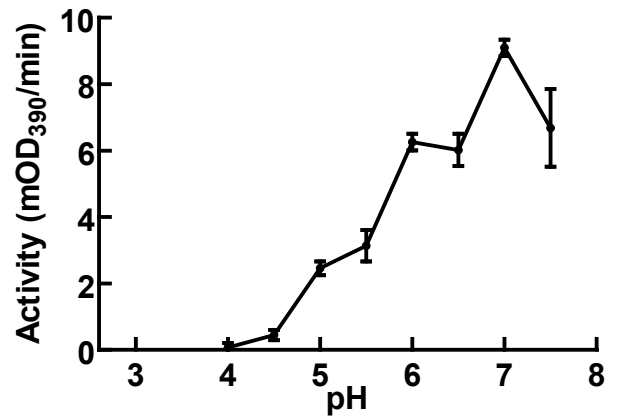
NBAD
