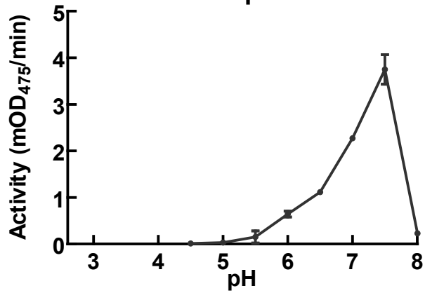
Dopa
