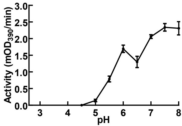
NADA
