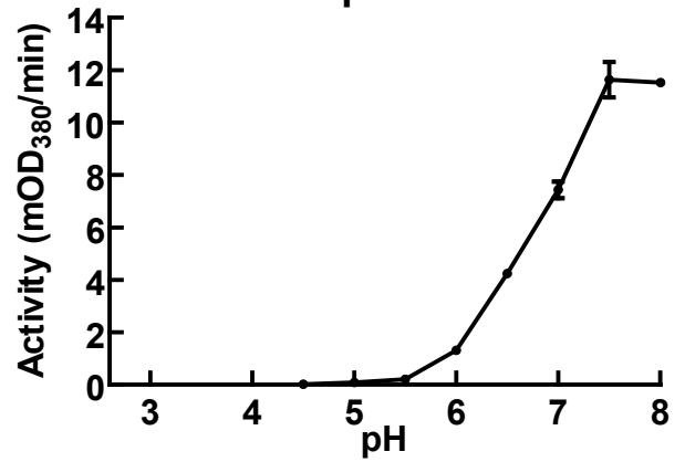
Dopamine
