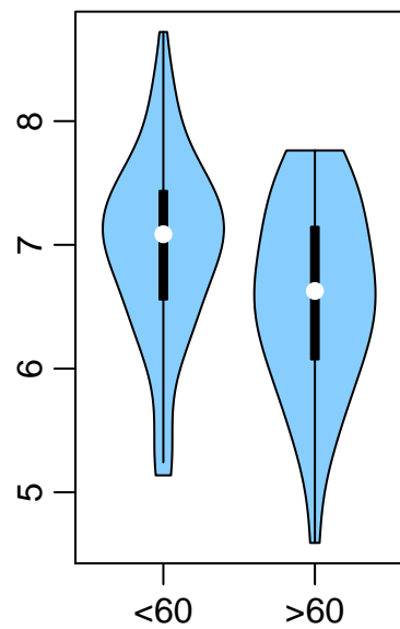
miR-340-3p
