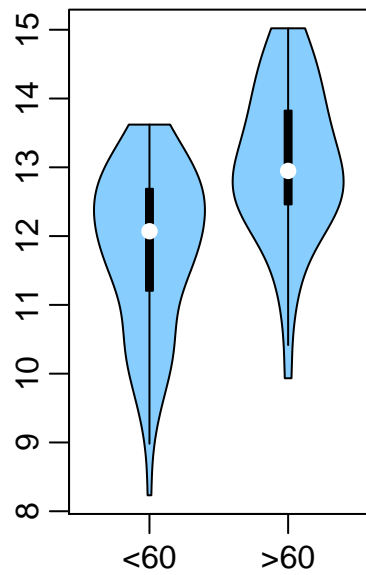
miR-146b-5p
