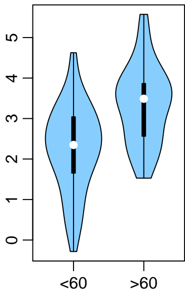
miR-146b-3p
