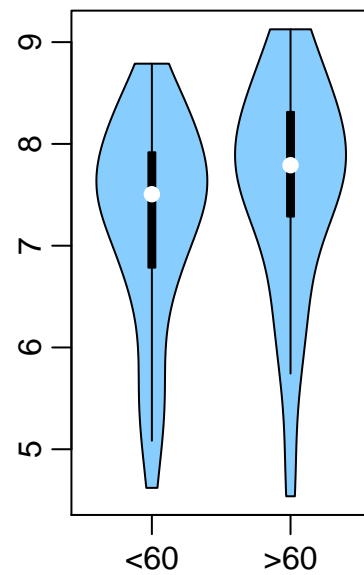
miR-218-5p
