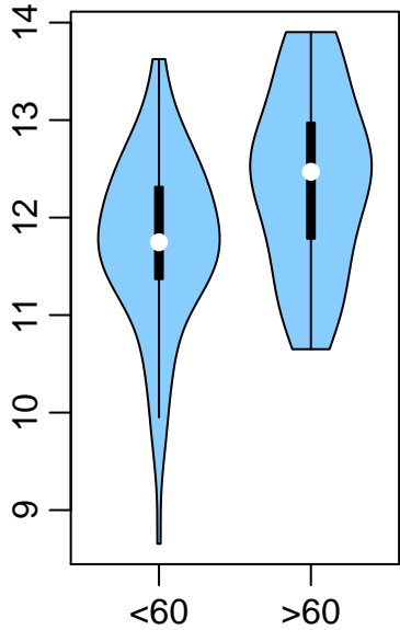
miR-146a-5p
