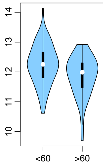
miR-193a-5p
