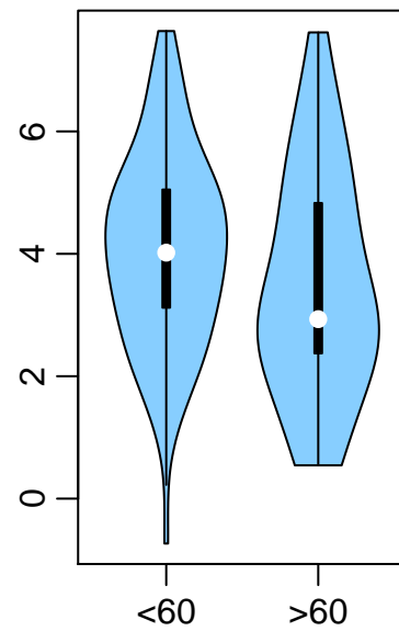
miR-1179
