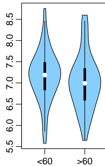
miR-29b-2-5p
