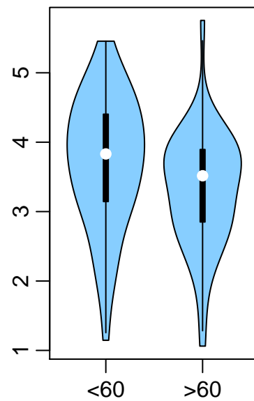
miR-4421
