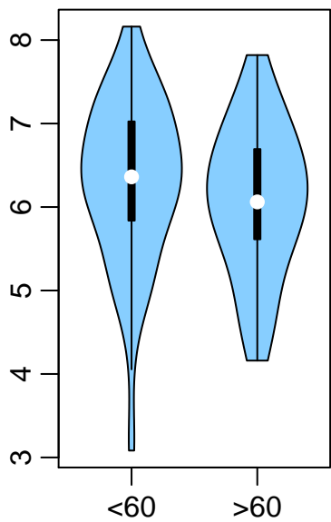
miR-598
