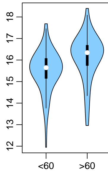
miR-21-5p
