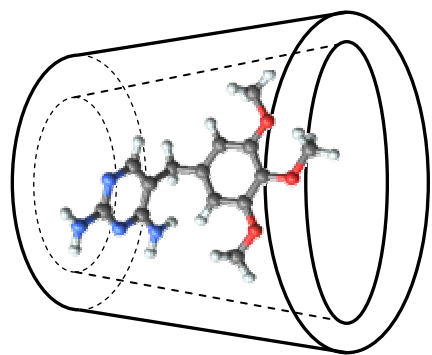
TMP/ \gamma -CD
