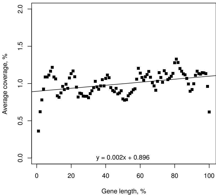
RNA-seq, Illumina
