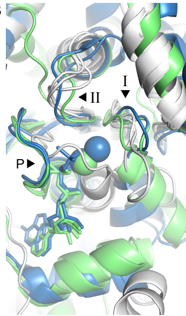
ParA
