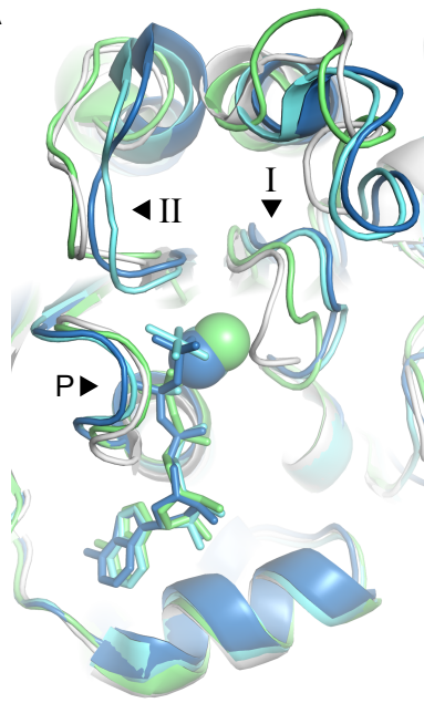
NifH
