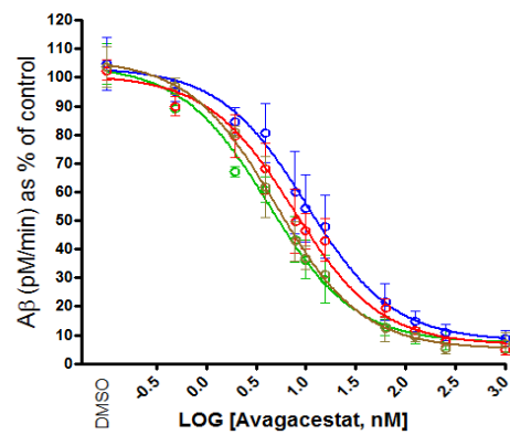
Avagacestat
