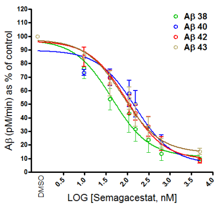
Semagacestat
