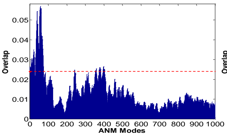
Enolase
