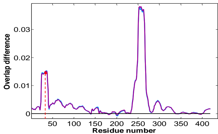
Enolase
