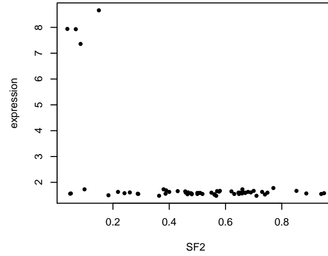
PTPRCAP : Corr = -0.486
