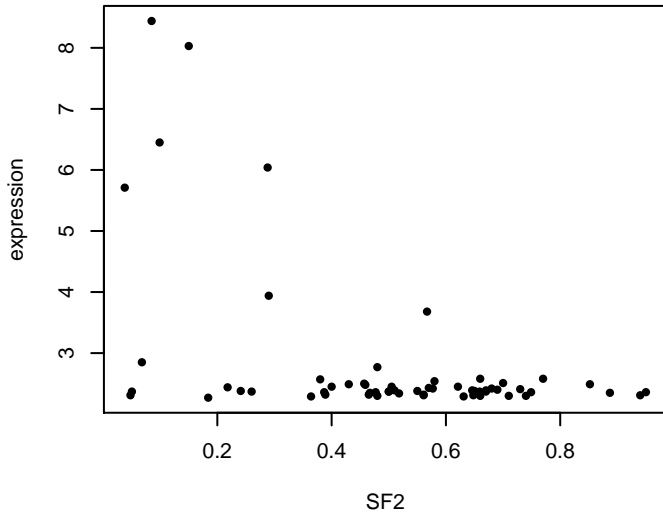
LAPTM5 : Corr = -0.498
