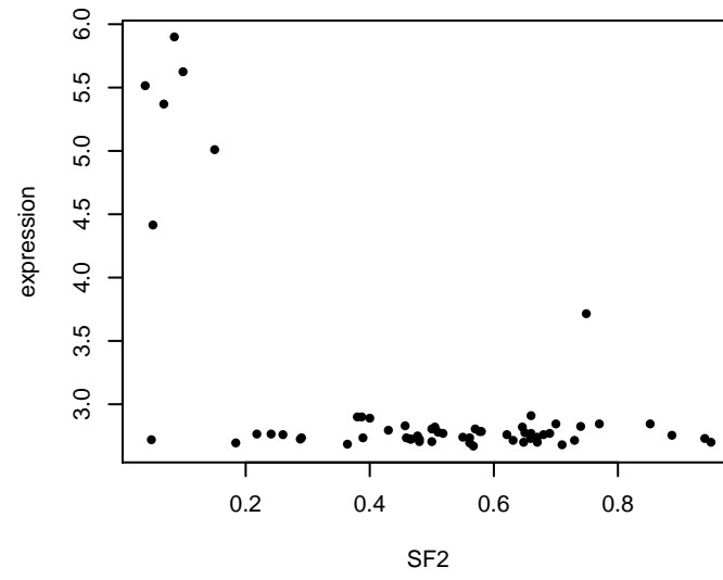
HCLS1 : Corr = -0.576
