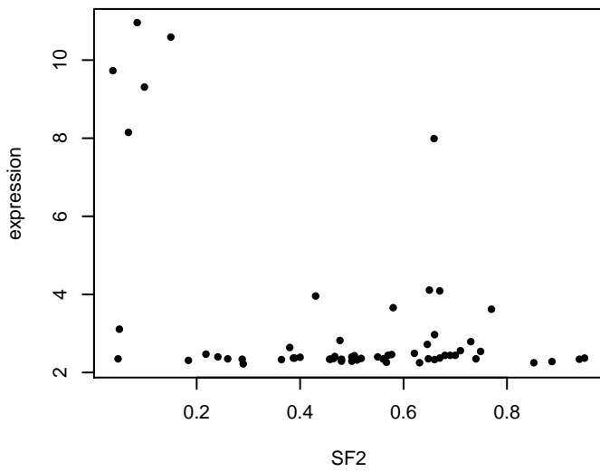
CORO1A : Corr = -0.464
