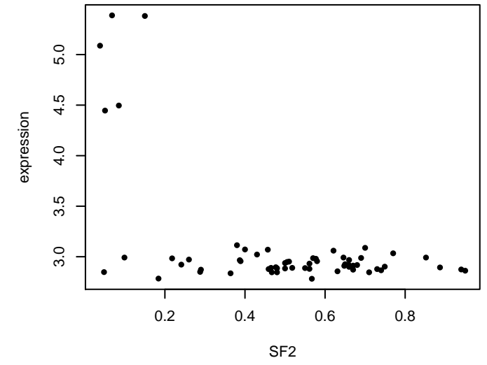
PTPRC : Corr = -0.543
