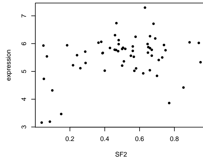
ANXA2 : Corr = 0.339
