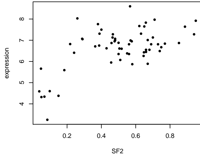
DAG1 : Corr = 0.603
