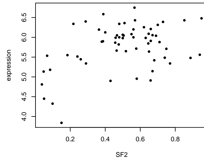
ANXA5 : Corr = 0.422
