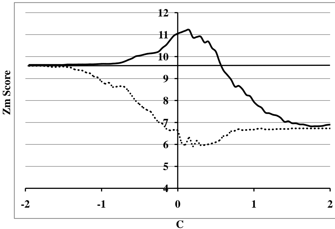
Figure2 Comparison of Zm-o, Zm-p, Zm-q values of HIF1(Zm-o horizontal line, Zm-p solid line, Zm-q dashed line)
