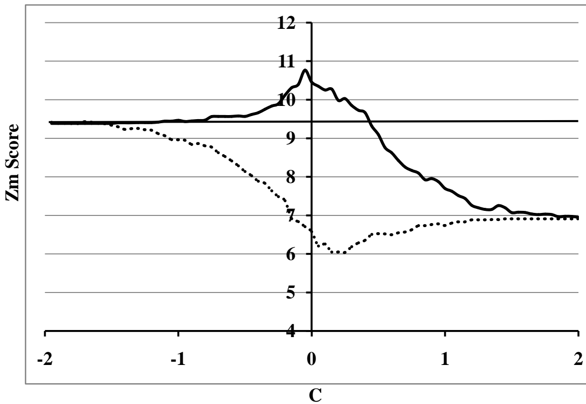
Figure4 Comparison of Zm-o, Zm-p, Zm-q values of AhR(Zm-o horizontal line, Zm-p solid line, Zm-q dashed line)
