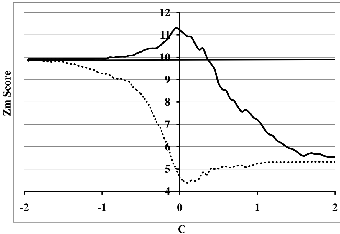
Figure1 Comparison of Zm-o, Zm-p, Zm-q values of Sp1(Zm-o horizontal line, Zm-p solid line, Zm-q dashed line)
