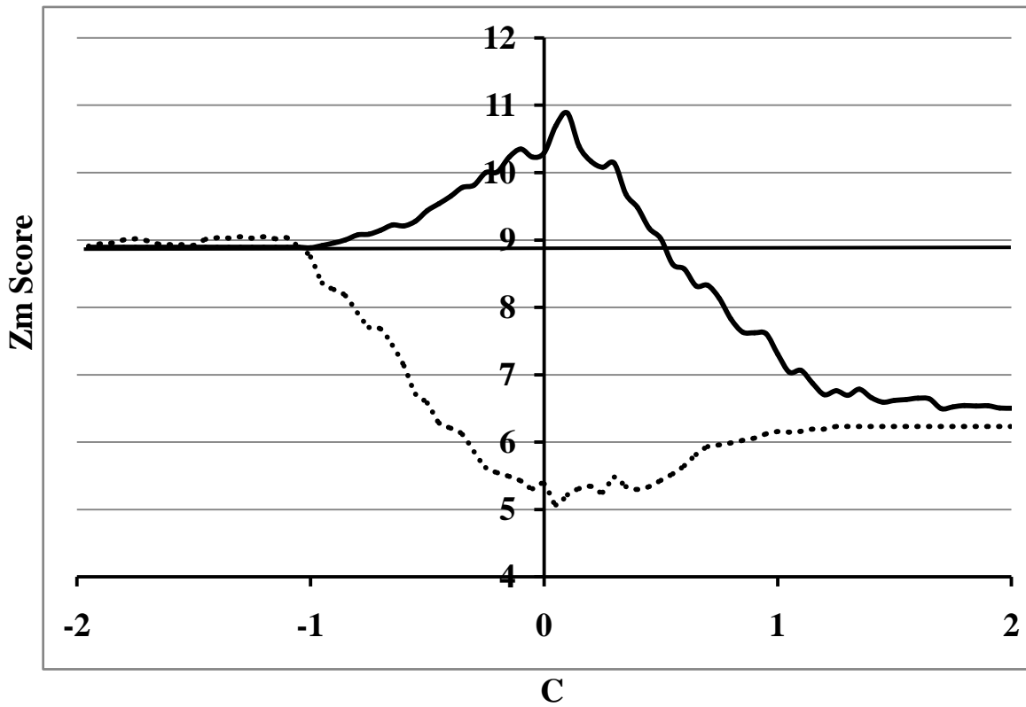
Figure3 Comparison of Zm-o, Zm-p, Zm-q values of Whn(Zm-o horizontal line, Zm-p solid line, Zm-q dashed line)
