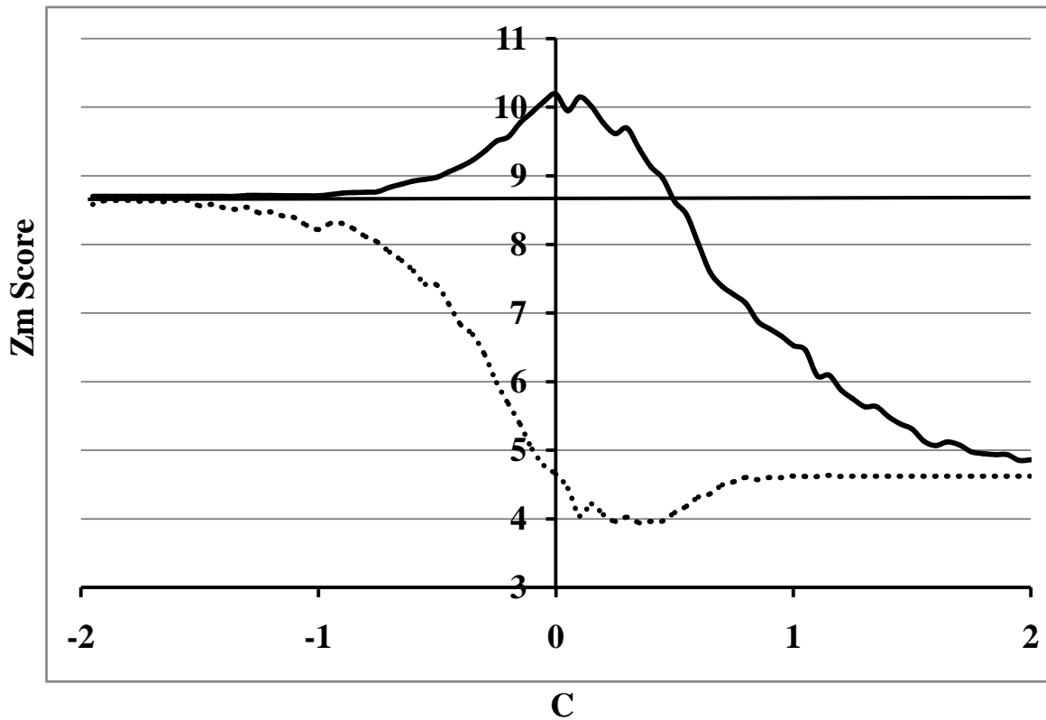
Figure7 Comparison of Zm-o, Zm-p, Zm-q values of KROX(Zm-o horizontal line, Zm-p solid line, Zm-q dashed line)
