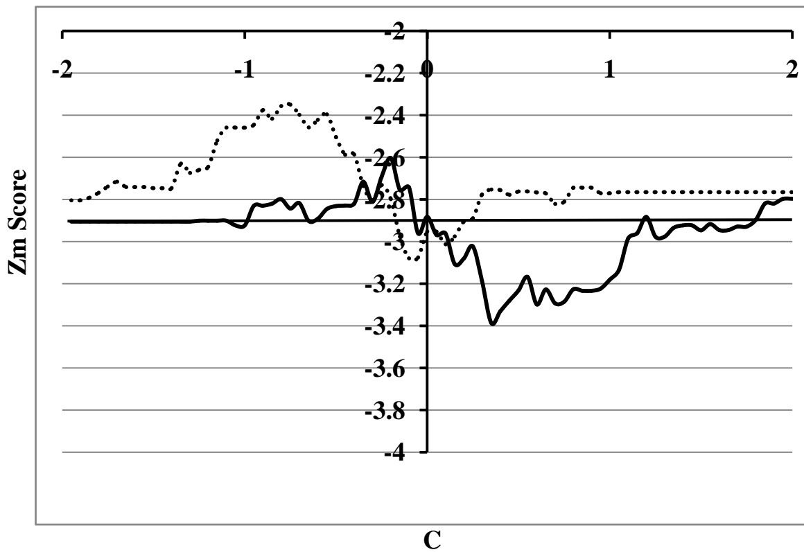
Figure8 Comparison of Zm-o, Zm-p, Zm-q values of GCNF(Zm-o horizontal line, Zm-p solid line, Zm-q dashed line)
