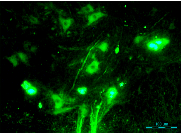
YFP
