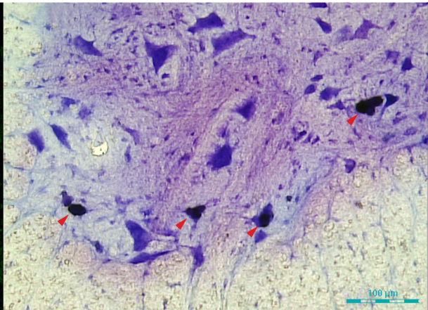
Azure B
