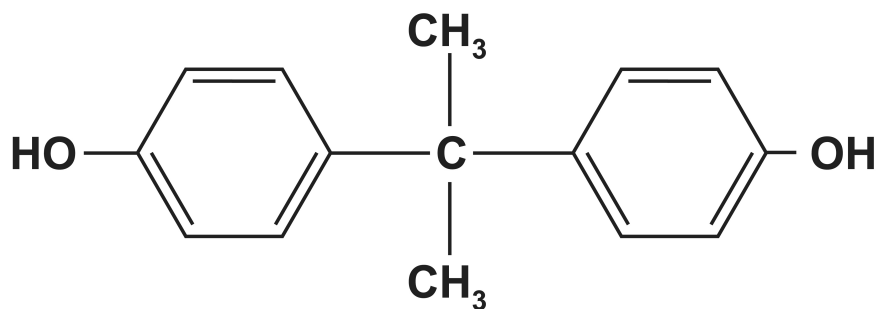
Bisphenol A
