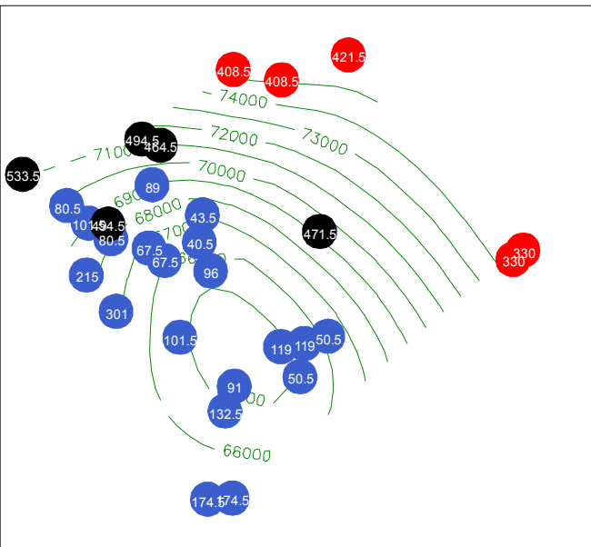
Calcium
