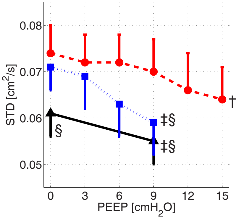
MRI ADC
