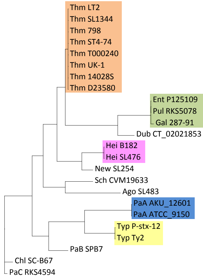
6-locus MLST
