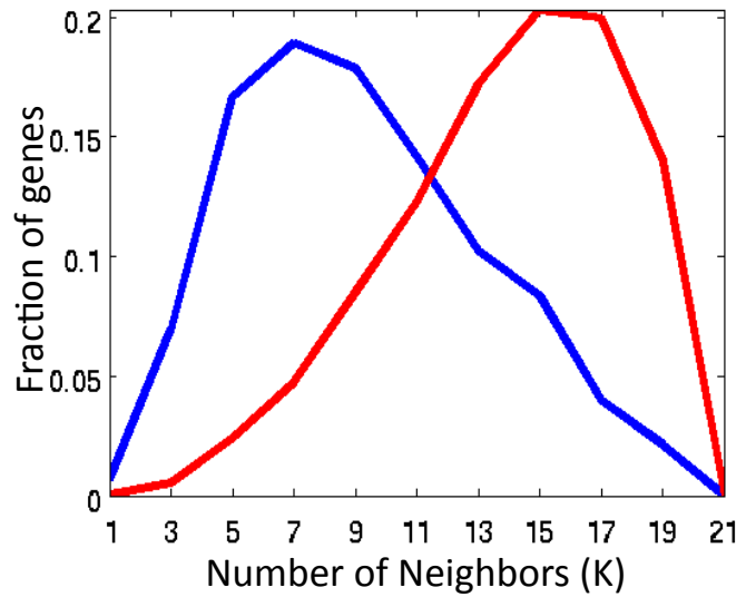
Intra-Pop (CEU) P < 10^{-274}
