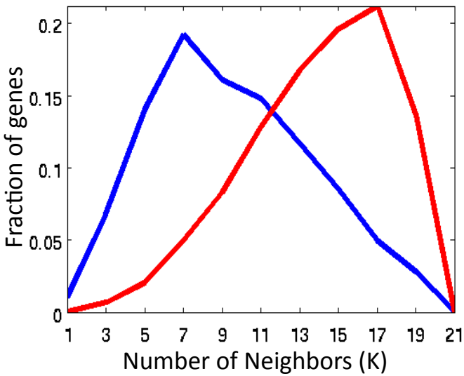
Intra-Pop (YRI) P < 10^{-225}
