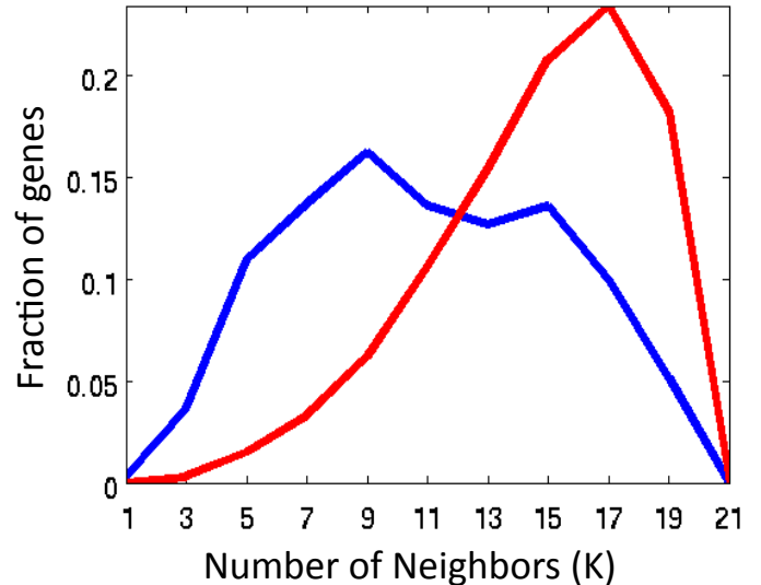
Intra-Pop (CEU) P < 10^{-274}
