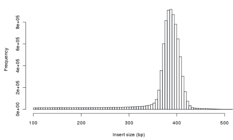
7BL PE insert size distribution
