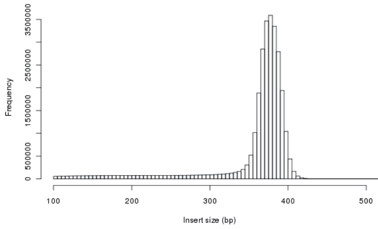
7BS PE insert size distribution
