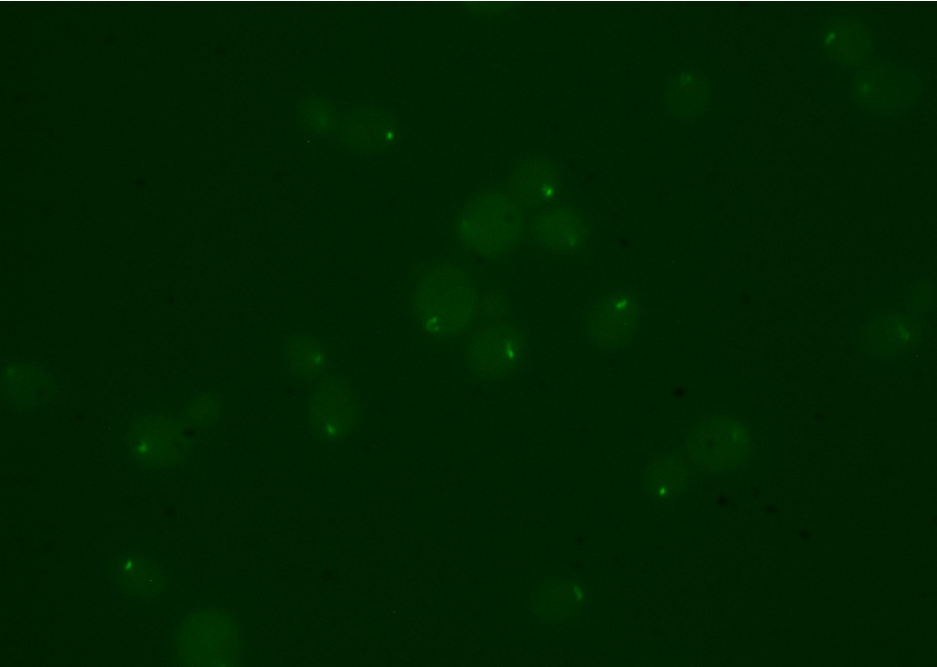
S6B. Rrn11-GFP in yna30Δ
