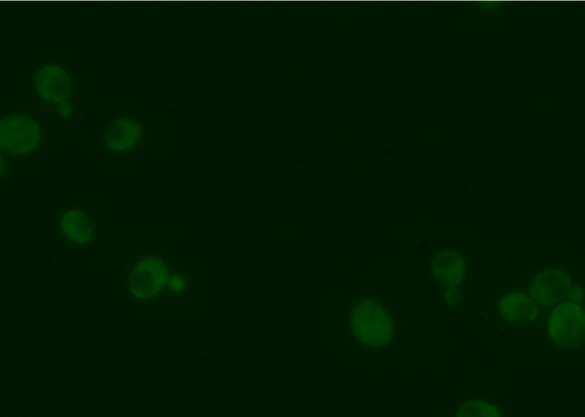
S10B. Glr1-GFP in yna30Δ
