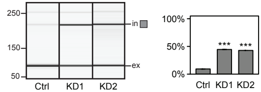
TNPO3
