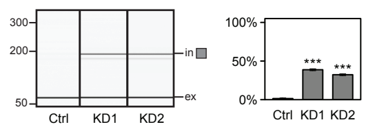
VHL
