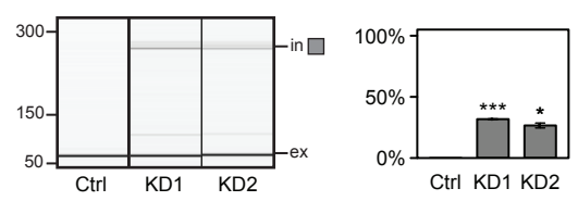
TOR1AIP1
