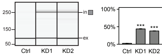
SF3B3
