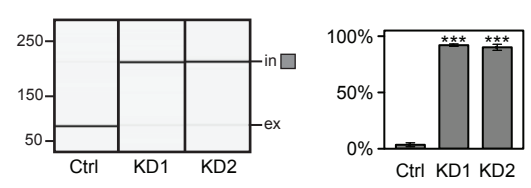
WRN
