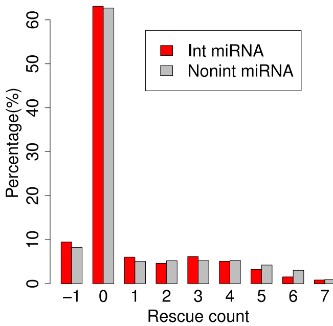
A. Human
