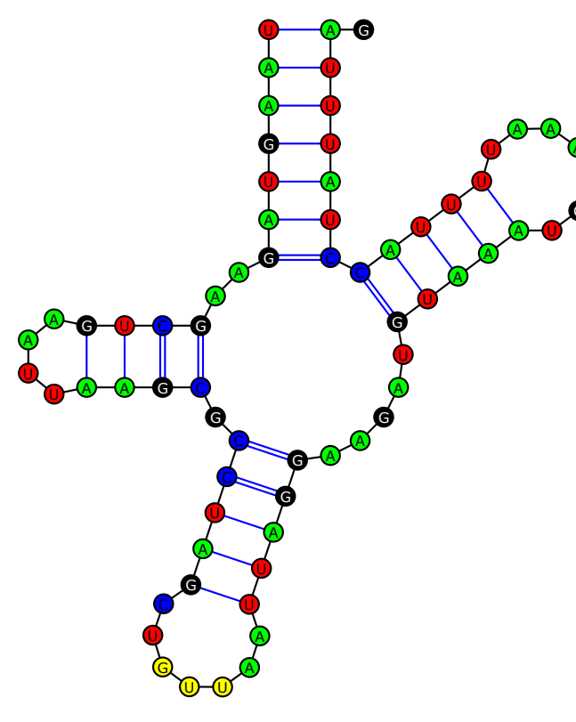
tRNA-Asn(GUU)
