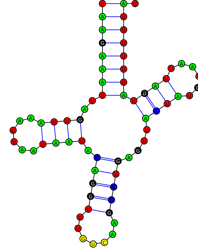
tRNA-Asp(GUC)
