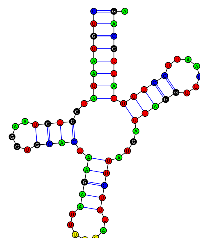
tRNA-Gln(UUG)
