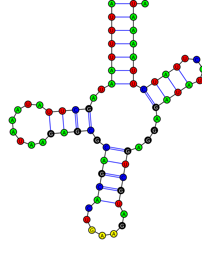
tRNA-Phe(GAA)
