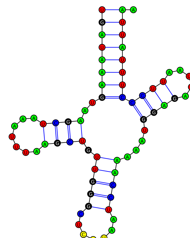
tRNA-Met(CAU)
