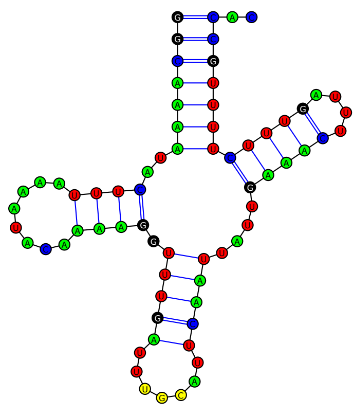
tRNA-Ala(UGC)
