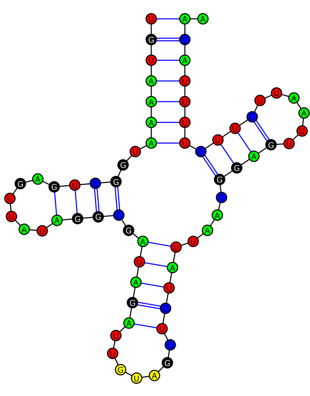
tRNA-Tyr(GUA)
