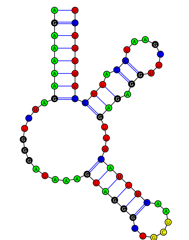
tRNA-Ser1(GCU)
