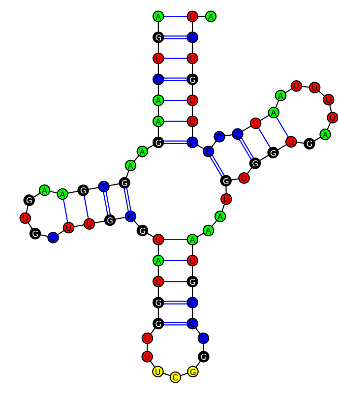
tRNA-Arg(UCG)
