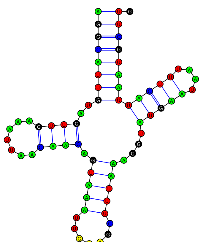
tRNA-Cys(GCA)
