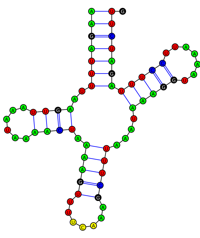
tRNA-Trp(UCA)
