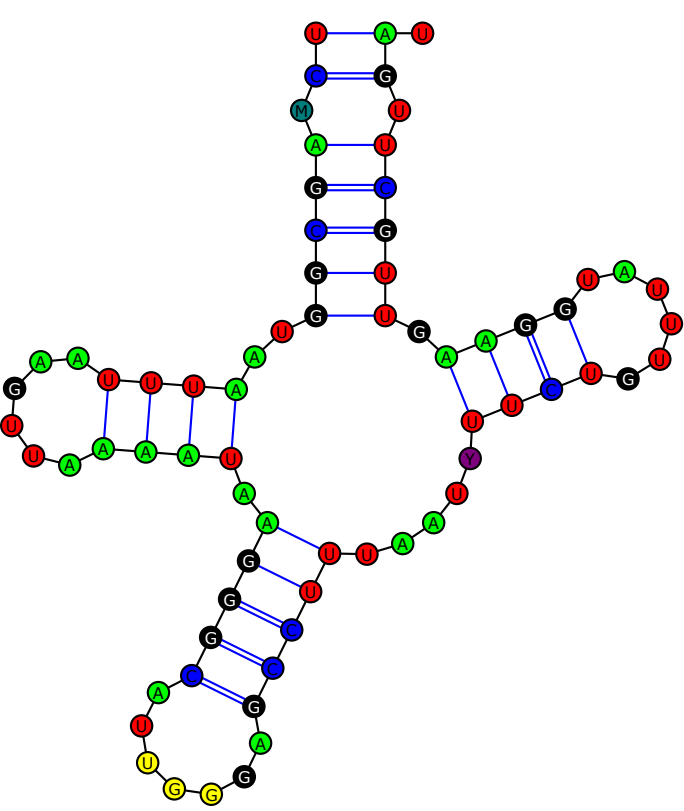
tRNA-Pro(UGG)
