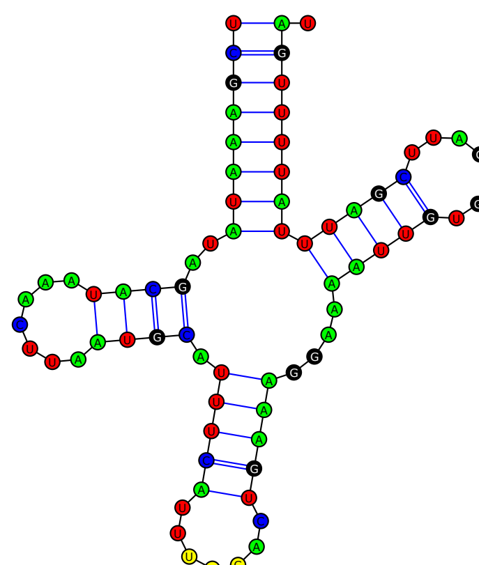
tRNA-Val(UAC)
