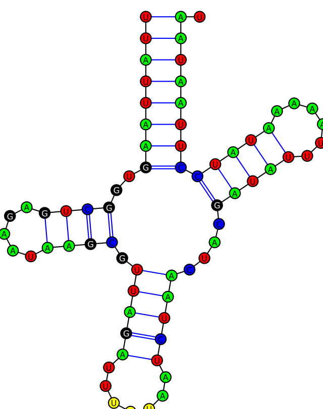
tRNA-Lys(UUU)
