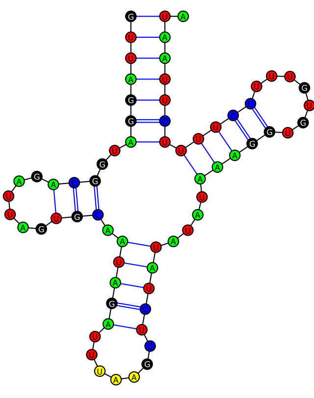
tRNA-Leu2(UAA)
