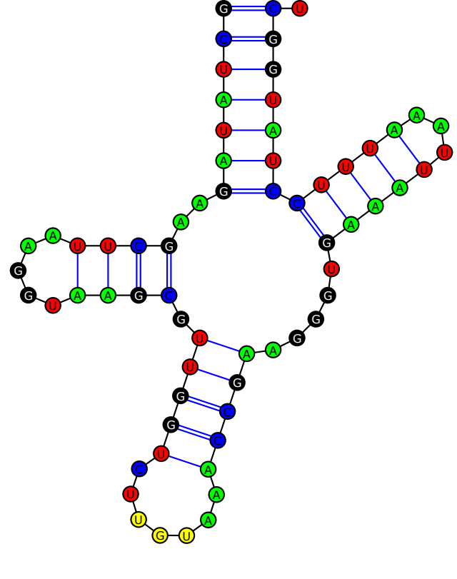
tRNA-Thr(UGU)
