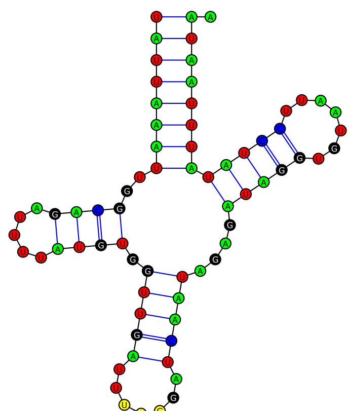
tRNA-Leu1(UAG)
