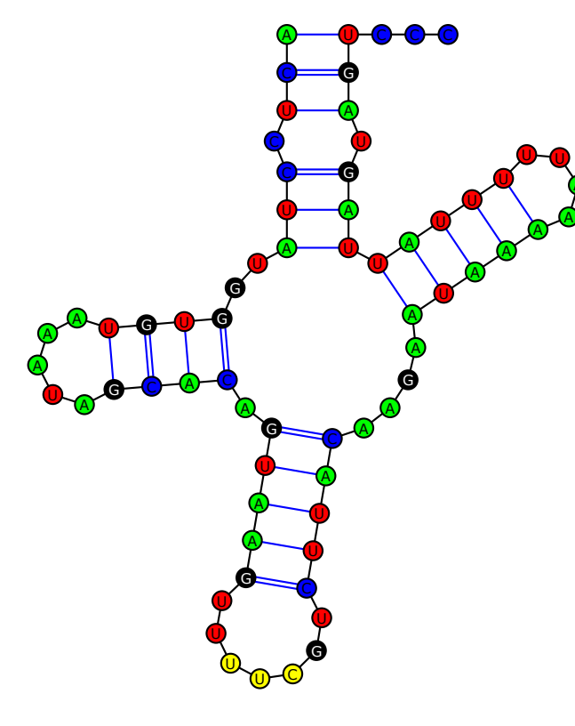
tRNA-Glu(UUC)
