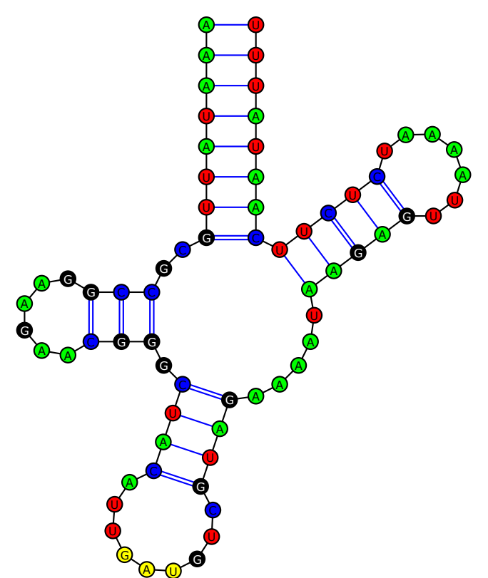
tRNA-Ile(GAU)
